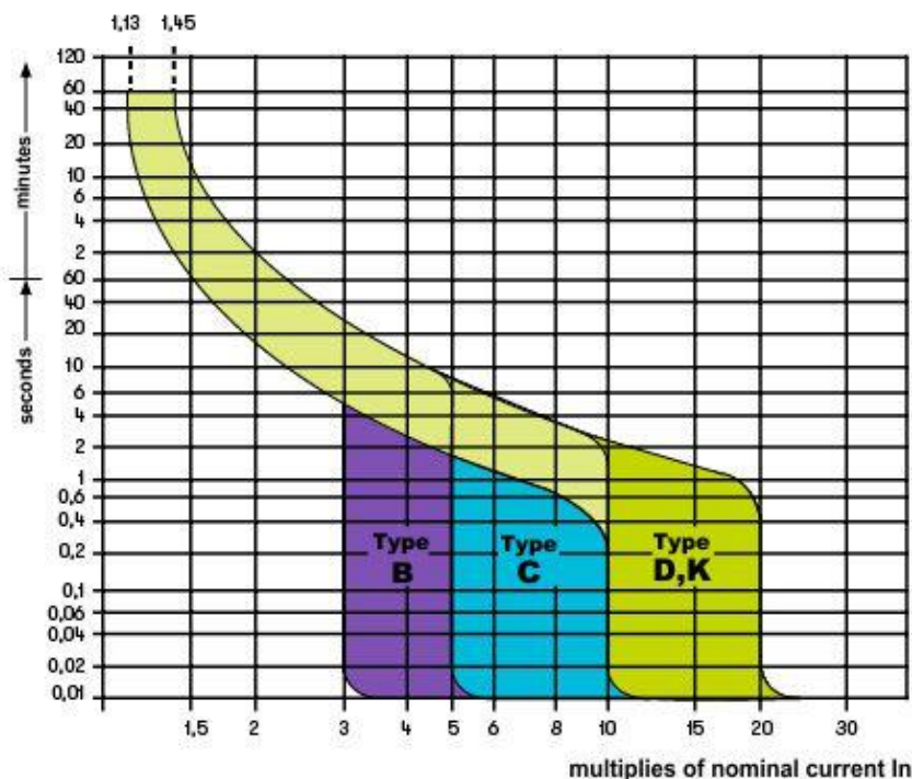
Fig. 52: Ejemplo de curvas de intervención de protección magnetotérmica (MCB)
