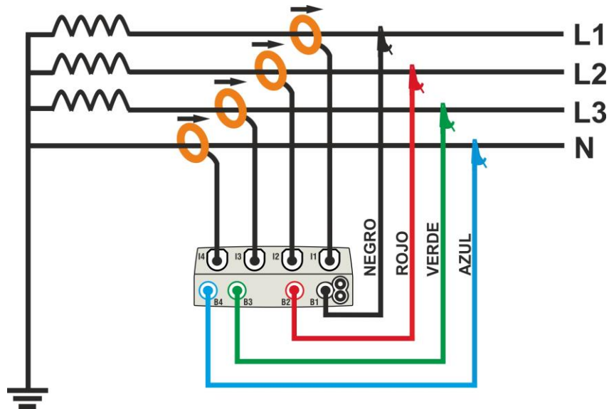
Fig. 37: Conexión para medida en sistema Trifásico 3 \phi -4HILOS
