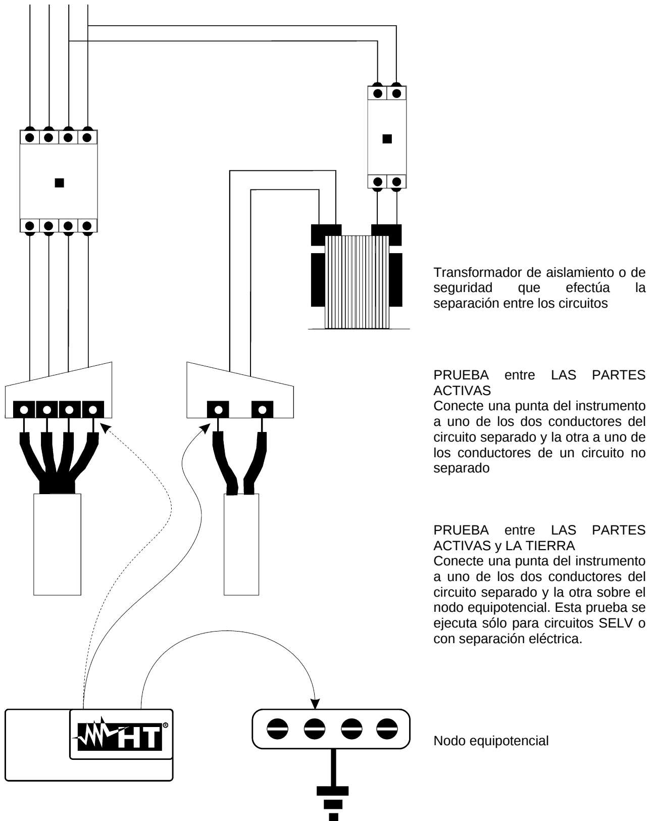
Fig. 51: medidas de separación entre circuitos en una instalación
