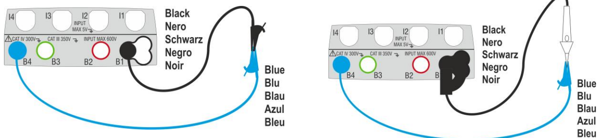
Fig. 7: Compensación de la resistencia de los cables y de la punta remota
