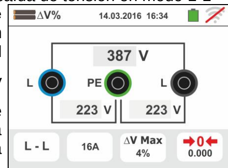
Fig. 35: Conexión del instrumento para la medida de la caída de tensión en modo L-L
