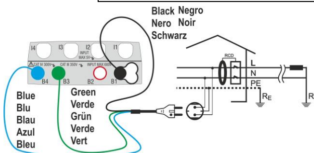
Fig. 10: Conexión en sistema monofásico mediante la toma shuko
