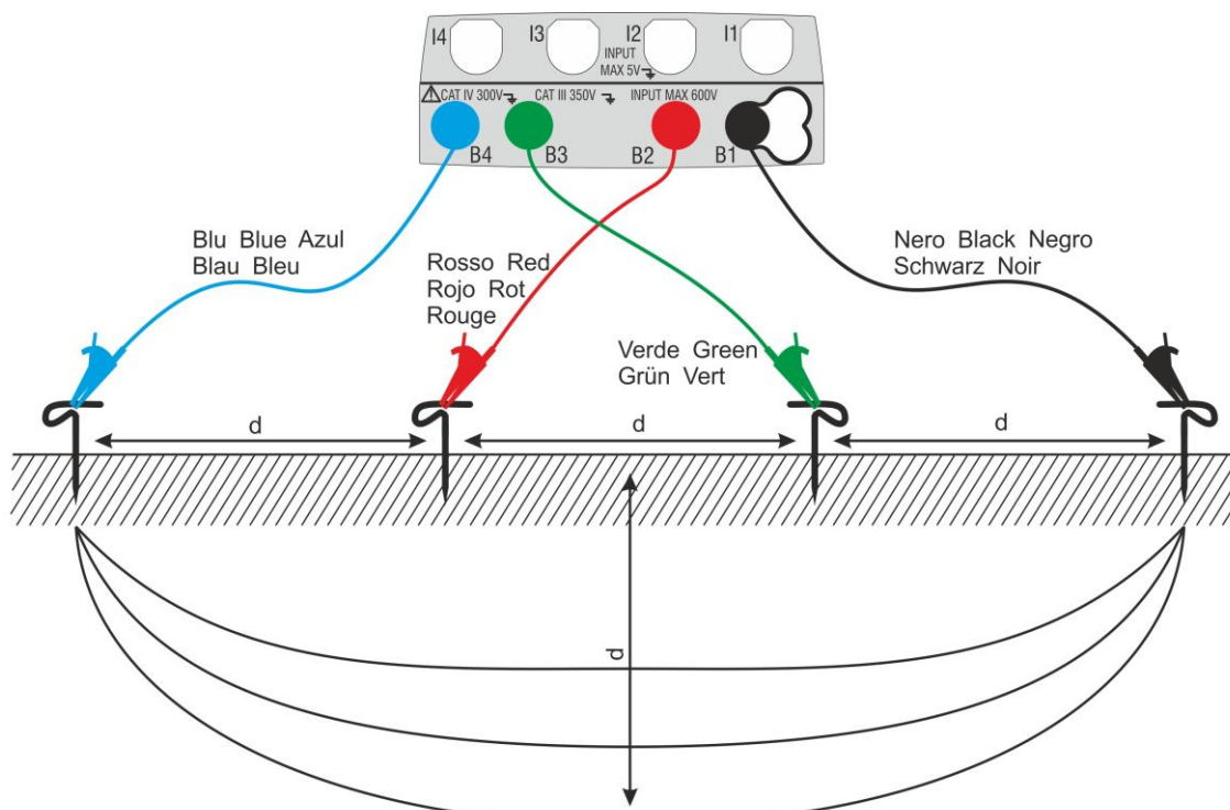
Fig. 30: Medida de la resistividad del terreno
