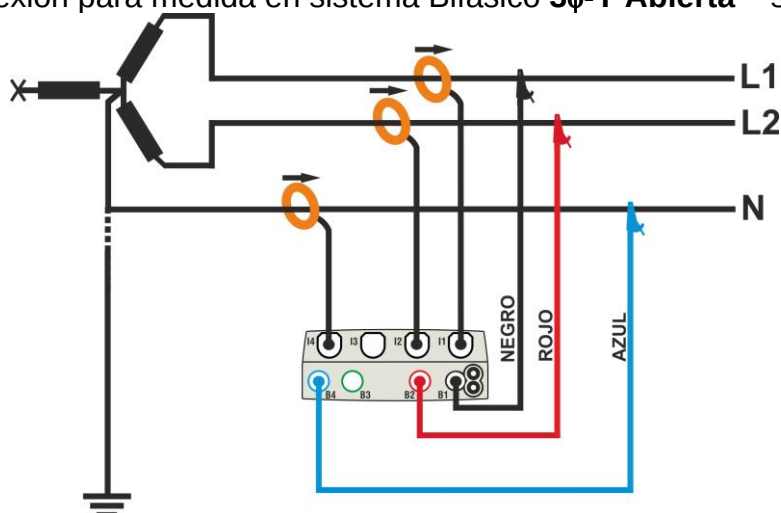
Fig. 43: Conexión para medida en sistema Bifásico 3φ-2EI. 1/2 – sistemas USA
