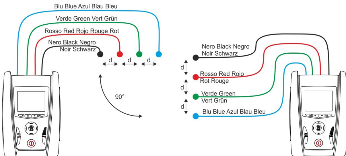
Fig. 55: Medida de la resistividad del terreno
