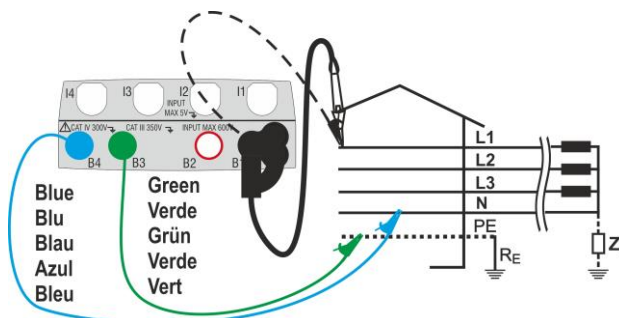
Fig. 22: Medida L-PE en sistemas IT con cables y punta remota
