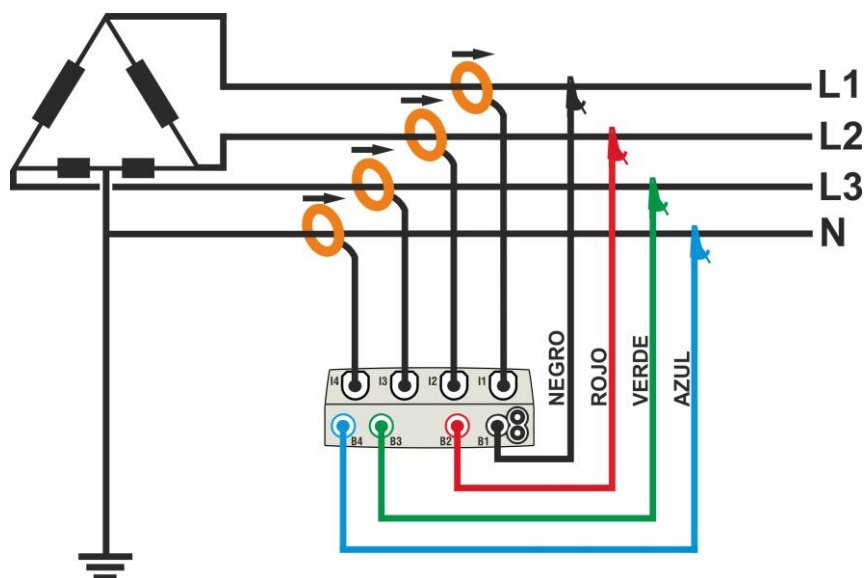
Fig. 40: Conexión para medida en sistema Trifásico 3φ-High Leg – sistemas USA
