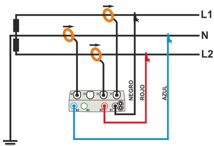
Fig. 44: Conexión para medida en sistema Bifásico 1φ-TomaCentral – sistemas USA
