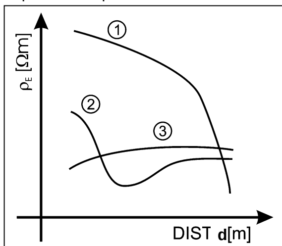
Fig. 56: Medida de la resistividad del terreno
