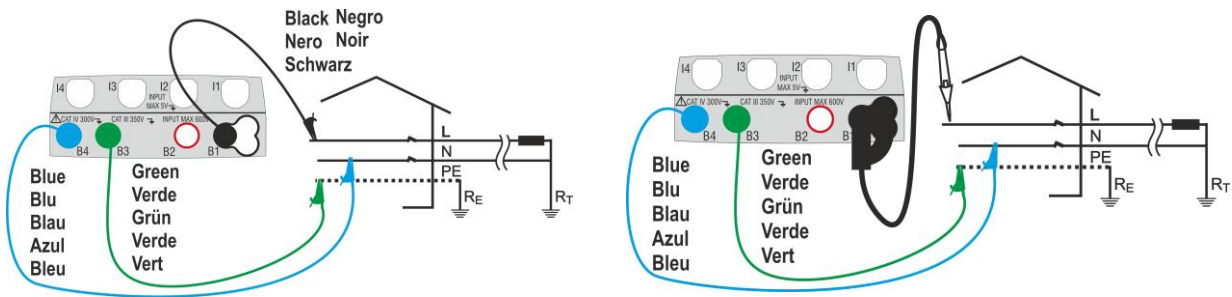
Fig. 18: Medida L-N/L-PE mono/bifásicas con cables y punta remota
