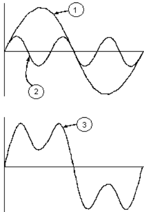
Fig. 57: Efecto de la sobreposición de dos frecuencias múltiple la una de la otra
