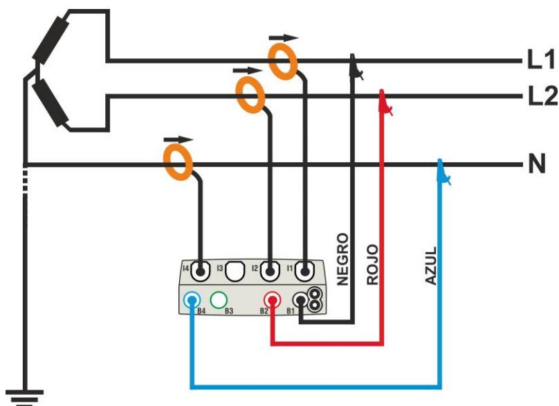
Fig. 42: Conexión para medida en sistema Bifásico 3φ-Y Abierta – sistemas USA
