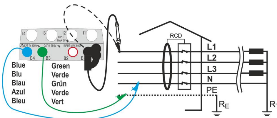
Fig. 13: Conexión en sistema trifásico con cables y punta remota
