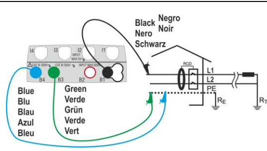
Fig. 11: Conexión sistema bifásico sin neutro (no RCD tipo B)
