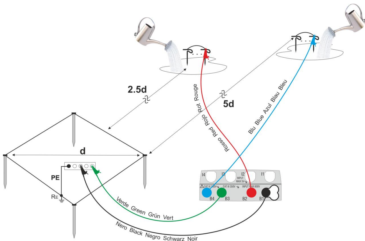
Fig. 53: Medida de tierra para dispersores de tierra de pequeñas dimensiones
