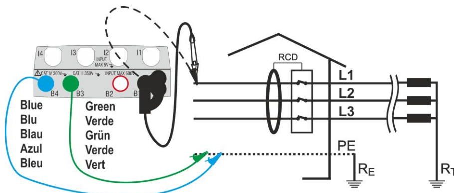
Fig. 15: Conexión en sistema trifásico (no N) con cables y punta remota (no RCD tipo B/B+)
