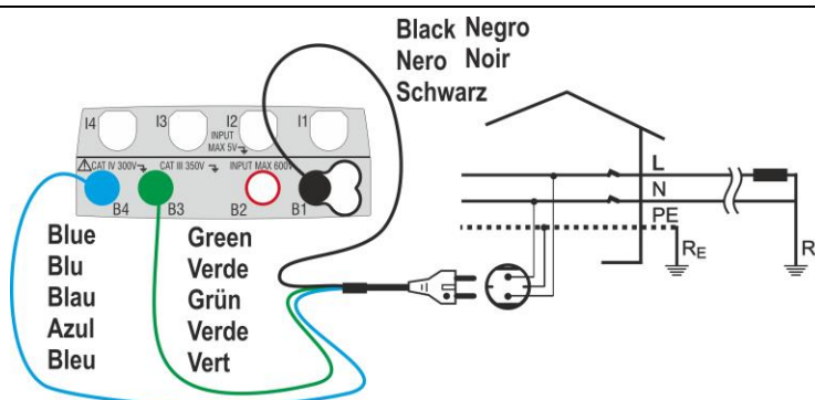
Fig. 17: Medida L-N/L-PE en instalaciones monofásicas mediante toma shuko
