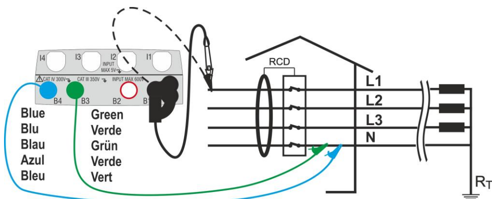
Fig. 14: Conexión en sistema trifásico (no PE) con cables y punta remota (no RCD tipo B/B+)
