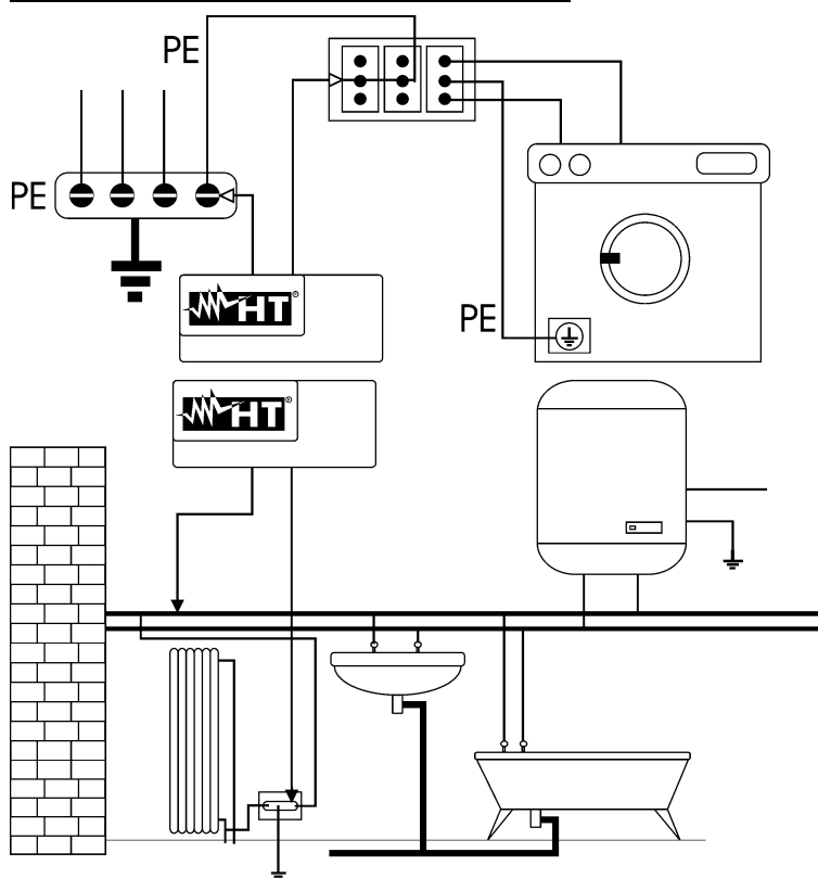
Fig. 50: Ejemplos de medidas de continuidad de los conductores
