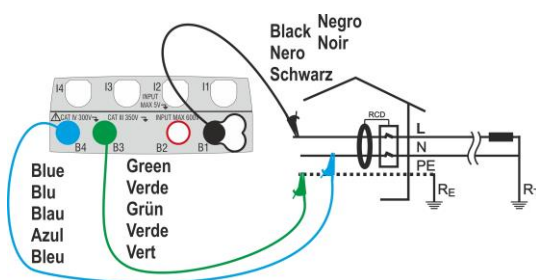
Fig. 12: Conexión en sistema monofásico con cables y punta remota
