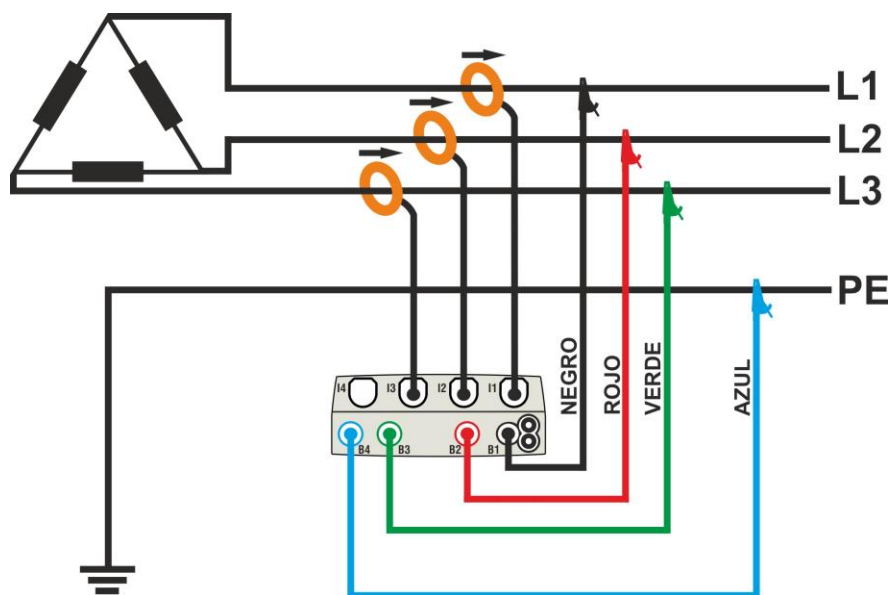
Fig. 39: Conexión para medida en sistema Trifásico 3φ-ARON
