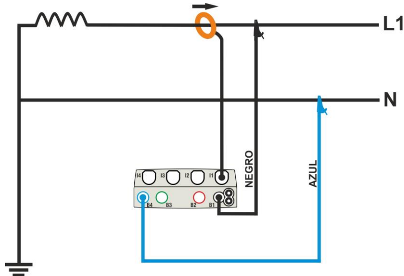
Fig. 36: Conexión para medida en sistema Monofásico 1 \phi -2HILOS
