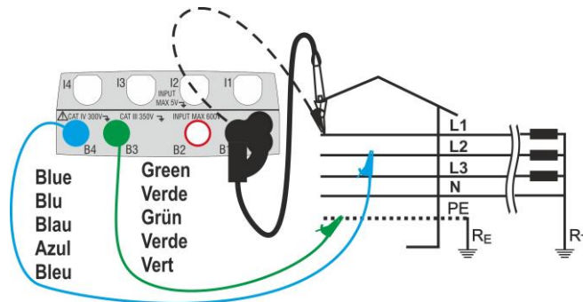
Fig. 20: Medida L-L en instalaciones trifásicas con cables y punta remota
