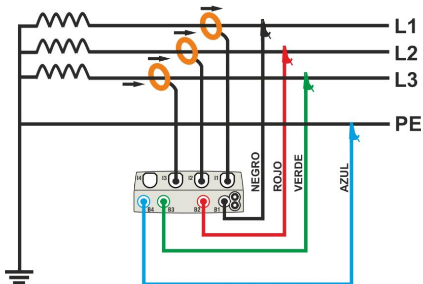
Fig. 38: Conexión para medida en sistema Trifásico 3 \phi -3HILOS
