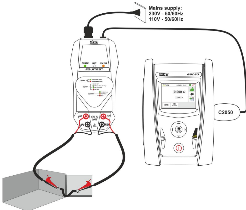
Fig. 33: Medida Continuidad de conductores de protección con accesorio EQUITEST
