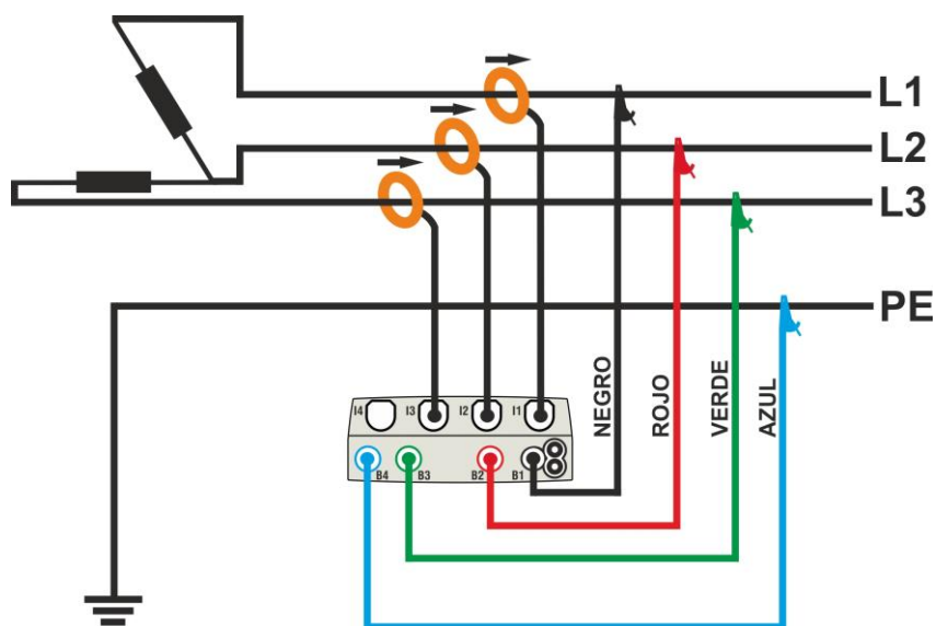
Fig. 41: Conexión para medida en sistema Trifásico 3φ-Δ Abierto – sistemas USA
