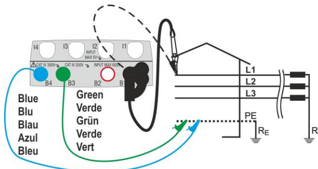
Fig. 21: Medida L-PE/L-N en instalaciones trifásicas (no N) con cables y punta remota
