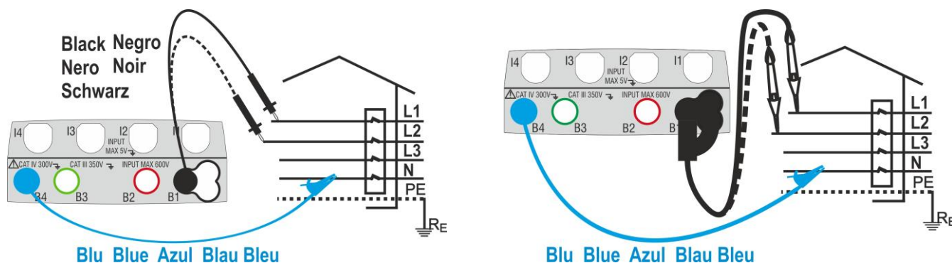
Fig. 24: Verificación del sentido cíclico de las fases 2T con dos puntas y/o punta remota
