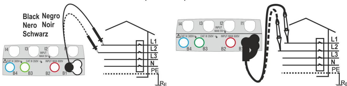
Fig. 23: Verificación del sentido cíclico de las fases 1T con una punta o punta remota
