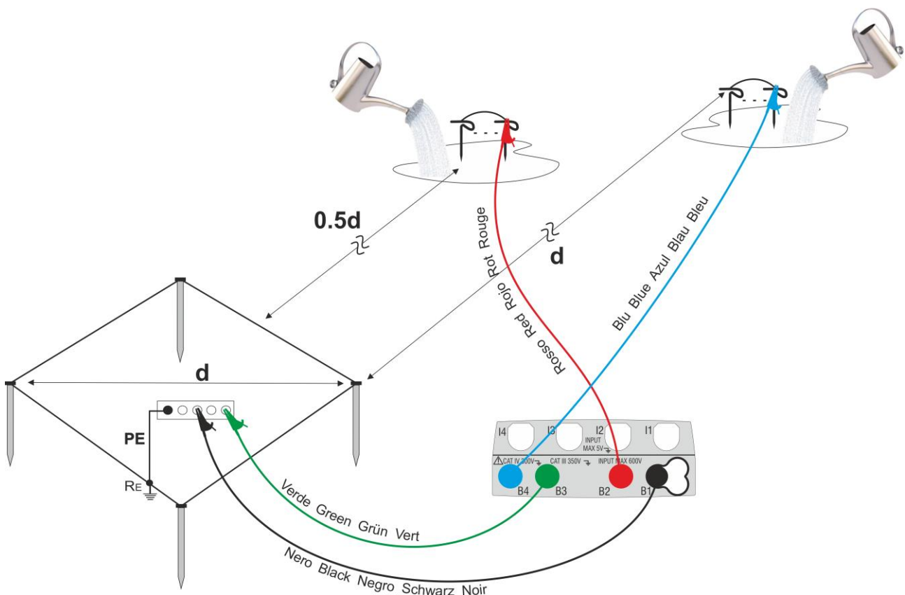
Fig. 54: Medida de tierra para dispersores de tierra de grandes dimensiones
