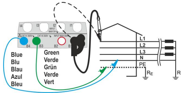
Fig. 19: Medida L-N/L-PE en trifásicas con cables y punta remota
