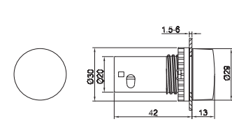
Piloto
