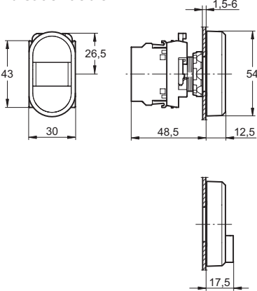
Pulsador doble
