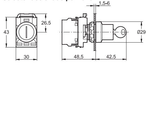
Selector accionado por llave
