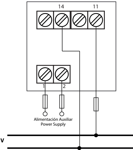
Figura 4: Medida de tensión DCB-48 Vac.
