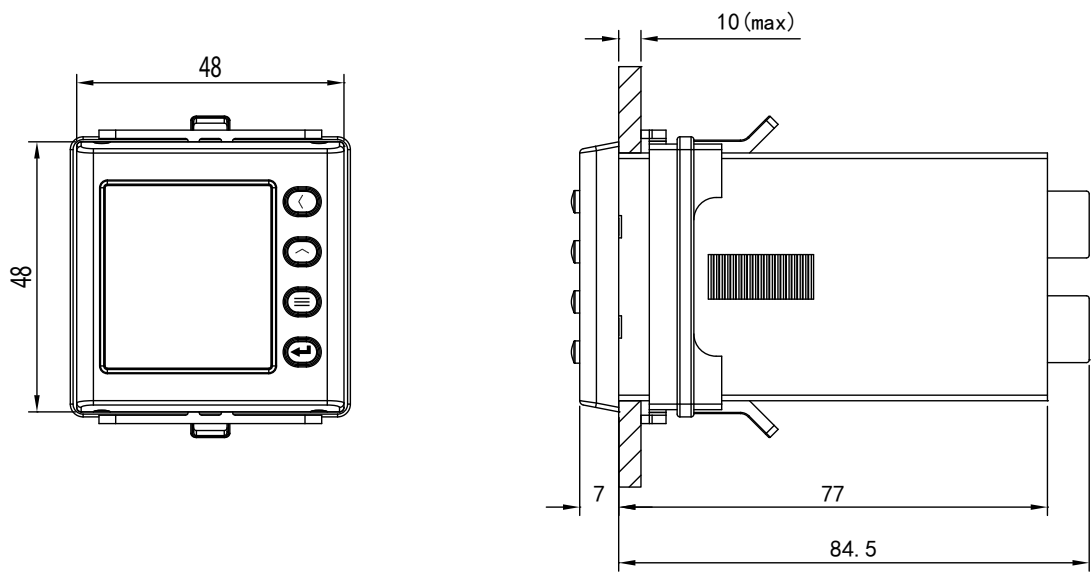
Figura 13: Dimensiones DCB-48 Vac.
