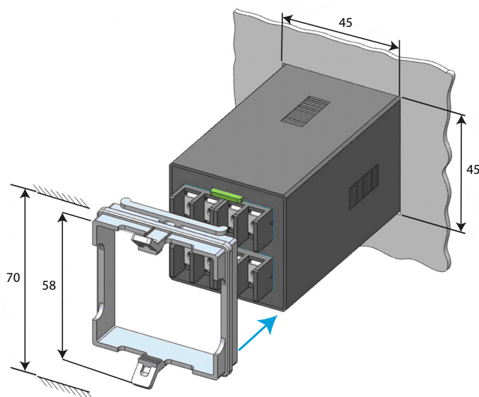
Figura 2: Instalación en panel.
