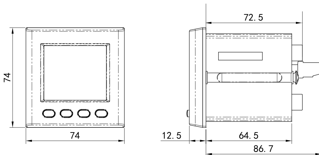
Figura 16: Dimensiones DCB-72 Vac.
