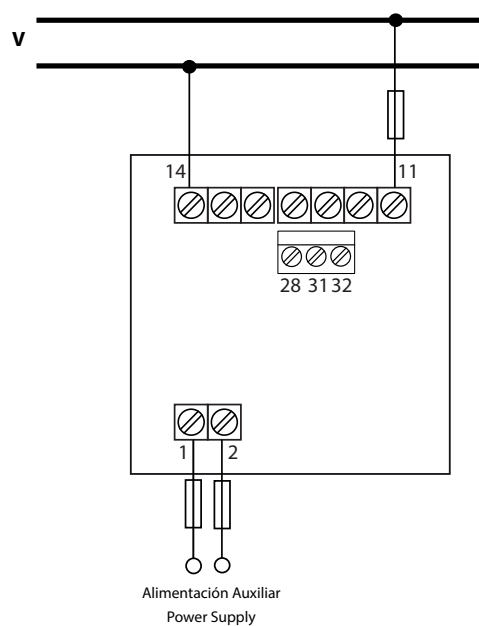
Figura 4: Medida de tensión DCB-72 Vac.
