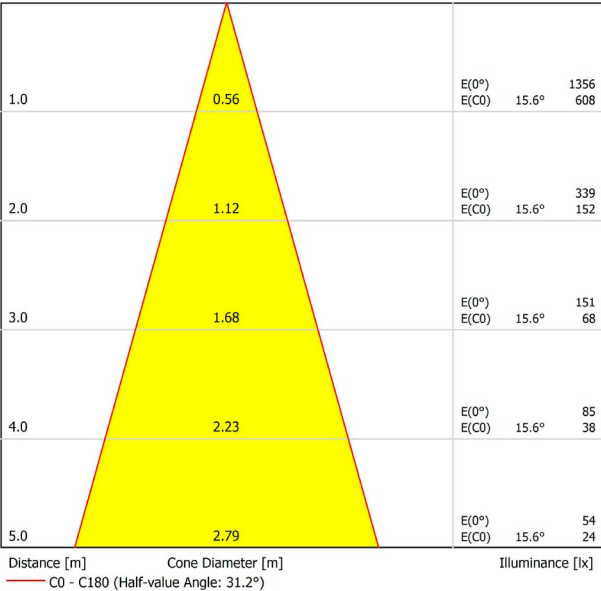
DIAGRAMA CÓNICO
