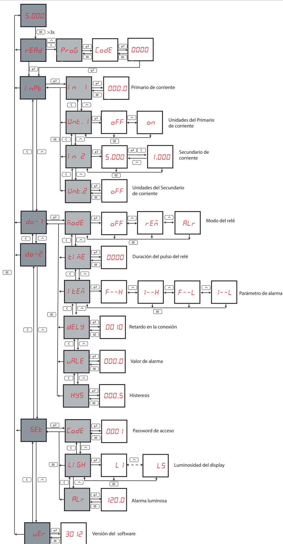
Figura 18:Menú de configuración DCB-72 Aac (con relés)
