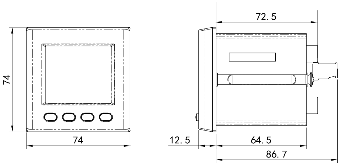
Figura 16: Dimensiones DCB-72 Aac.
