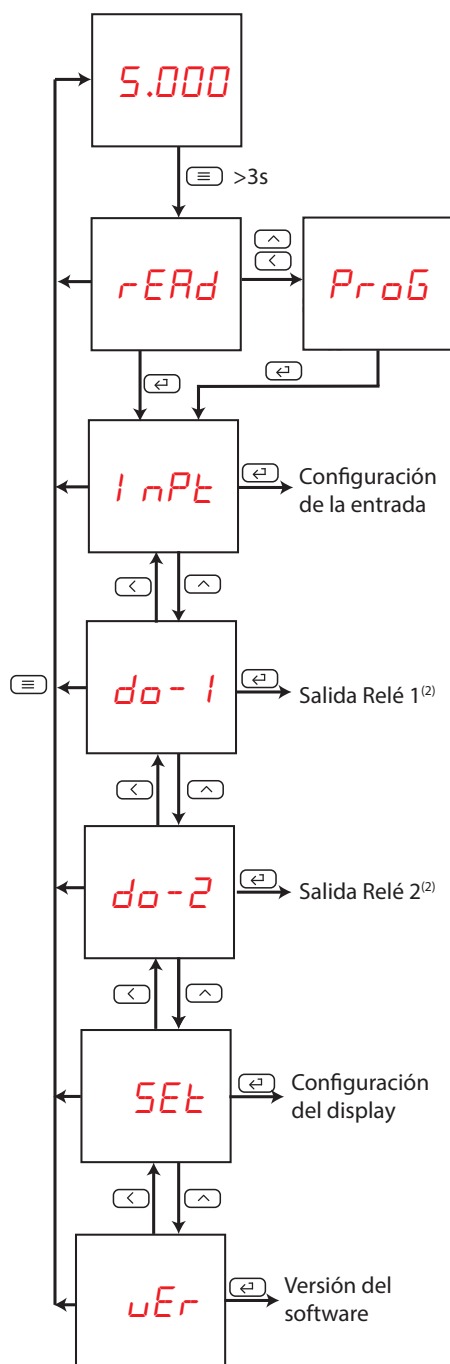
Figura 6: Menú de configuración DCB-72 Aac.
