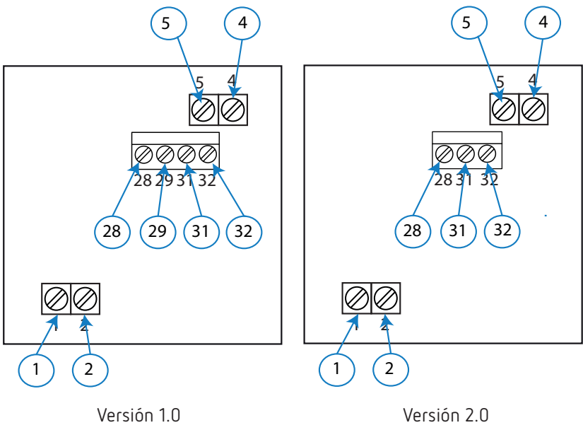
Figura 3:Bornes DCB-72 Aac.
