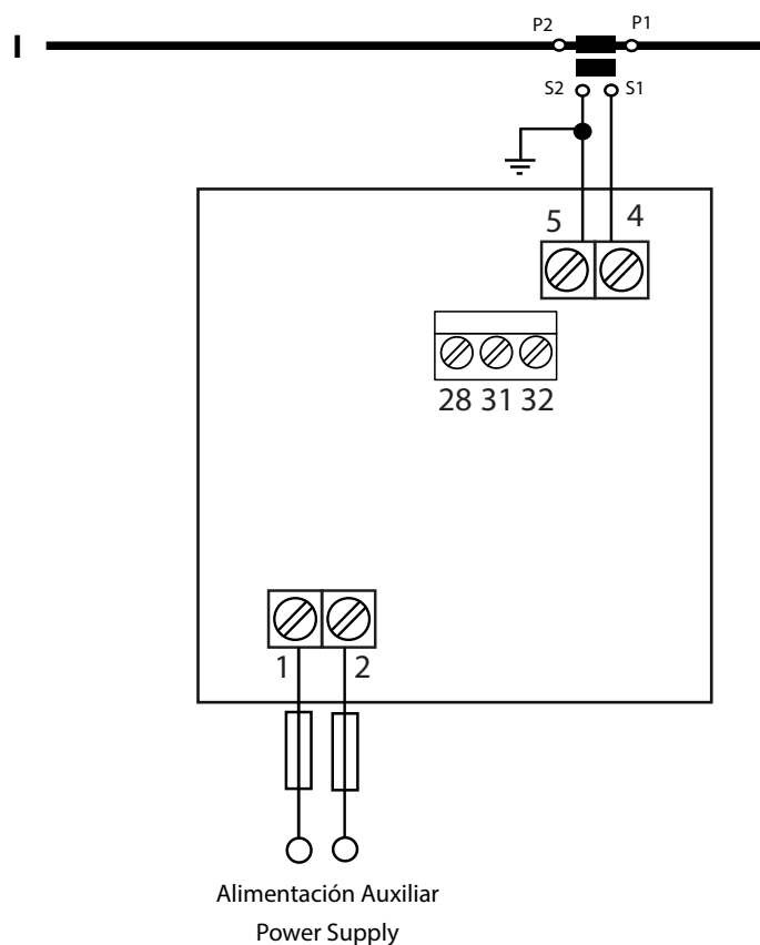
Figura 4: Medida de corriente DCB-72 Aac.
