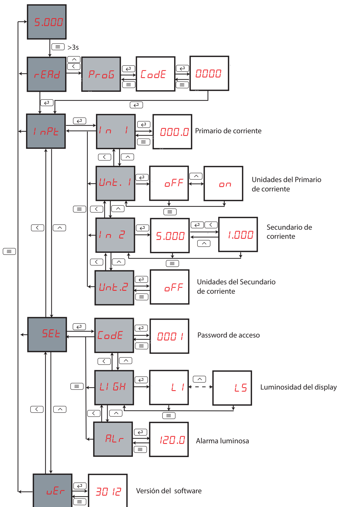
Figura 17: Menú de configuración DCB-72 Aac
