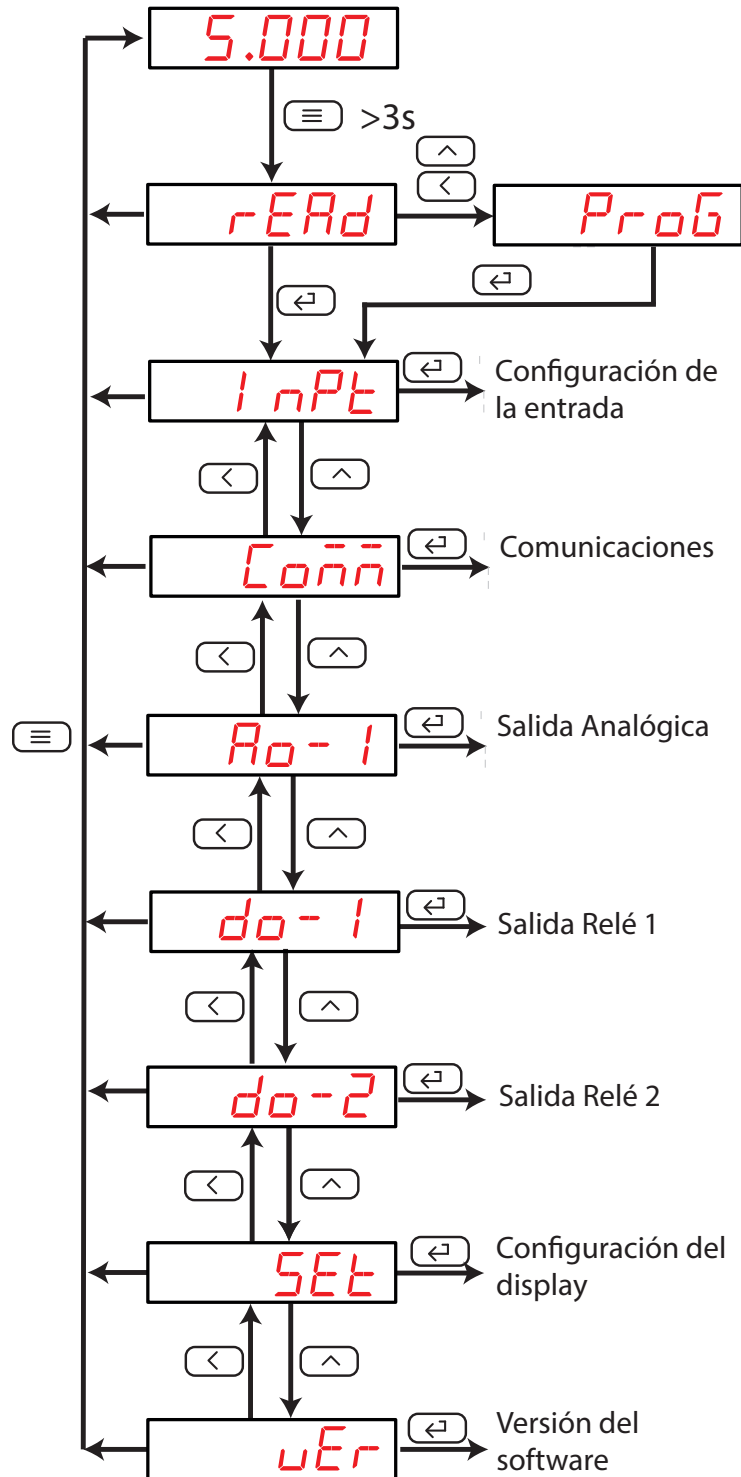
Figura 7: Menú de configuración DHC-96 Aac.
