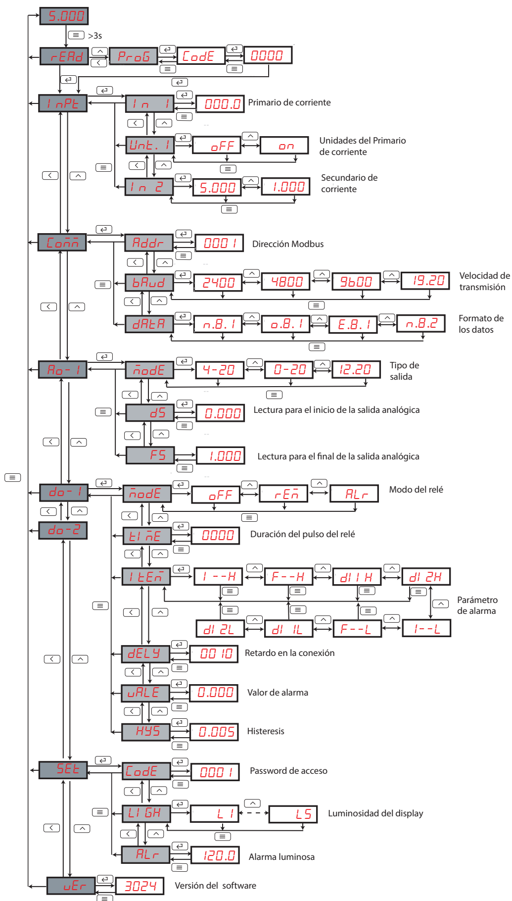
Figura 23: Menú de configuración DHC-96 Aac.
