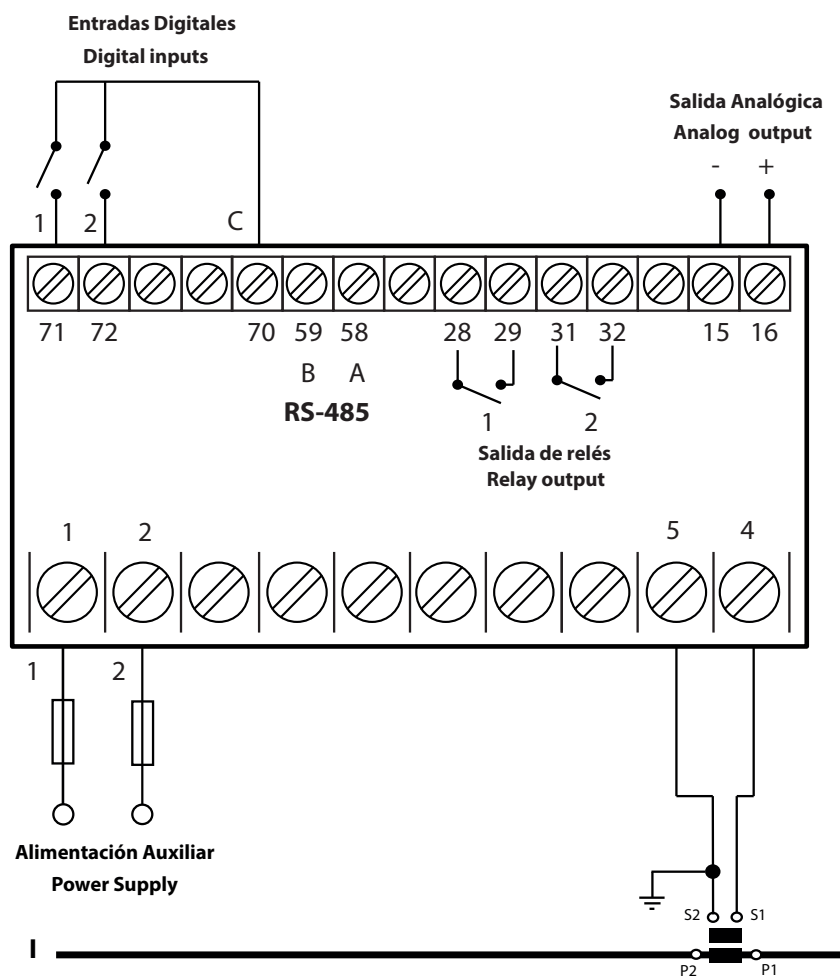
Figura 4: Medida de corriente DHC-96 Aac.
