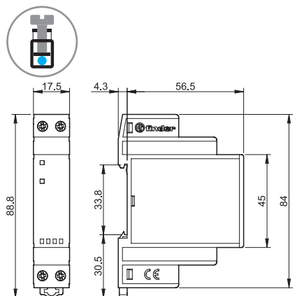
Tipo 77.01 DC Borne de jaula
