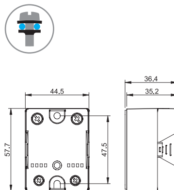
Tipo 77.x5 Borner a pletina
