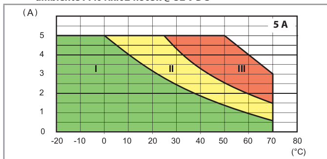
L77-1 Máxima corriente efectiva en función de la temperatura ambiente 77.01.x.024.805x @ 32 V DC
