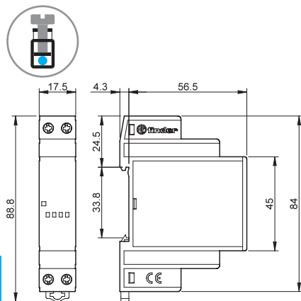
Tipo 77.01 Borne de jaula
