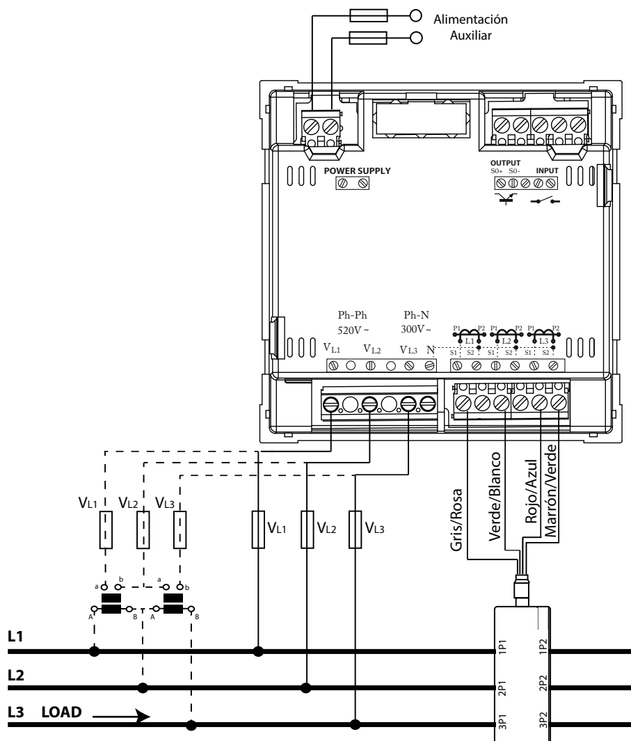
Figura 5: Medida trifásica con conexión a 3 hilos, modelo CVM-C5-MC-IC.
