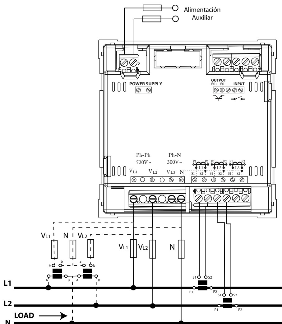
Figura 7: Medida bifásica con conexión a 3 hilos.
