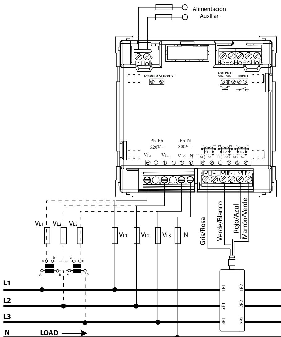
Figura 3: Medida trifásica con conexión a 4 hilos, modelo CVM-C5-MC-IC.
