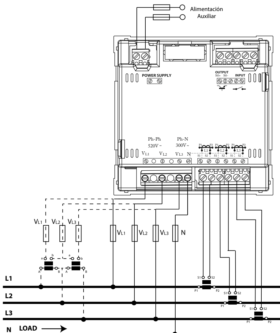
Figura 2: Medida trifásica con conexión a 4 hilos, modelos CVM-C5-IC y CVM-C5-mV-IC.
