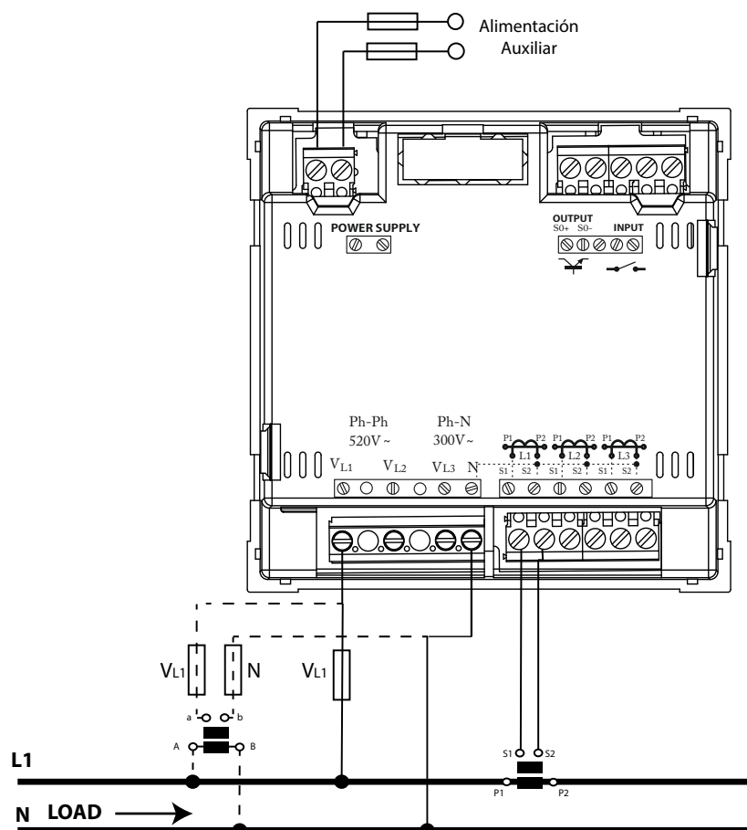
Figura 9: Medida monofásica de fase a neutro de 2 hilos.
