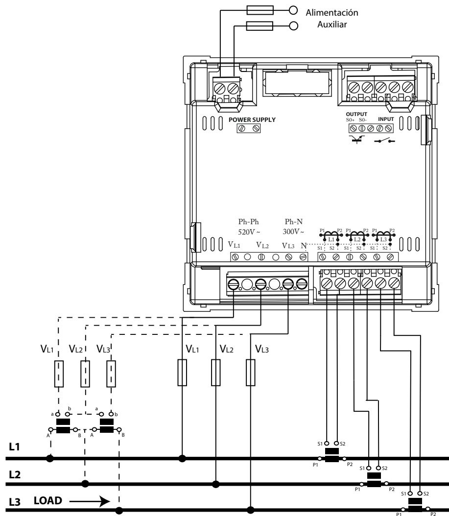
Figura 4: Medida trifásica con conexión a 3 hilos, modelos CVM-C5-IC y CVM-C5-MV-IC.
