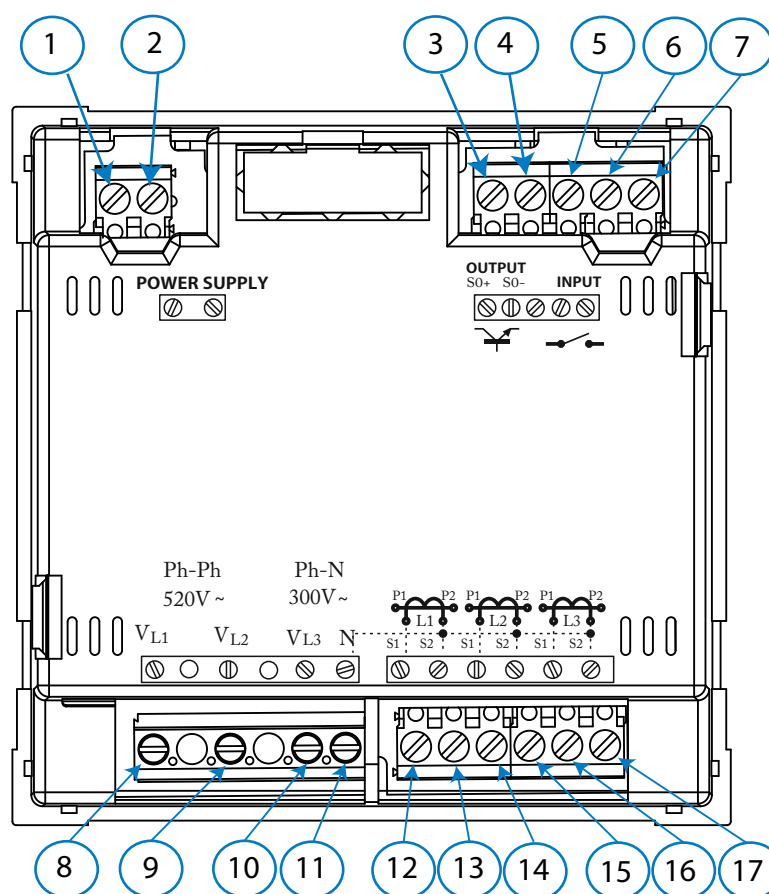
Figura 1: Bornes del CVM-C5.
