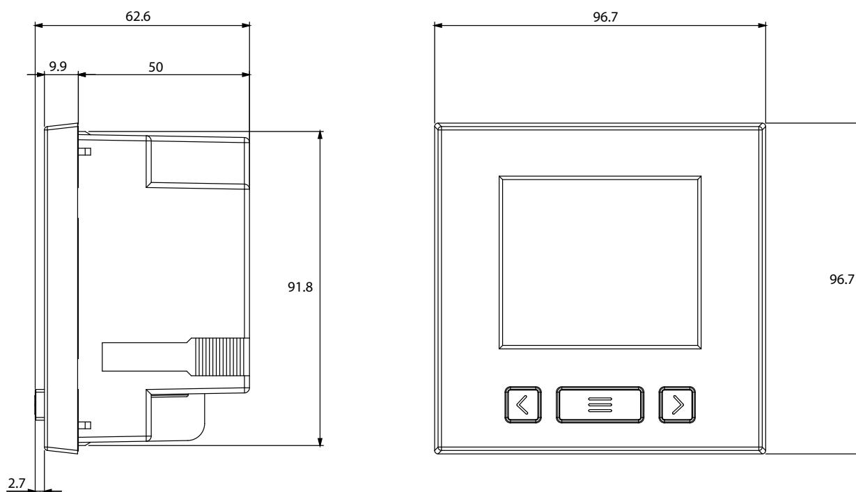
Figura 15:Dimensiones.
