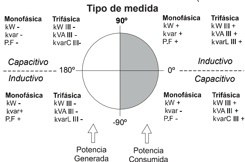
Figura 10: Cuatro cuadrantes de CVM-C5.
