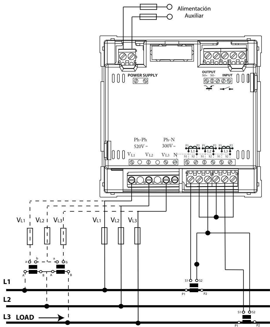
Figura 6: Medida trifásica con conexión a 3 hilos y transformadores en conexión ARON.
