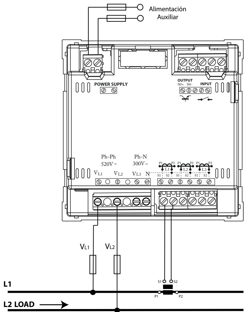
Figura 8: Medida monofásica de fase a fase de 2 hilos.
