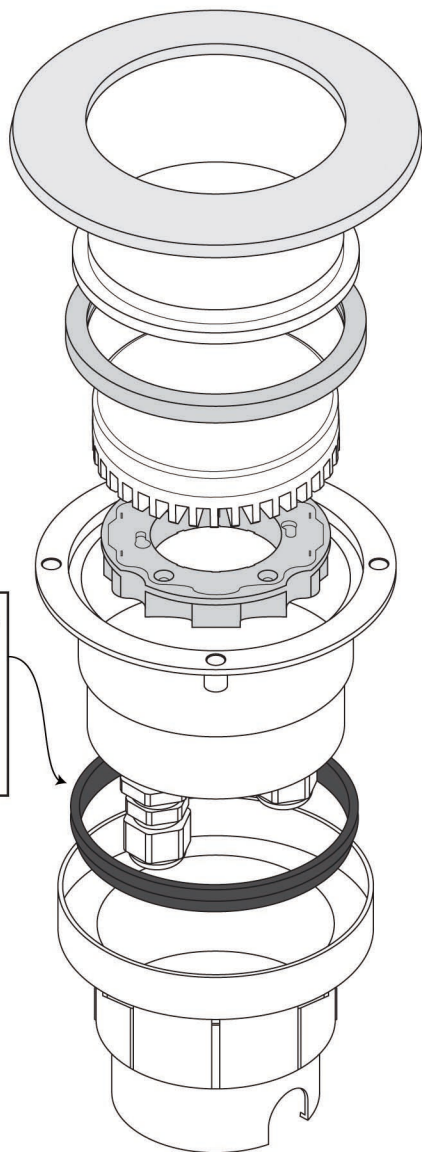
FIXATION GASKET
