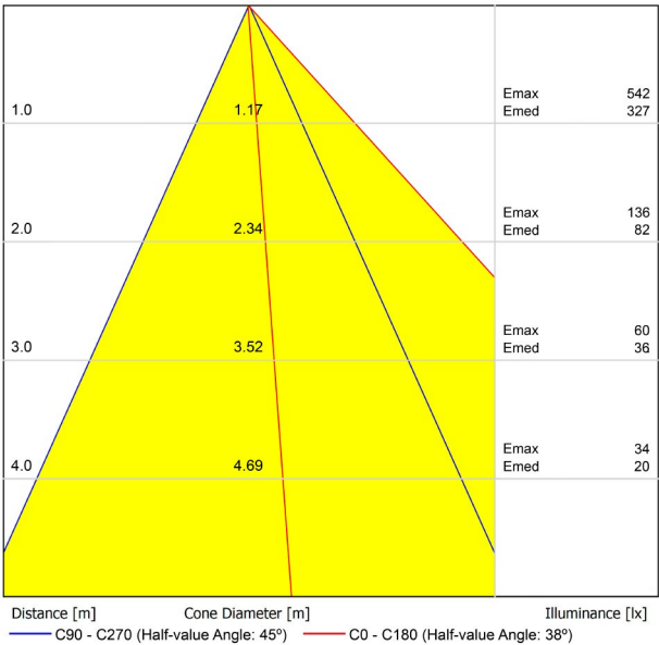
DIAGRAMA CÓNICO
