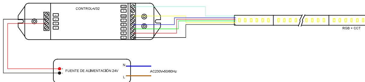
Figura 1. Esquema de conexión.
