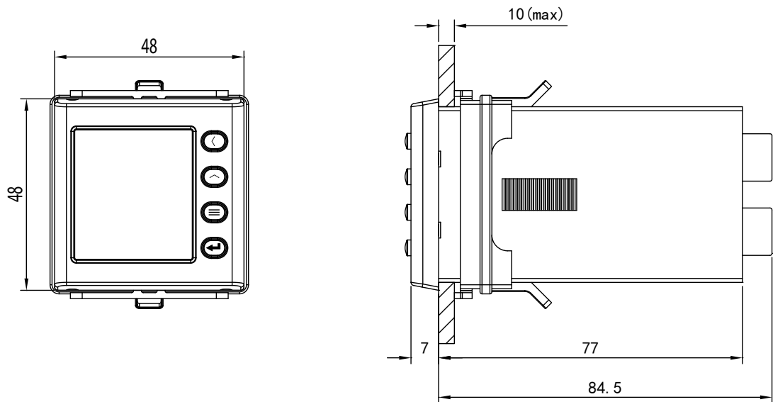
Figura 13: Dimensiones DCB-48 Vdc.
