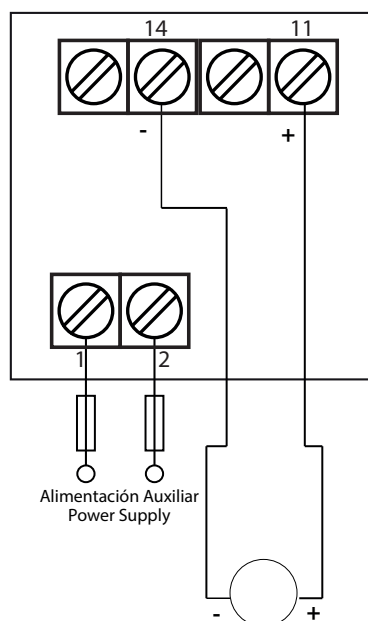
Figura 4: Medida de tensión DCB-48 Vdc.
