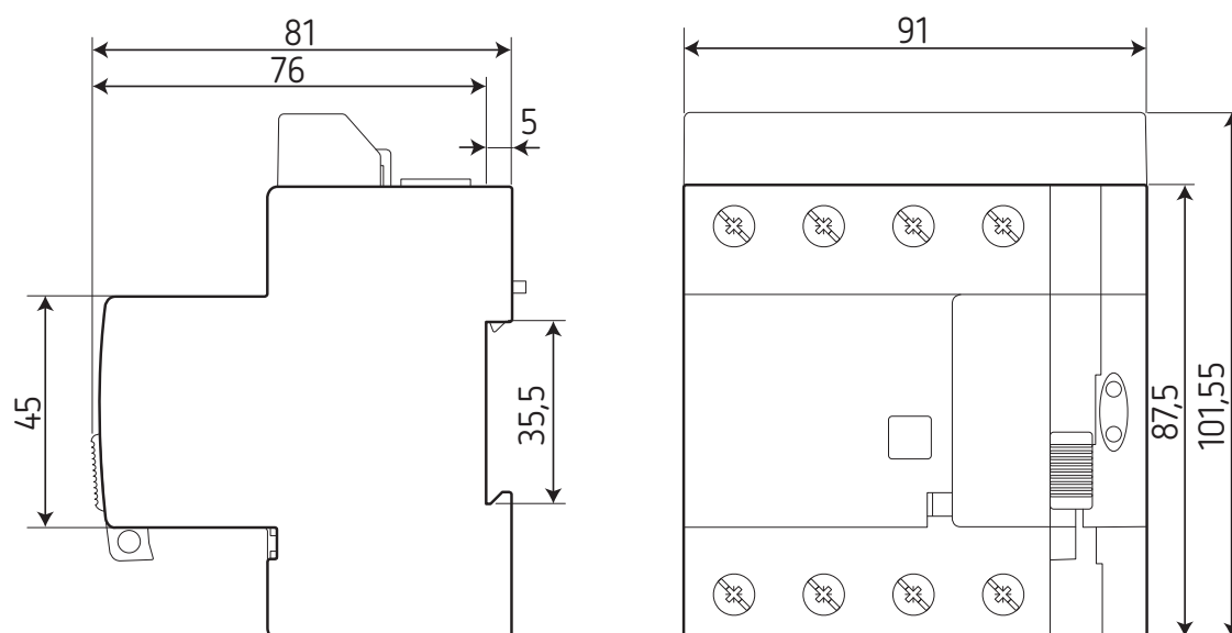
Figura 12: Dimensiones REC4-4P.
