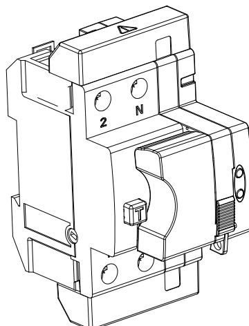
Figura 9: REC4 en modo automático, pasador selector de modo en ON.
