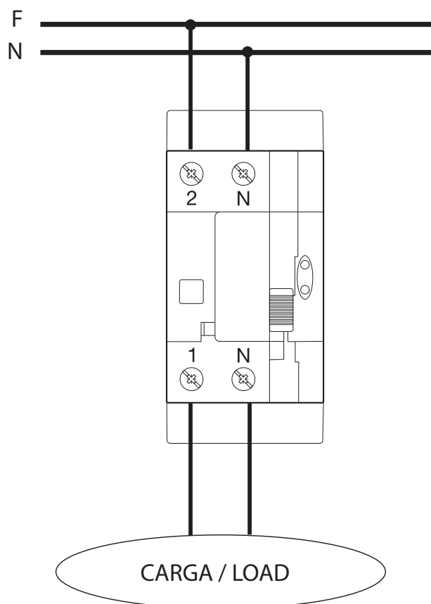
Figura 1: Esquema de conexión REC4-2P.
