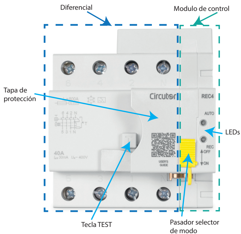
Figura 5: Descripción del REC4-4P.
