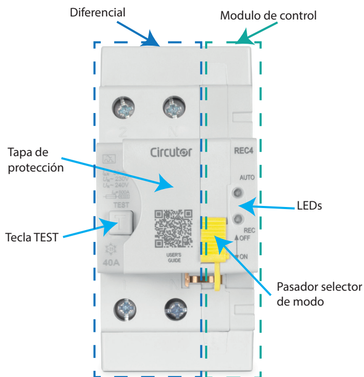
Figura 4: Descripción del REC4-2P.
