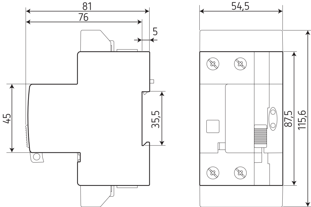
Figura 11:Dimensiones REC4-2P.
