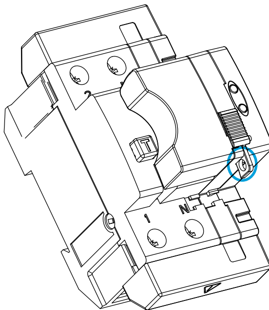
Figura 7: Orificio M2 del pasador para precintar el acceso al diferencial.
