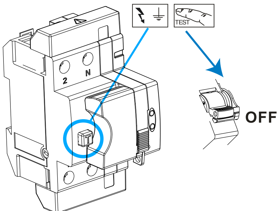
Figura 10: Secuencia de Test del interruptor diferencial.
