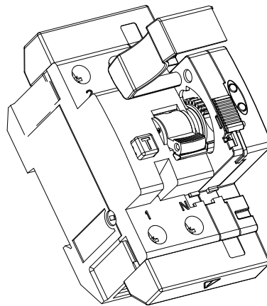
Figura 8: REC4 en modo manual, pasador selector de modo en OFF.
