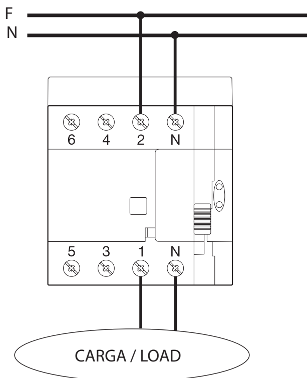
Figura 3: Esquema de conexión REC4-4P: Sistema monofásico.
