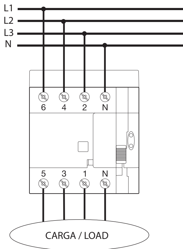
Figura 2: Esquema de conexión REC4-4P: Sistema trifásico.
