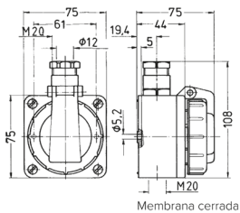
Plano 1 MB 347 Dim. en mm
