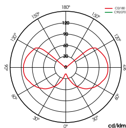
BALL 4W
