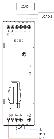
78.1D - Conexión de la fuente de alimentación
