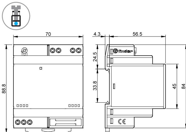
Tipo 78.61 Borne de jaula
