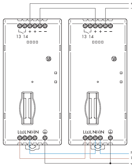
Esquema de conexión para el tipo 78.2K
