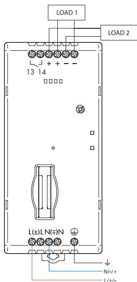
Conexiones básicas
