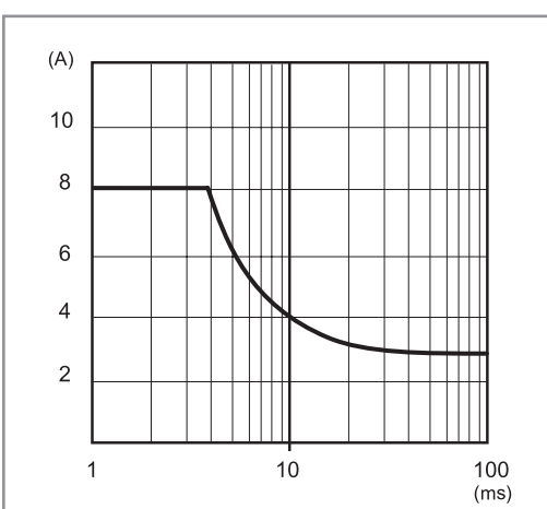
P78-6 Pico de corriente de salida en función del tiempo (78.61)
