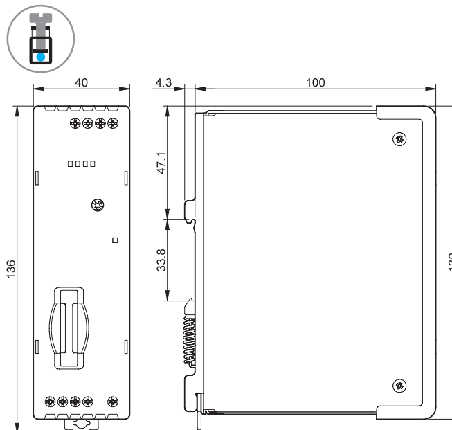
Tipo 78.1B Borne de jaula
