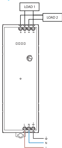
Esquema de conexión para el tipo 78.1A
