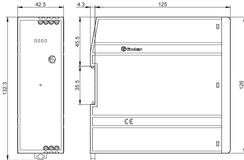
Tipo 78.2A Borne de jaula
