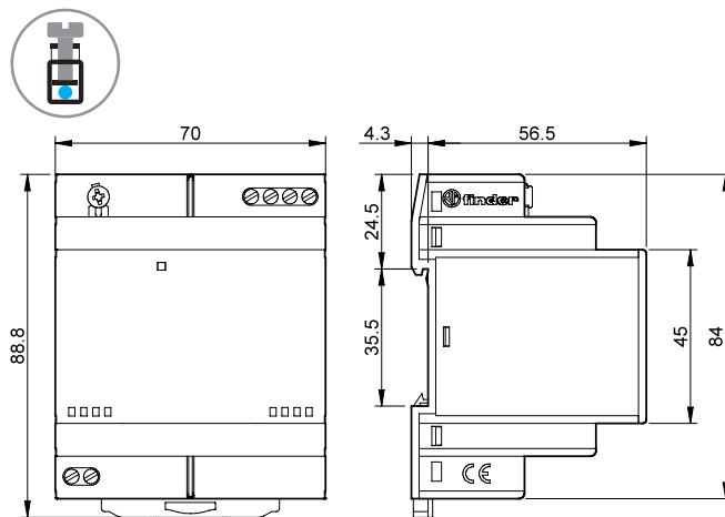
Tipo 78.1B Borne de jaula
