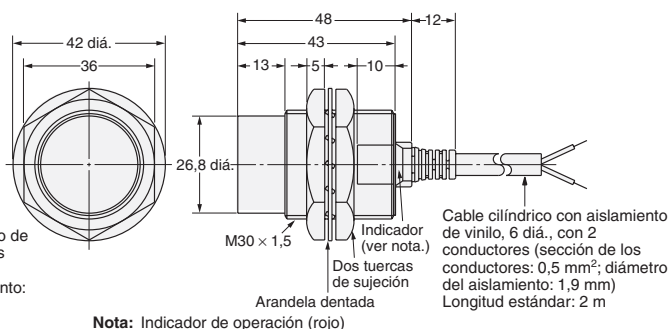
Fig. 8 : E2E-X18MY□
