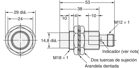
Fig. 12 : E2E-X10MY□-M1
