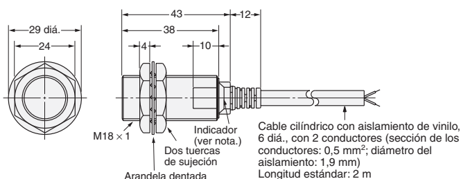
Fig. 7 : E2E-X10Y□
