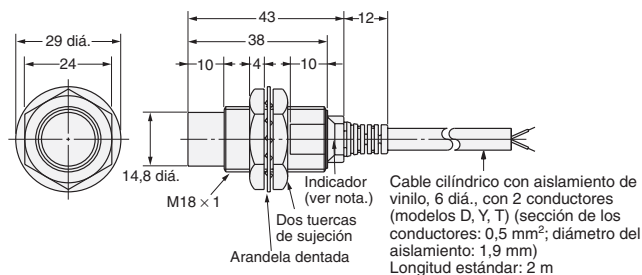
Fig. 6 : E2E-X10MY□
