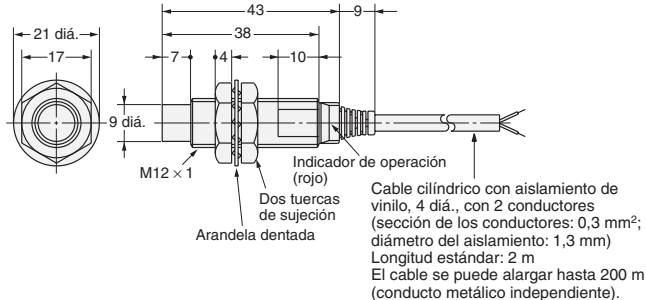
Fig. 4 : E2E-X5MY□
