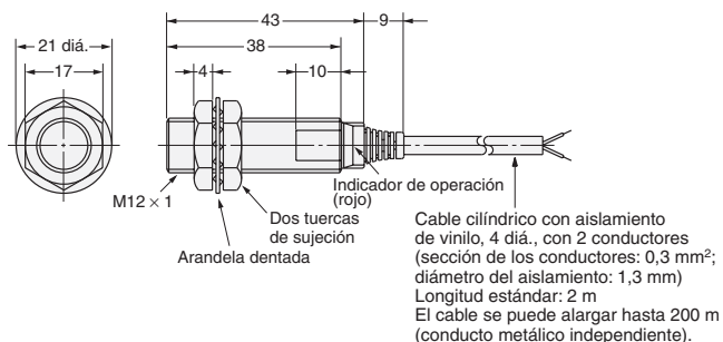
Fig. 3 : E2E-X2Y□
