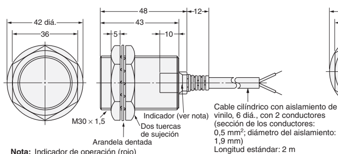
Fig. 7 : E2E-X10Y□
