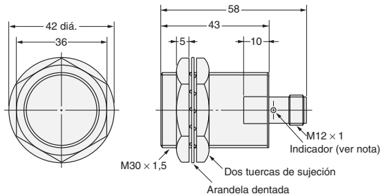
Fig. 13 : E2E-X10Y□-M1
