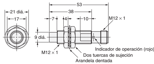
Fig. 10 : E2E-X5MY□-M1
