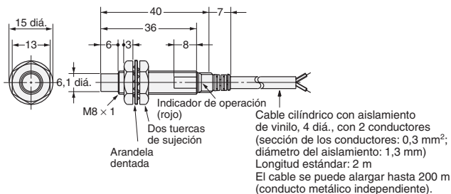
Fig. 2 : E2E-X2MY□
