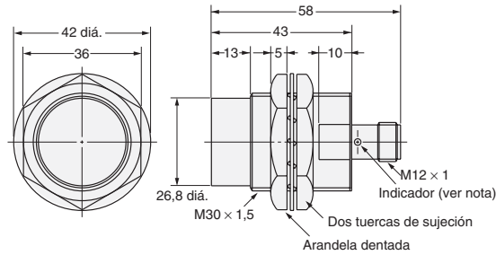
Fig. 14 : E2E-X18MY□-M1
