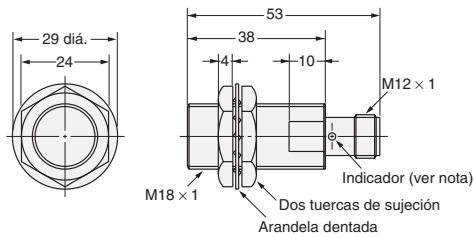
Fig. 11 : E2E-X5Y□-M1
