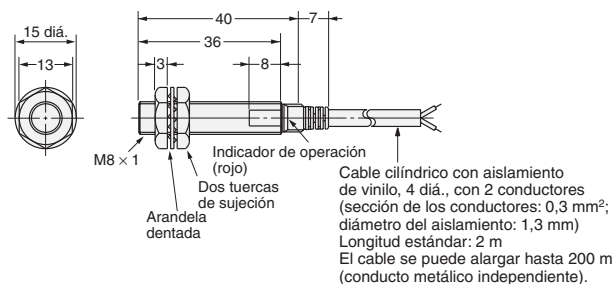
Fig. 1 : E2E-X1R5Y□
