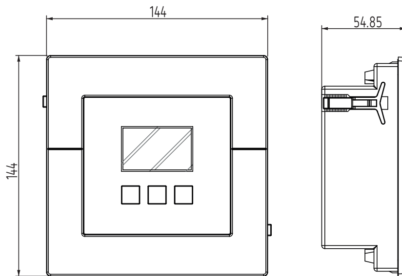
Figura 22: Dimensiones computer C Wi-Fi.
