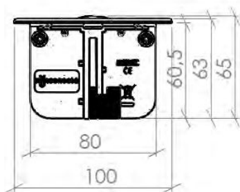
Alzado
