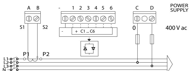
Figura 10: Conexión tipo de un regulador con un solo TC. ( En caso de usar Computer SMART III 12Vdc se usan 3 TC. Consultar manual específico. )
