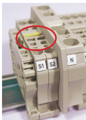
Figura 8: Puente para cortocircuitar el secundario del transformador de corriente (TC).
