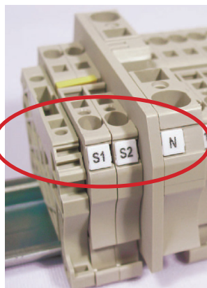
Figura 7: Terminales de conexión del transformador de corriente (TC).
