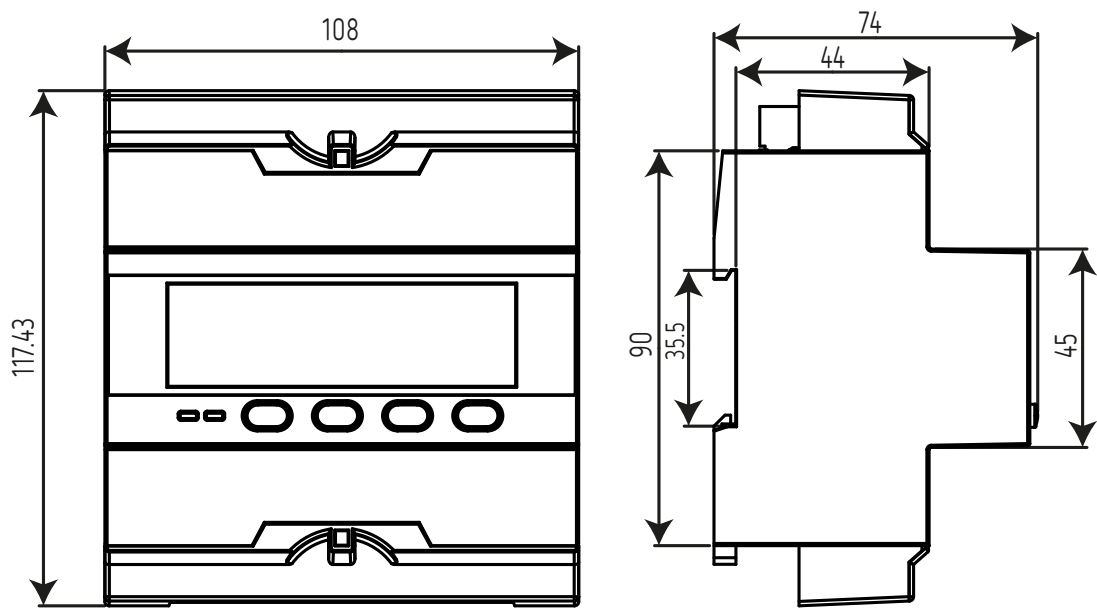
Figura 26: Dimensiones CVM-D41 DC.
