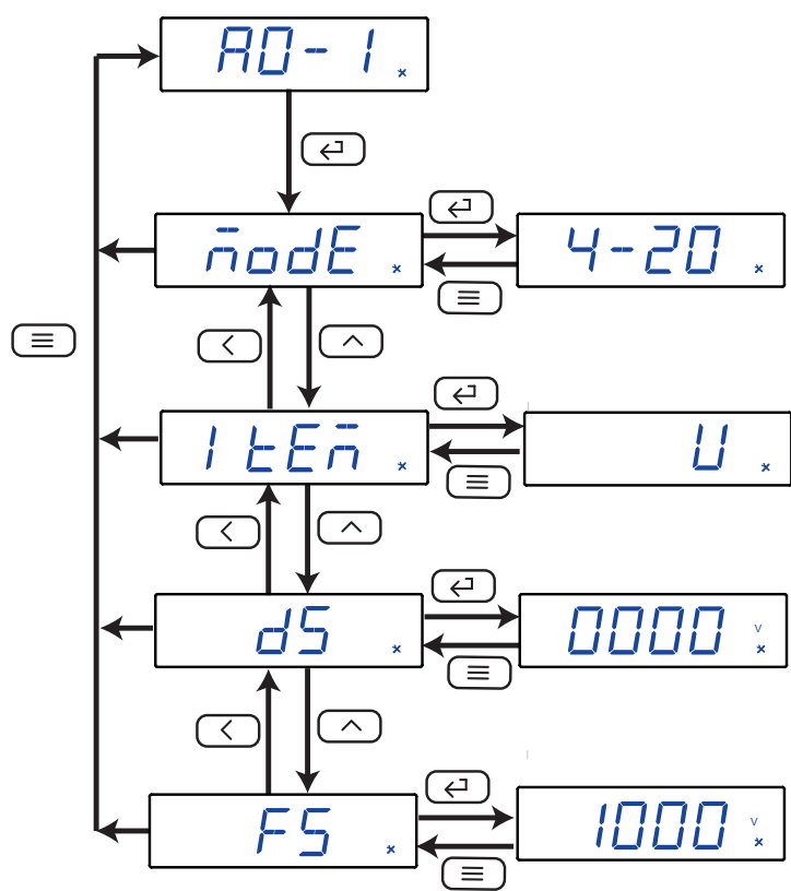
Figura 19: Menú de configuración de la salida analógica.
