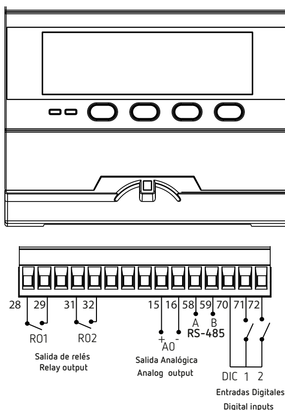
Figura 10: Salidas de relés, Entradas digitales y Salida analógica.
