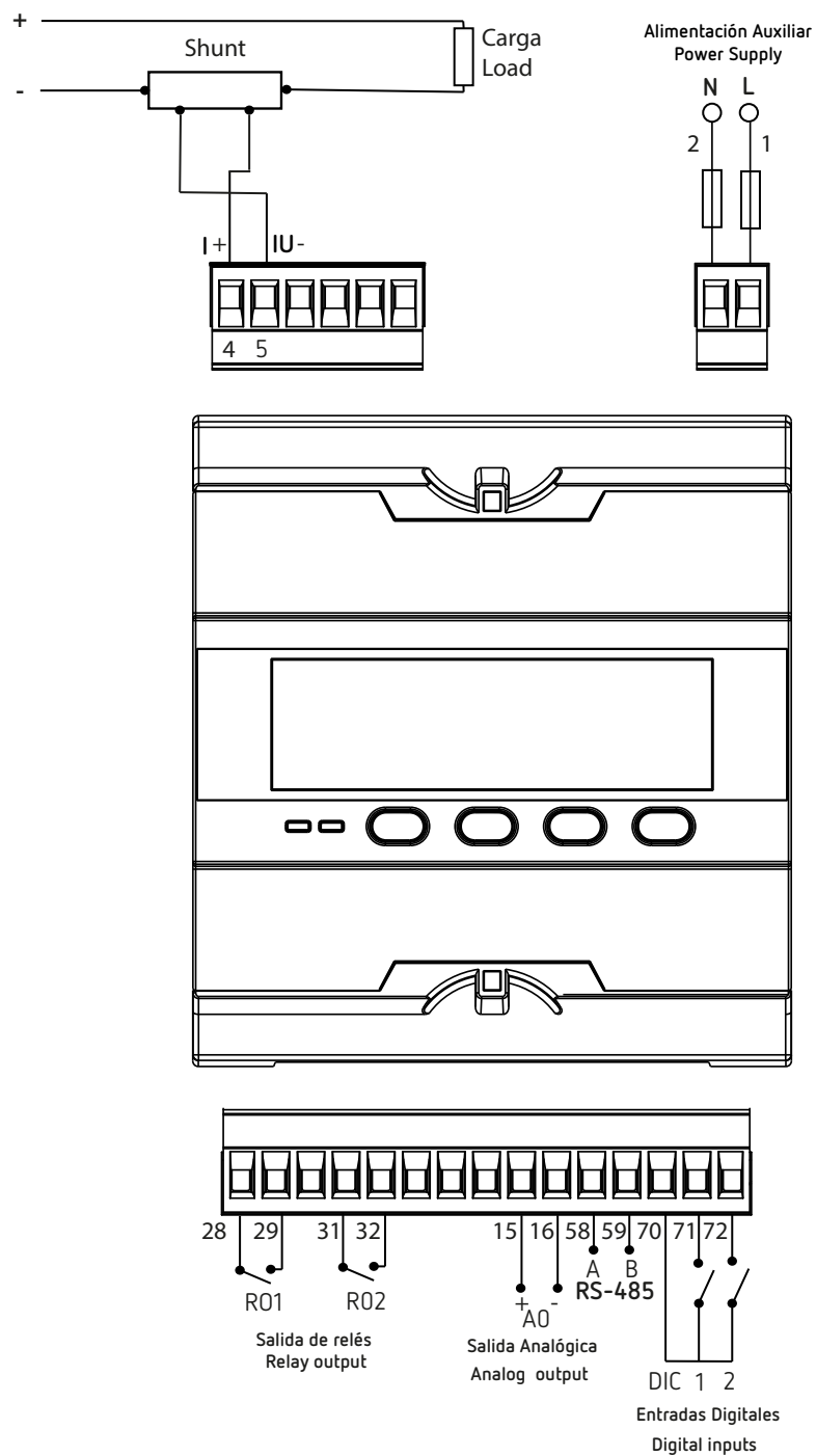
Figura 6: Medida de Corriente (Shunt polo negativo).
