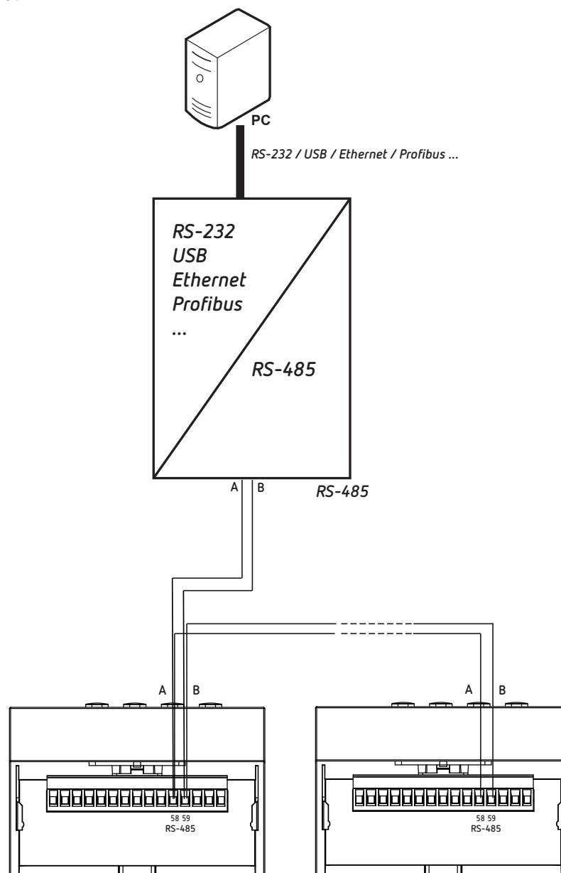
Figura 25: Esquema de conexionado RS-485.
