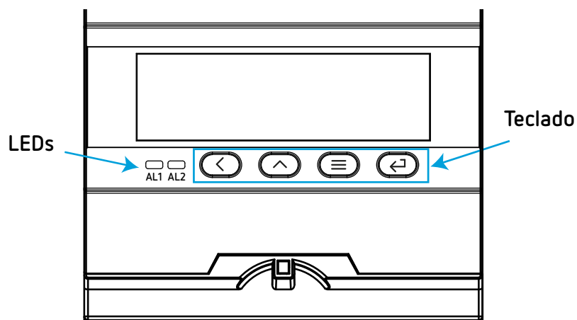
Figura 9: Teclado y LEDs CVM-D41 DC.
