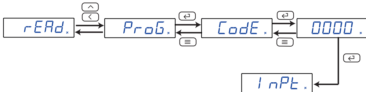
Figura 12: Acceso al menú de configuración en modo programación.
