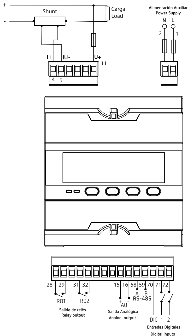
Figura 3: Medida de Tensión y Corriente (Shunt polo negativo).
