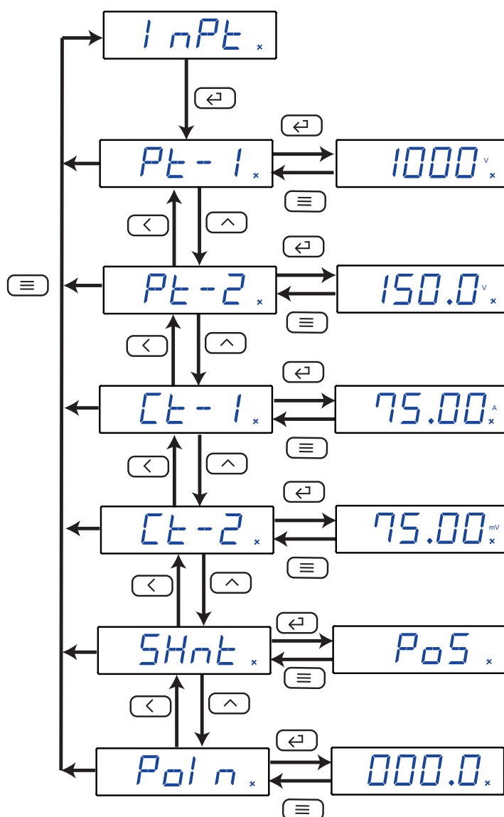
Figura 15: Menú de configuración de la entrada.
