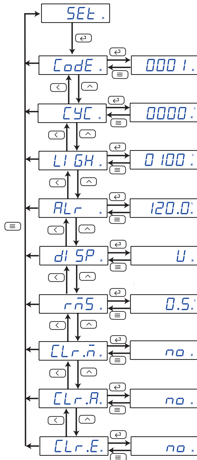
Figura 24:Menú de configuración del display.
