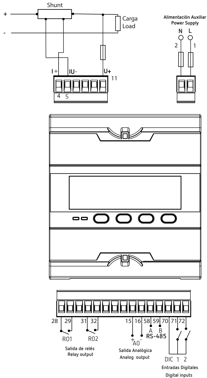
Figura 4: Medida de Tensión y Corriente (Shunt polo positivo).
