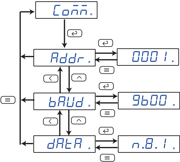
Figura 17: Menú de configuración de las comunicaciones.
