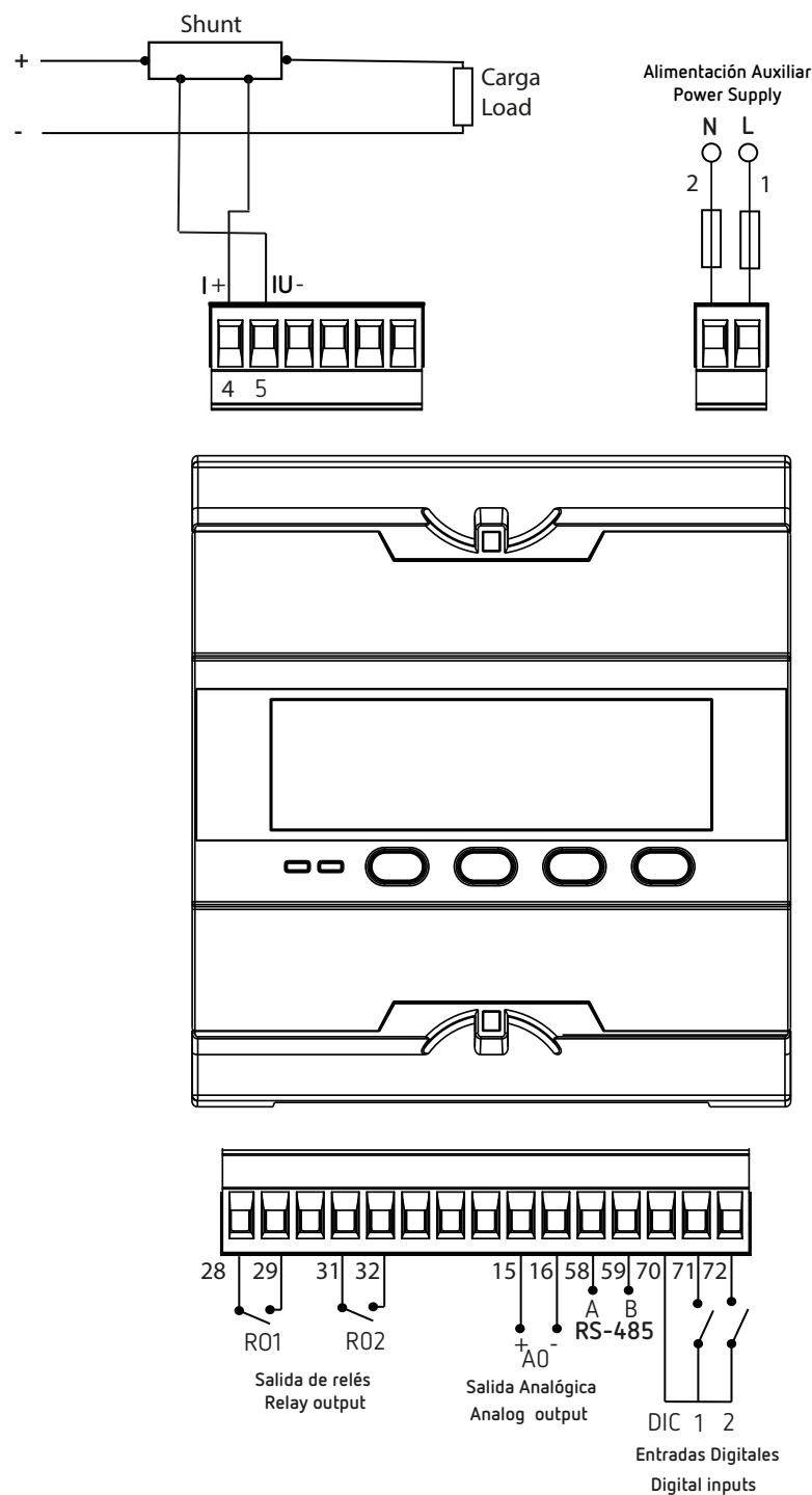
Figura 7: Medida de Corriente (Shunt polo positivo).
