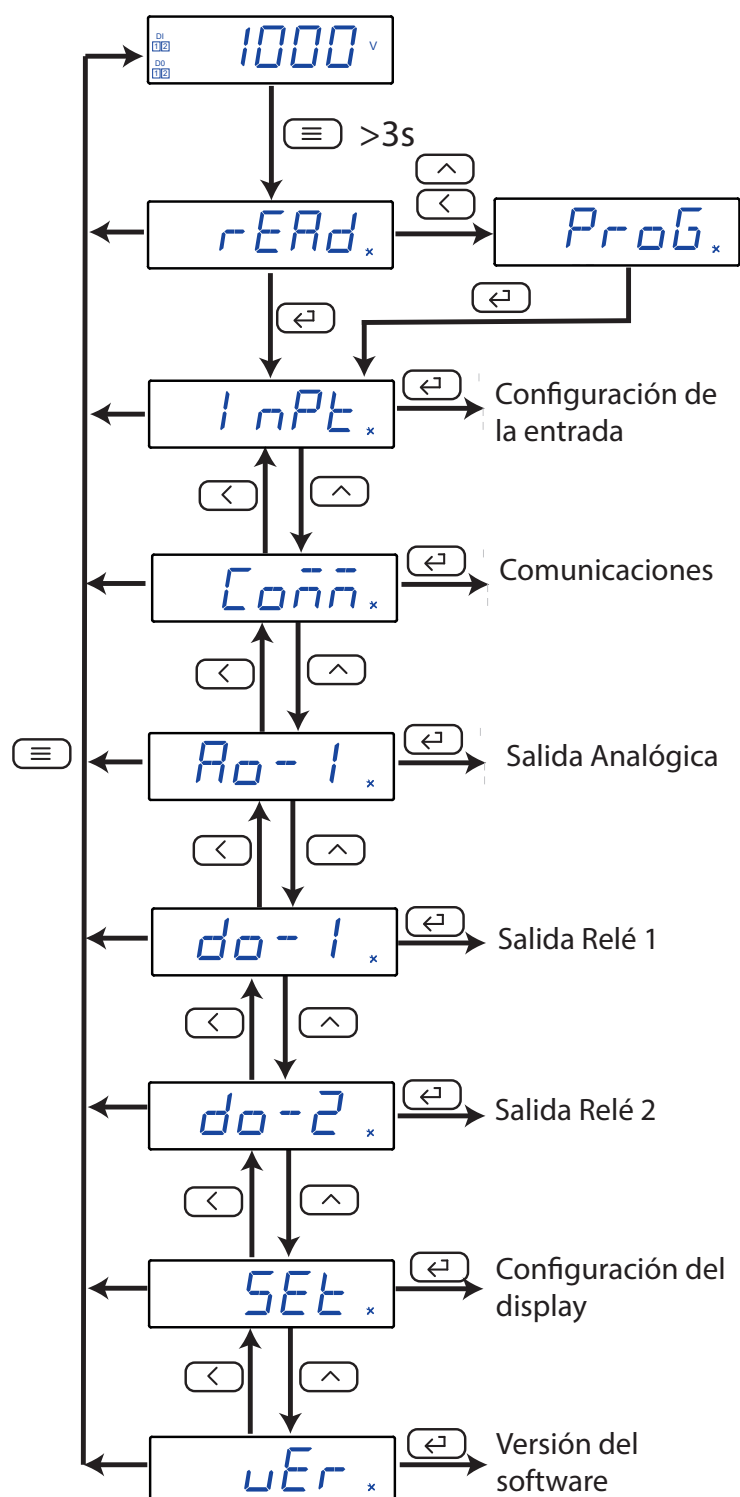
Figura 11: Menú de configuración CVM-D41 DC.
