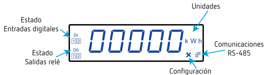
Figura 8: Display CVM-D41 DC.
