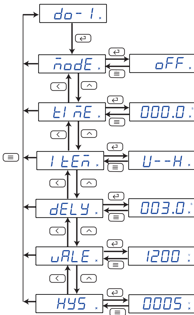
Figura 21: Menú de configuración de la salida de relé 1.
