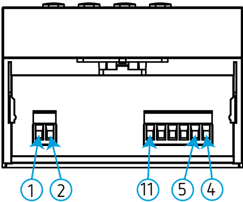
Figura 1: Bornes CVM-D41 DC (Superior).
