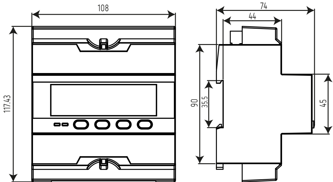
Figura 24: Dimensiones CVM-D41 DC.
