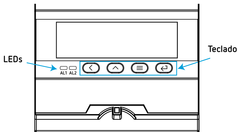
Figura 7: Teclado y LEDs CVM-D41 DC.
