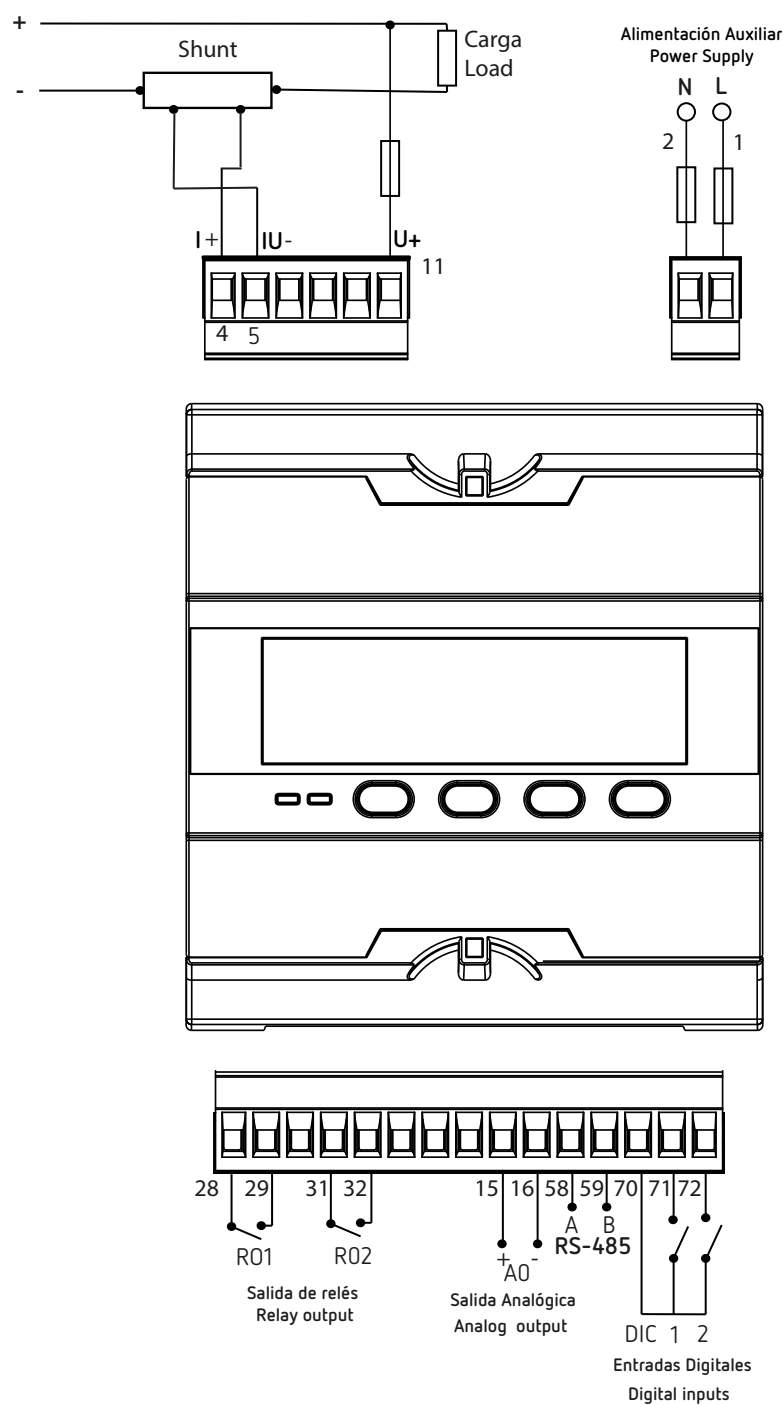
Figura 3: Medida de Tensión y Corriente.
