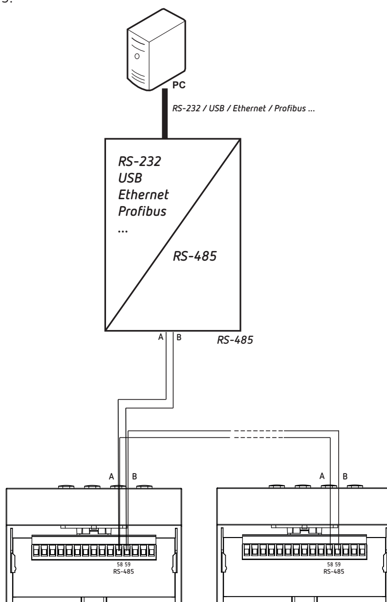
Figura 23: Esquema de conexionado RS-485.
