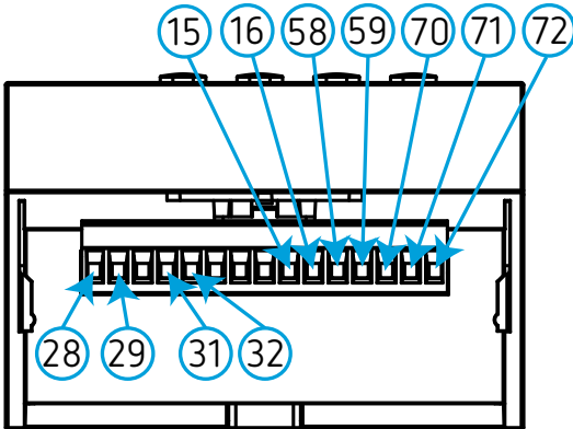
Figura 2: Bornes CVM-D41 DC (Inferior).
