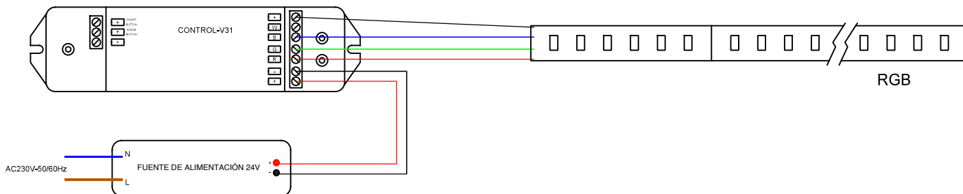
Figura 1. Esquema de conexión.
