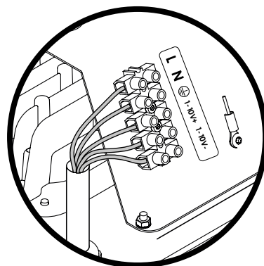
Regulación 1-10V/ 1-10V regulation
