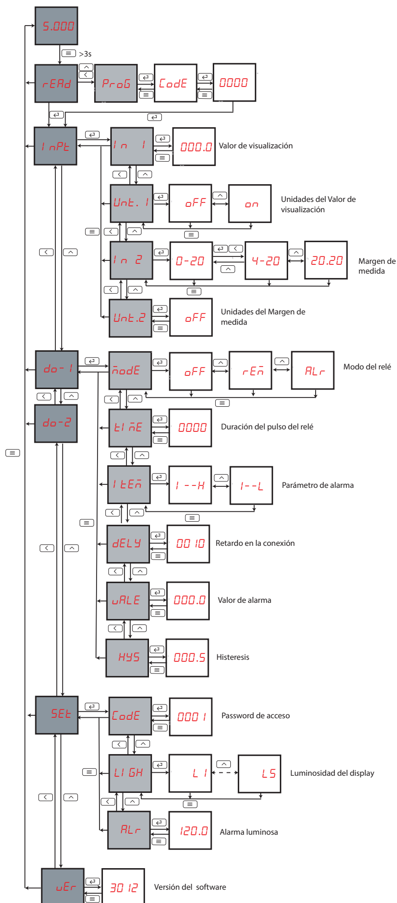
Figura 18: Menú de configuración DCB-72 mAdc (con relés)
