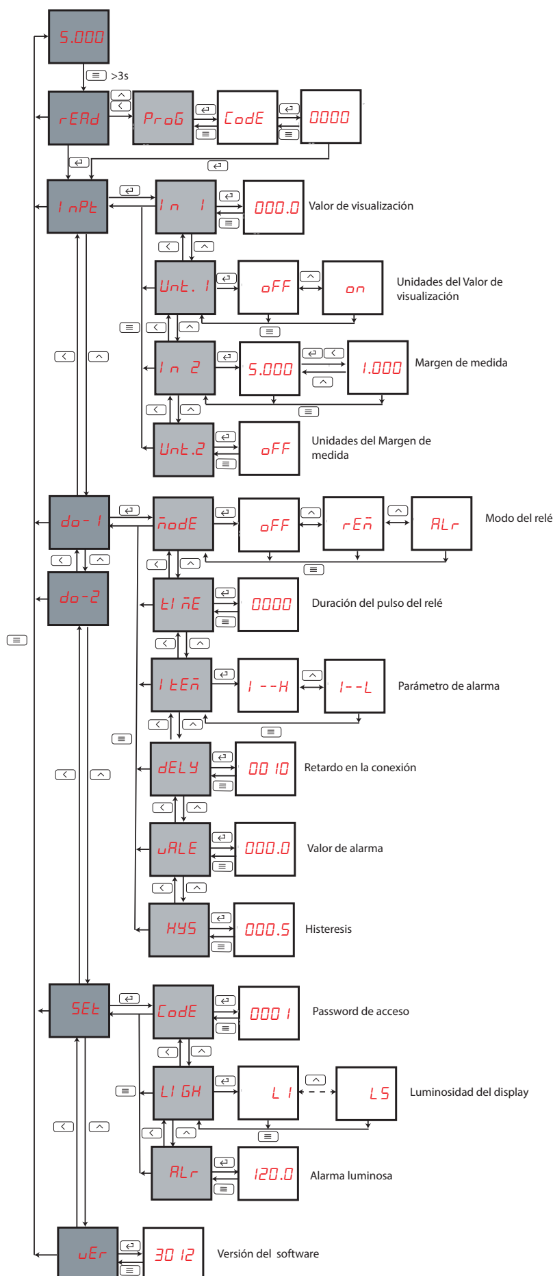
Figura 20:Menú de configuración DCB-72 Adc (con relés)
