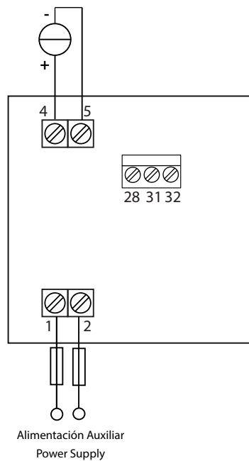
Figura 4: Medida de corriente DCB-72 Adc.
