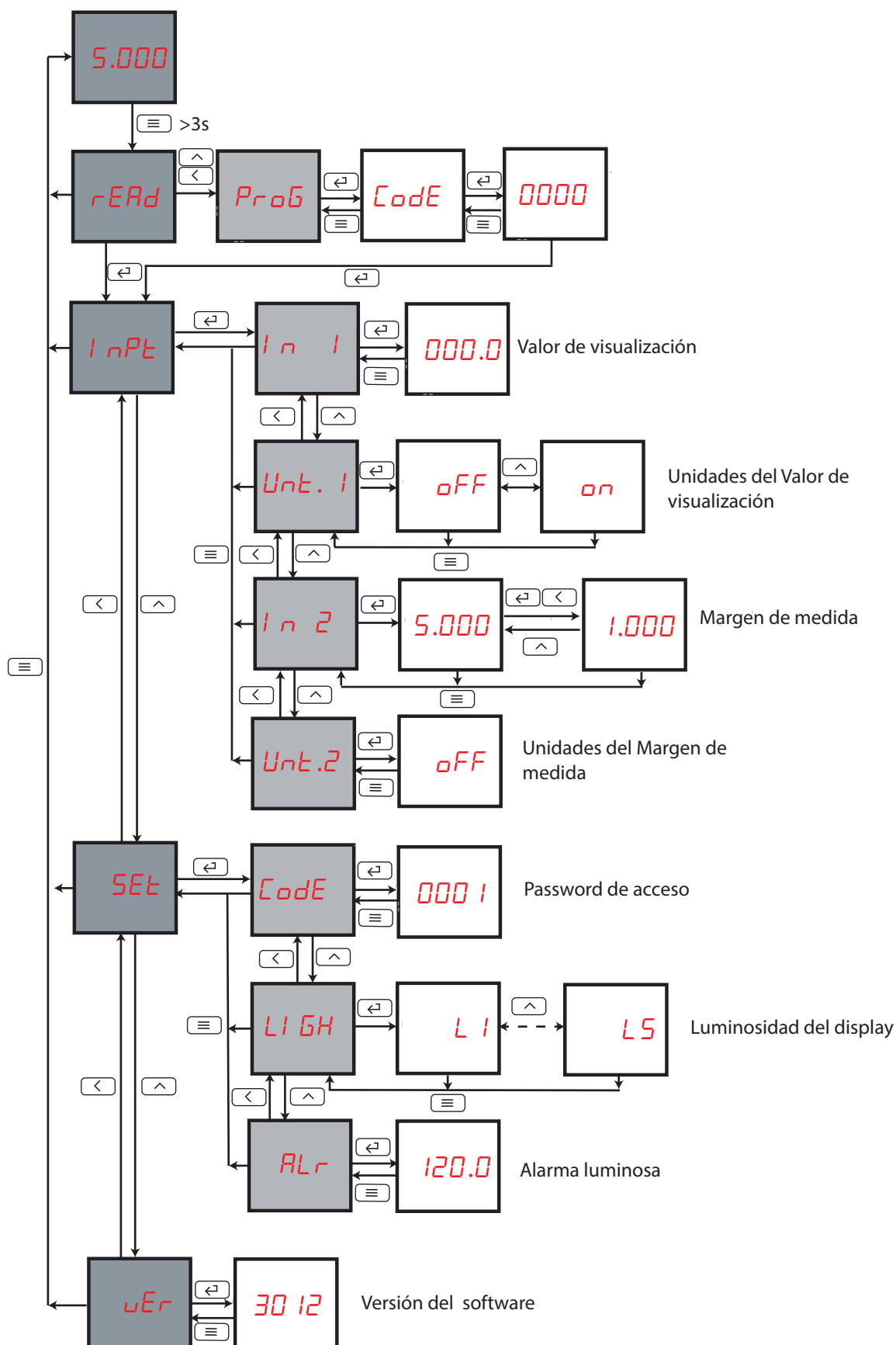
Figura 19: Menú de configuración DCB-72 Adc
