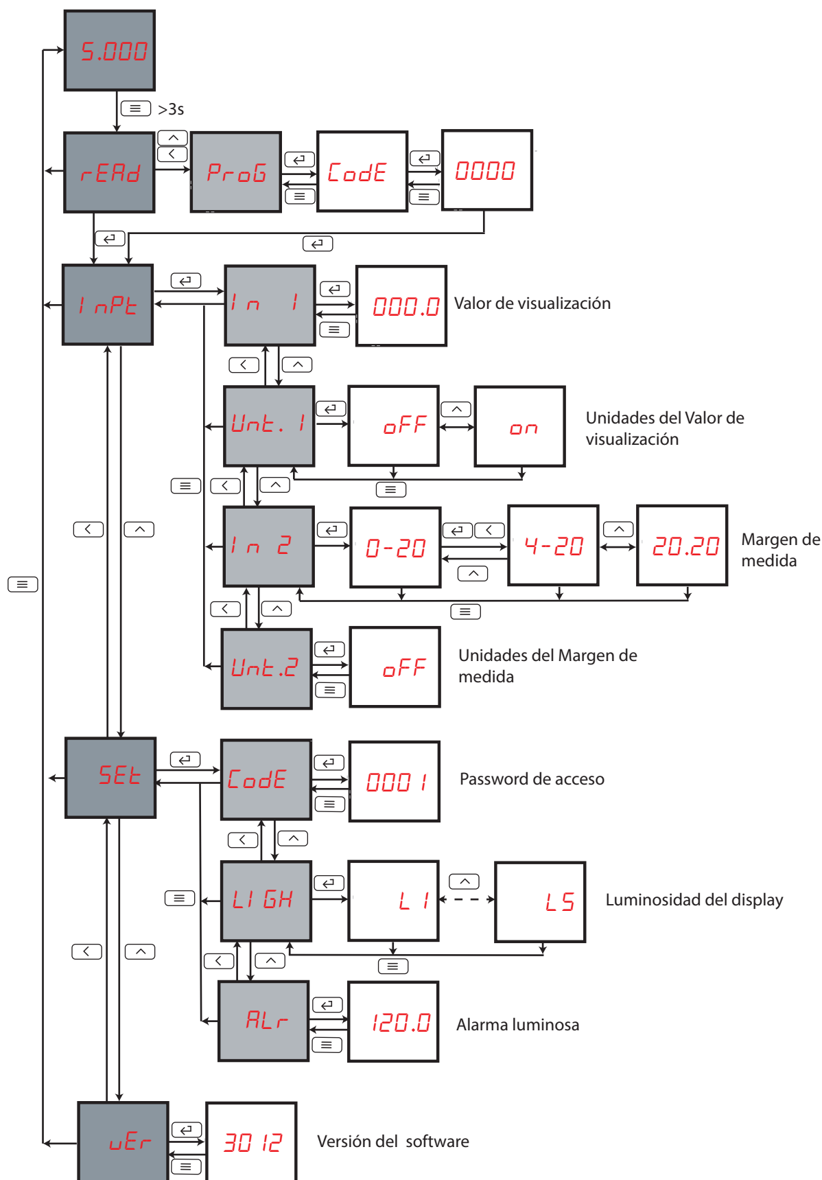
Figura 17: Menú de configuración DCB-72 mAdc
