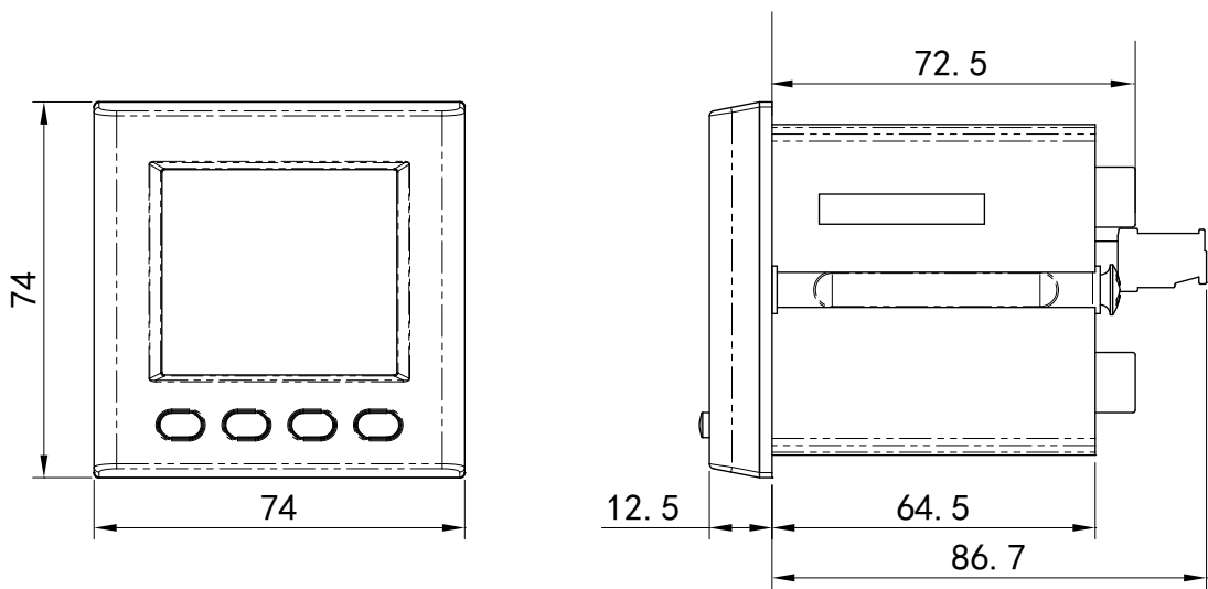
Figura 16: Dimensiones DCB-72 Adc.
