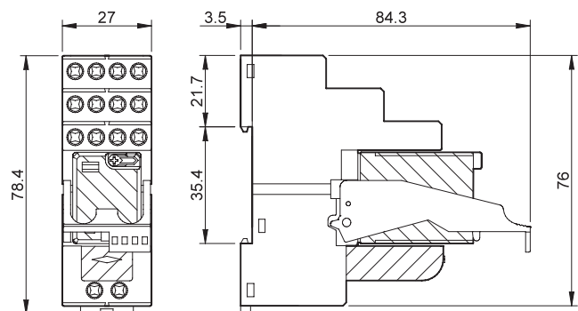
Tipo 58.P3 Bornes push-in
