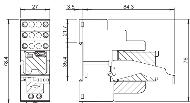
Tipo 58.34 Bornes de jaula
