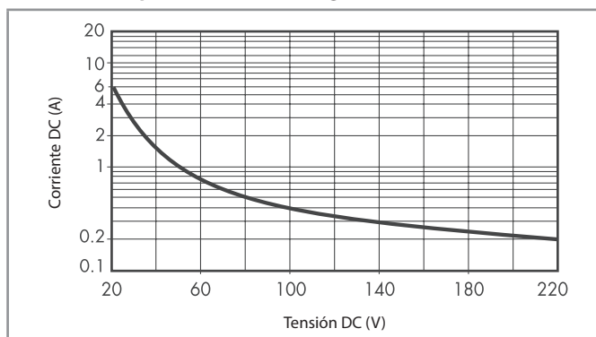
H 32 - Máximo poder de corte con cargas en DC1
