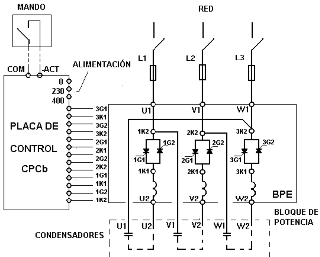
Figura 3.- Esquema de conexión
