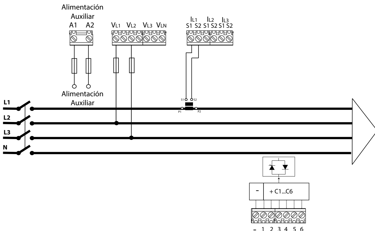
Figura 7: 2 tensiones y 1 corriente, modelo Computer SMART III 6 FAST 12Vdc.
