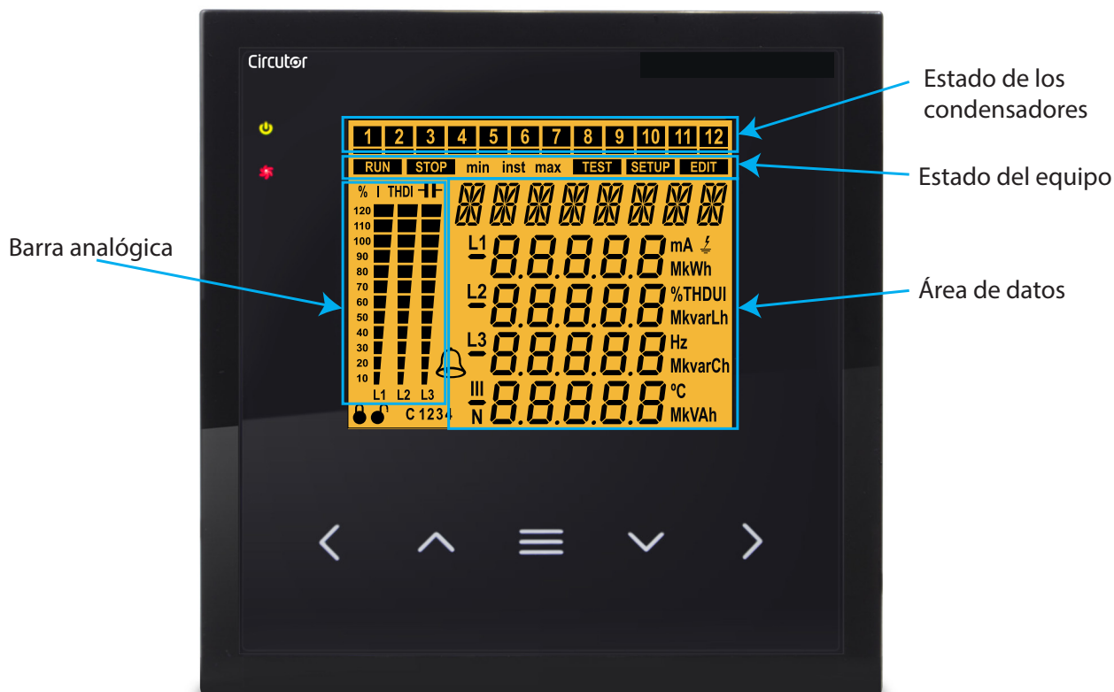
Figura 12: Áreas del display del Computer SMART III FAST 12Vdc.
