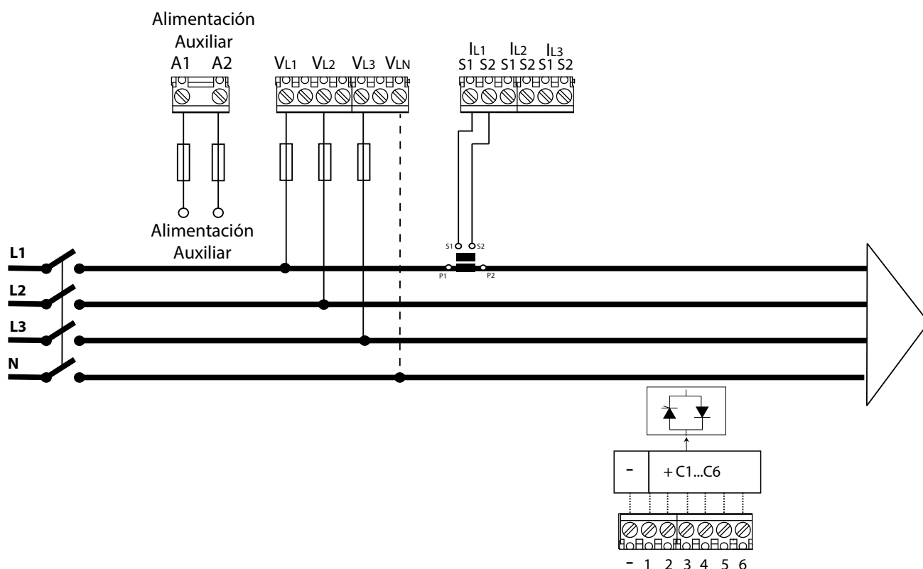
Figura 5: 3 tensiones + neutro y 1 corriente, modelo Computer SMART III 6 FAST 12Vdc.
