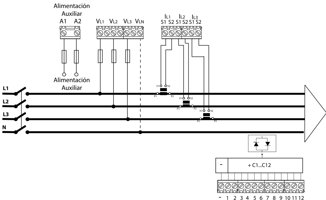
Figura 4: 3 tensiones + neutro y 3 corrientes, modelo Computer SMART III 12 FAST 12Vdc.
