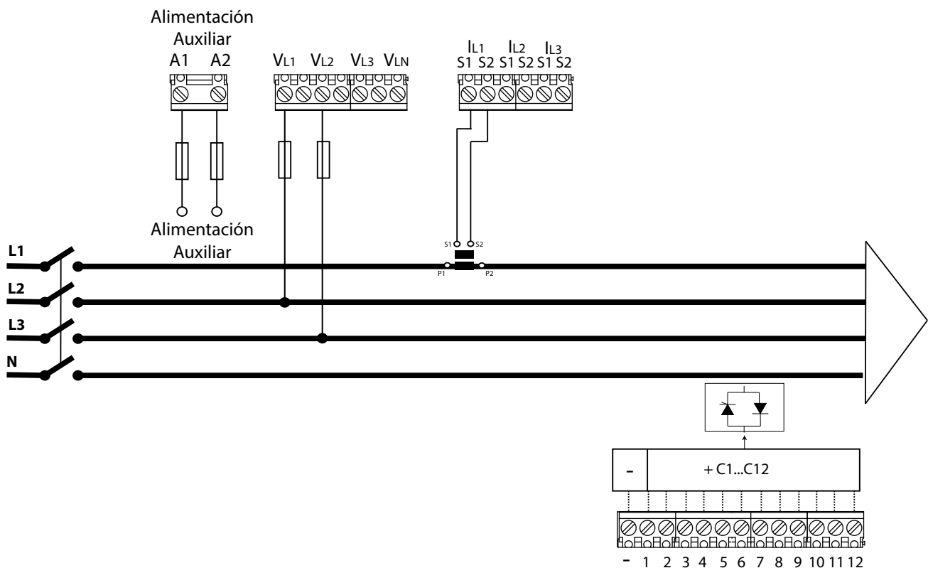
Figura 8: 2 tensiones y 1 corriente, modelo Computer SMART III 12 FAST 12Vdc.
