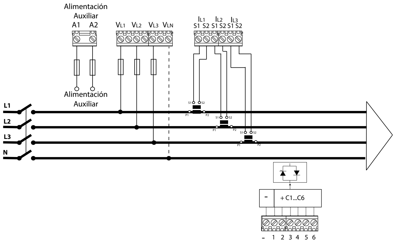
Figura 3: 3 tensiones + neutro y 3 corrientes, modelo Computer SMART III 6 FAST 12Vdc.
