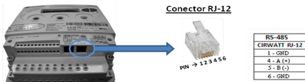
Figura 6: Conector RS-485
