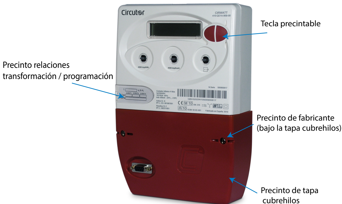
Figura 2:Precintos.
