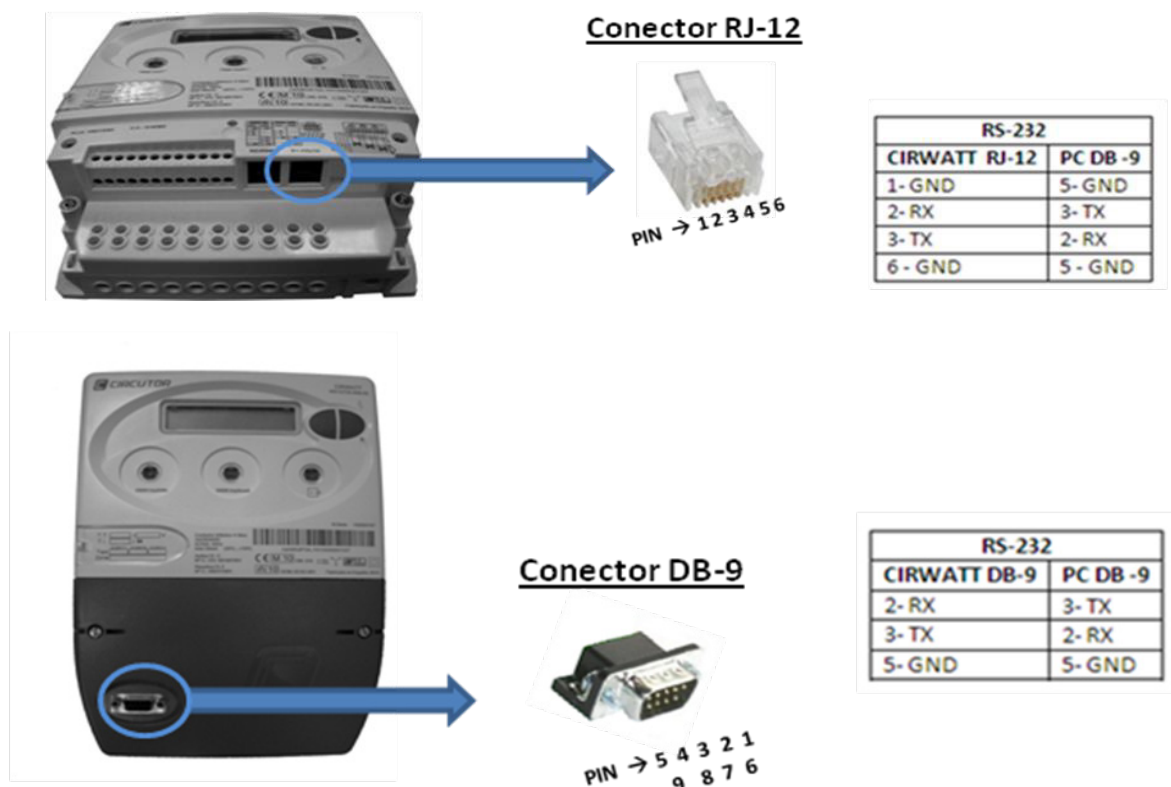
Figura 5: Conectores RS-232.
