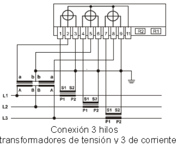
Figura 14: Conexión indirecta.
