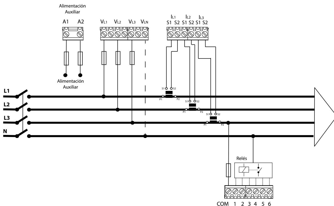
Figura 3: 3 tensiones + neutro y 3 corrientes, modelo Computer SMART III 6.
