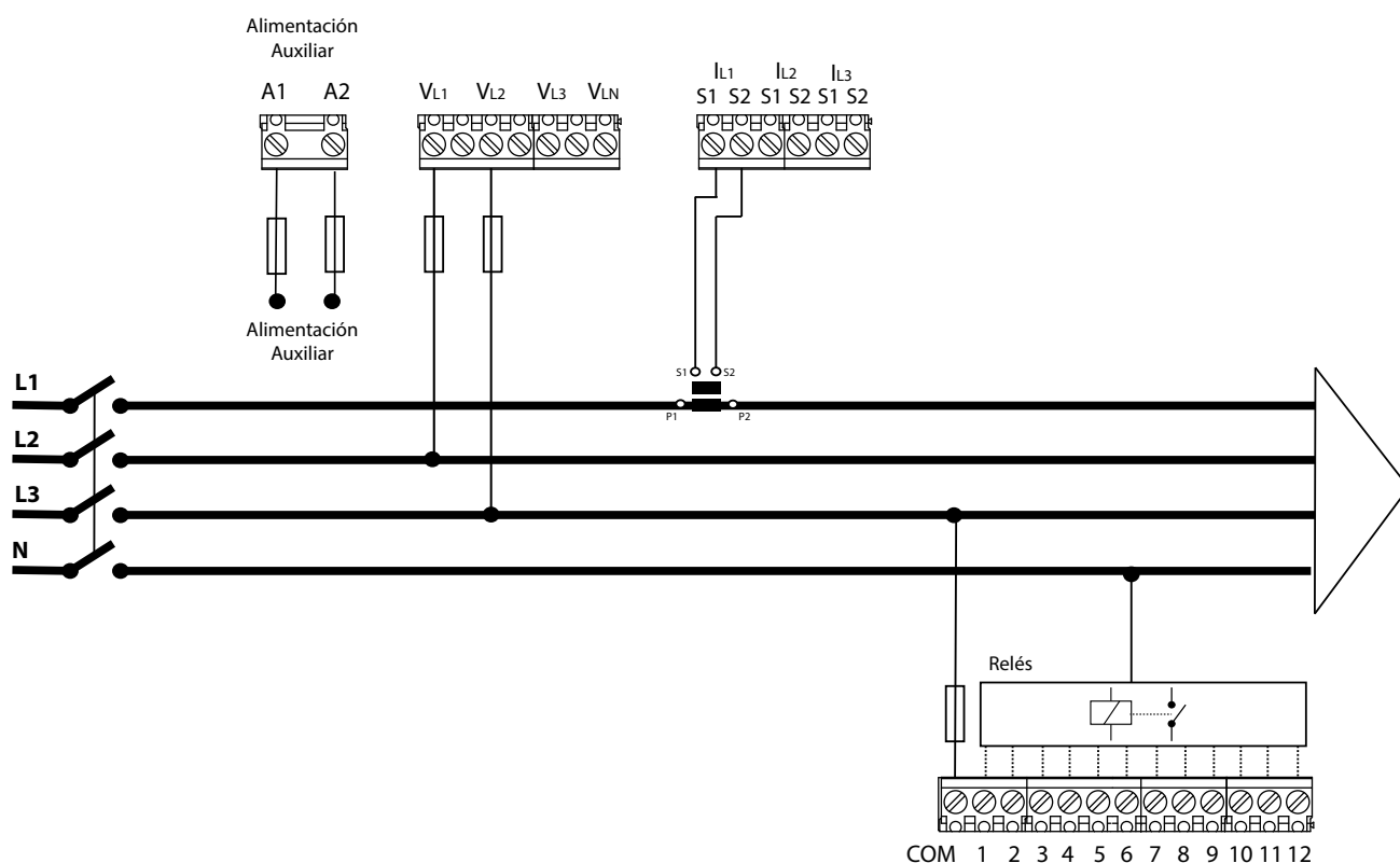
Figura 10: 2 tensiones y 1 corriente, modelo Computer SMART III 12.
