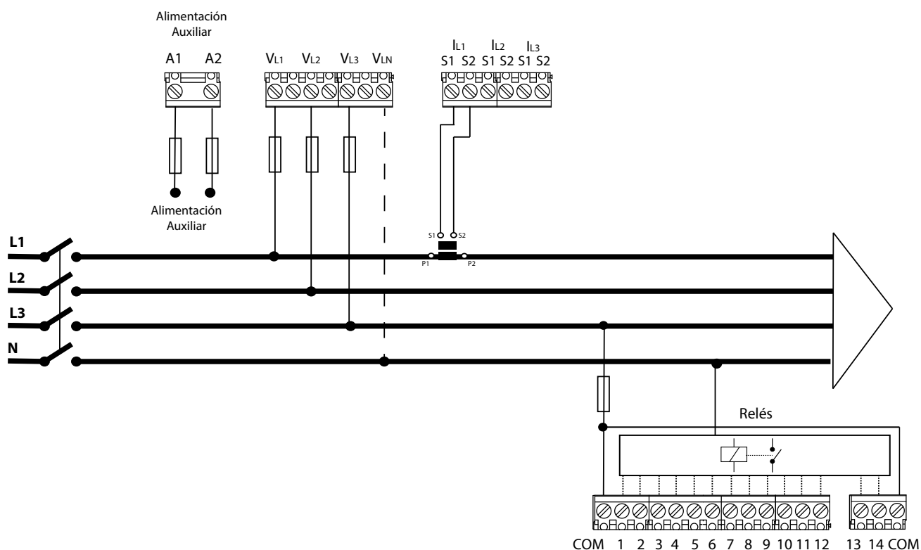
Figura 8: 3 tensiones + neutro y 1 corriente, modelo Computer SMART III 14.
