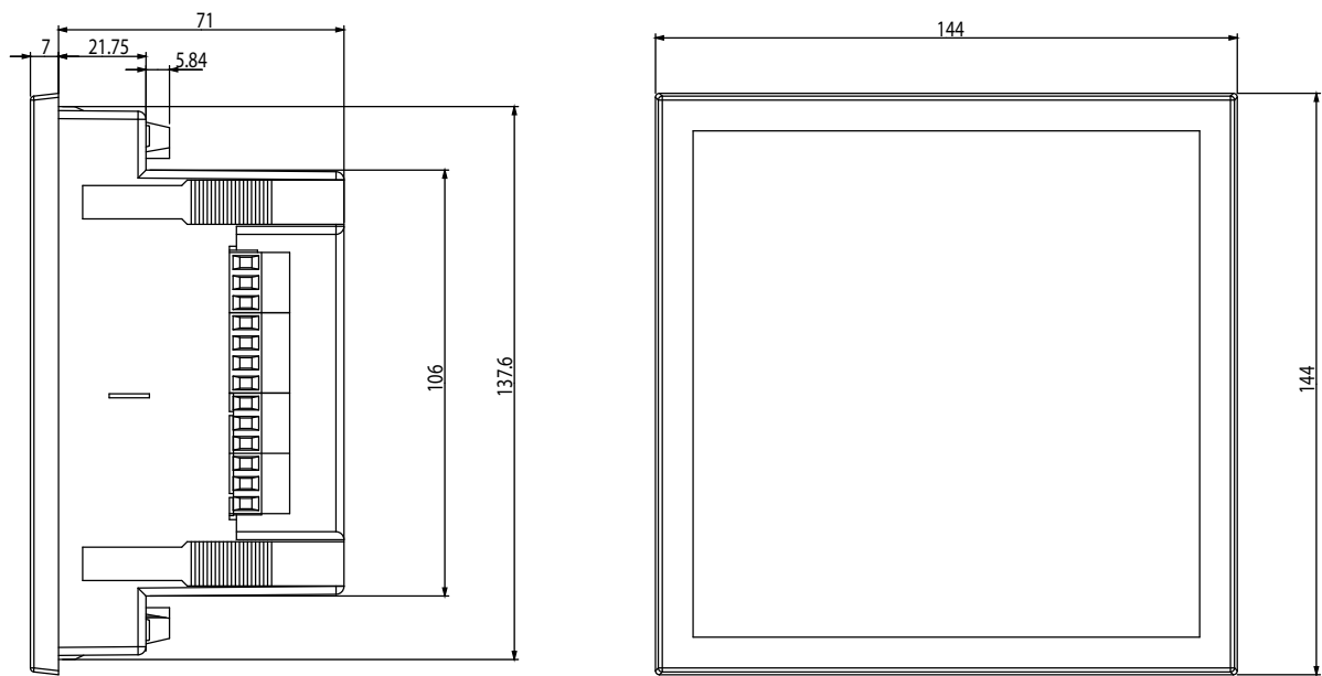
Figura 21: Dimensiones del Computer SMART III
