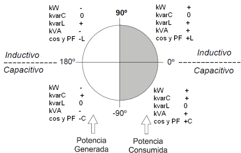
Figura 20: Esquema de los cuatro cuadrantes de medida y compensación.
