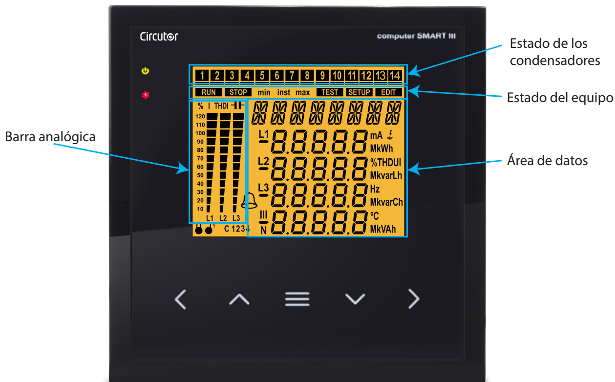
Figura 15: Áreas del display del Computer SMART III.
