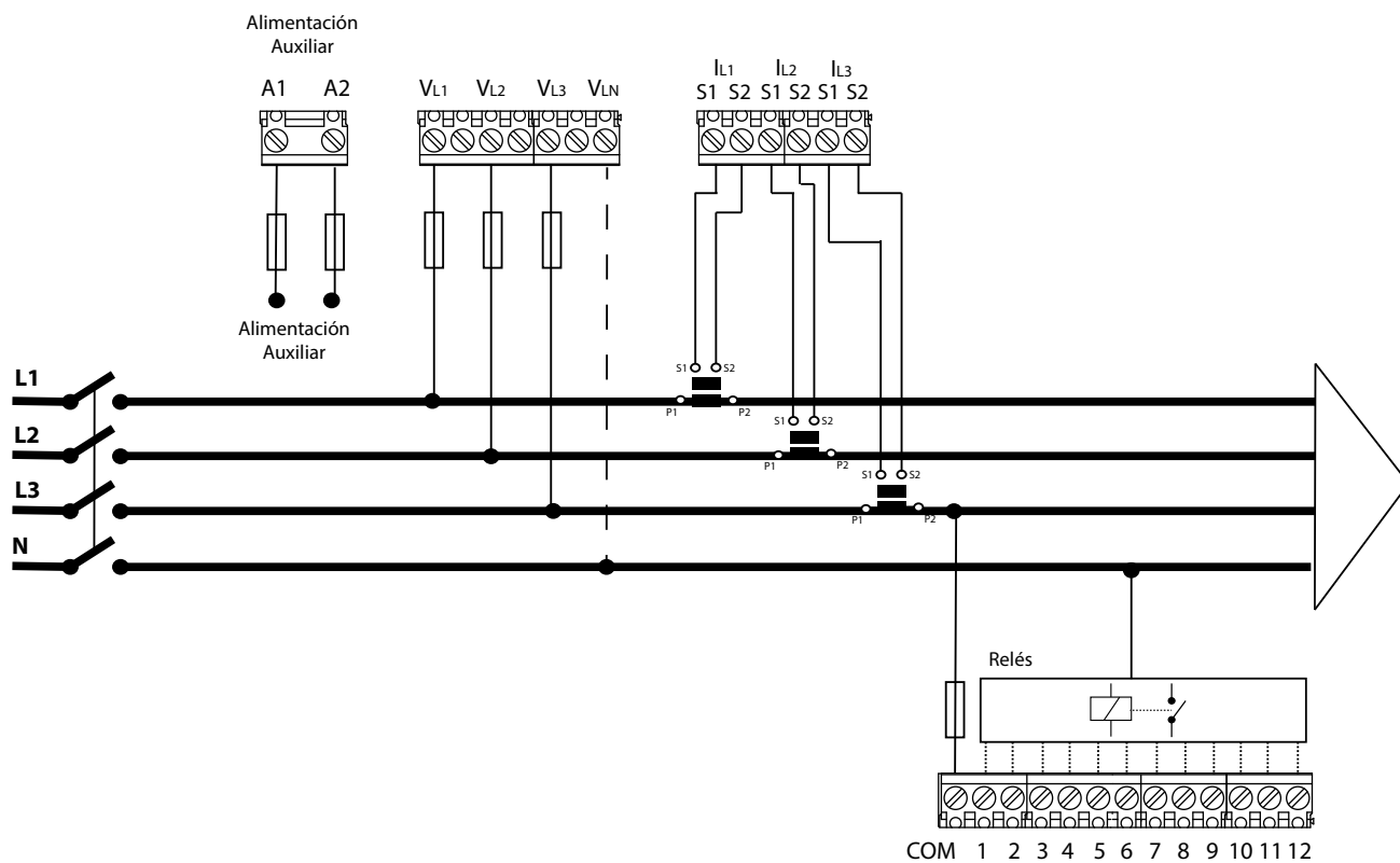
Figura 4: 3 tensiones + neutro y 3 corrientes, modelo Computer SMART III 12.
