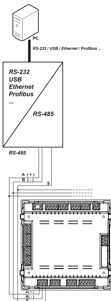
Figura 19: Esquema de conexionado RS-485
