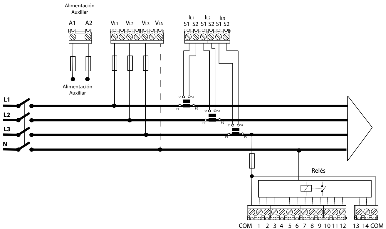
Figura 5: 3 tensiones + neutro y 3 corrientes, modelo Computer SMART III 14.
