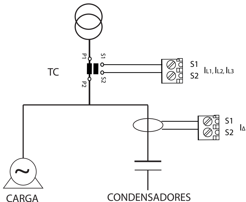
Figura 12: Conexión del transformador de corriente de fugas ( I_{\Delta} ).
