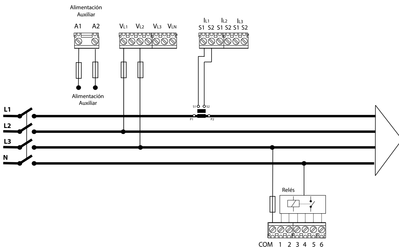
Figura 9: 2 tensiones y 1 corriente, modelo Computer SMART III 6.
