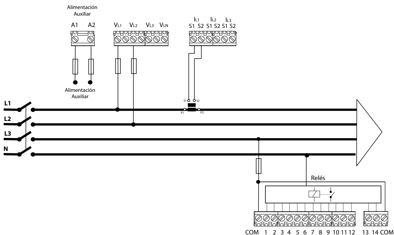
Figura 11: 2 tensiones y 1 corriente, modelo Computer SMART III 14.
