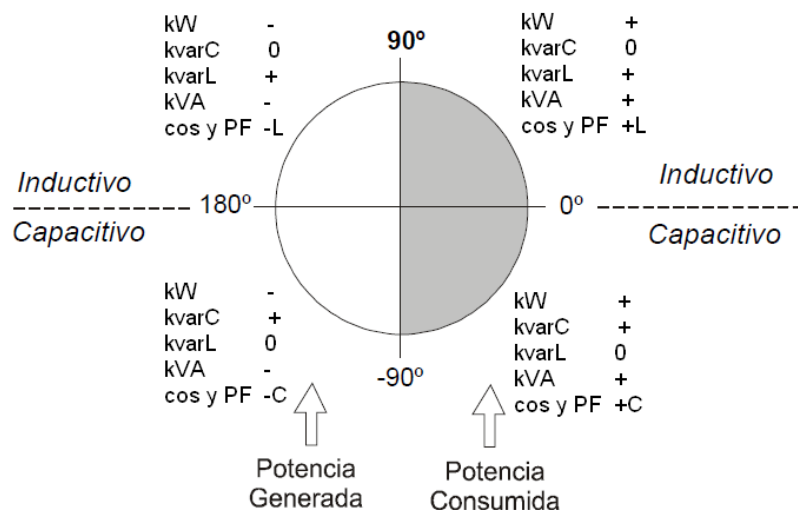
Figura 14: Medida y Compensación en los 4 cuadrantes.
