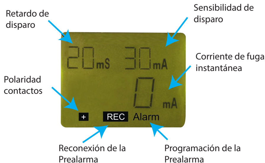
Figura 11: Descripción display.
