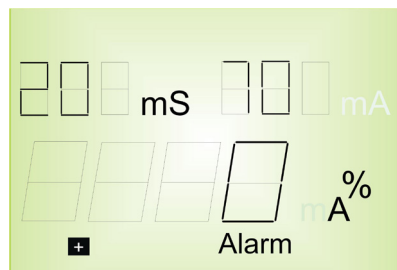
Figura 20: Ajuste de la seguridad positiva de prealarma.
