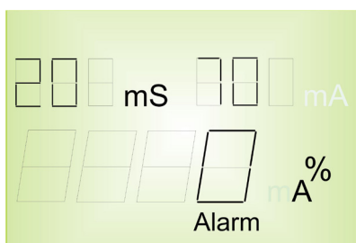
Figura 17: Ajuste del relé de prealarma.
