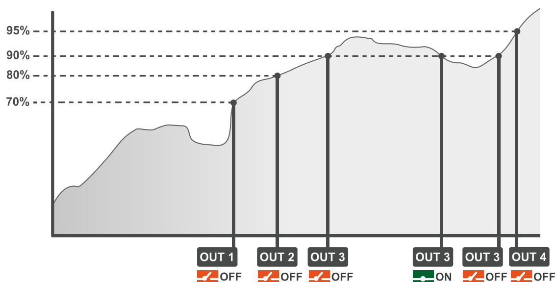
Figura 6: Gráfica con la respuesta del MDC-4
