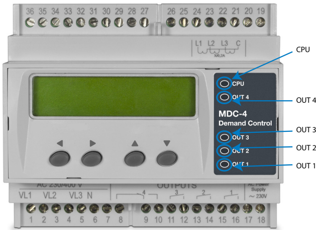
Figura 7: Indicadores LED.
