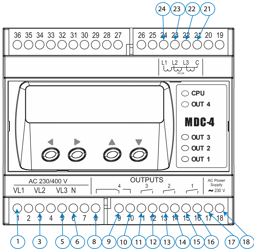
Figura 1: Bornes del MDC-4.
