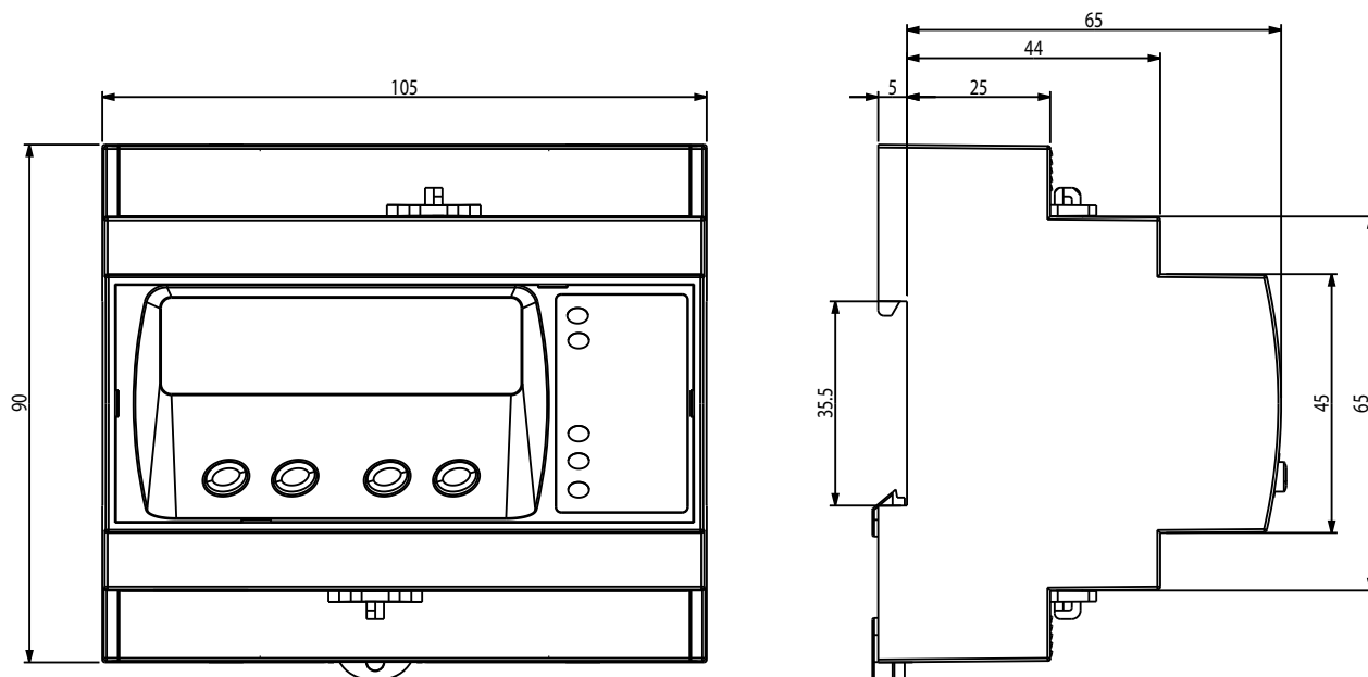
Figura 8: Dimensiones del MDC-4.
