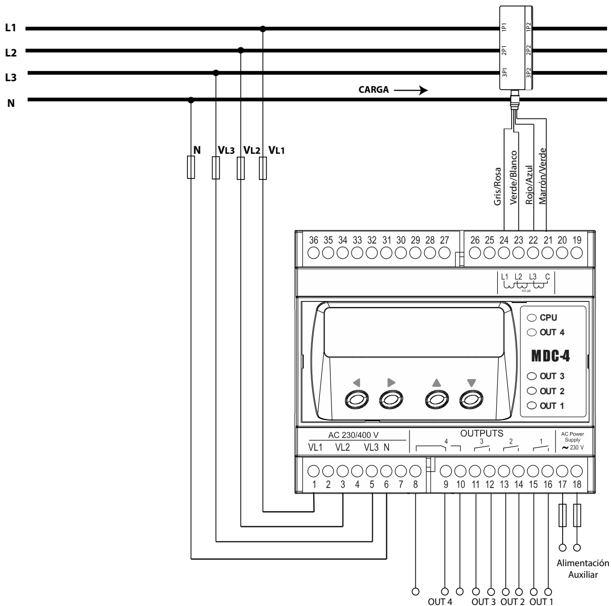
Figura 2: Medida de Red trifásica con conexión a 4 hilos.
