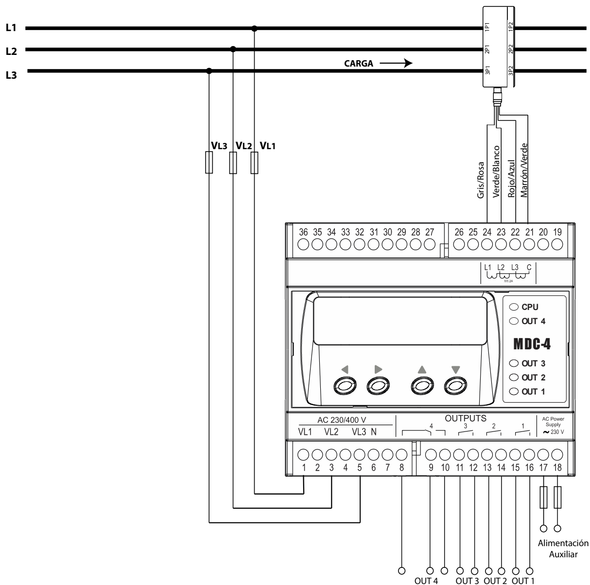
Figura 3: Medida de Red trifásica con conexión a 3 hilos.
