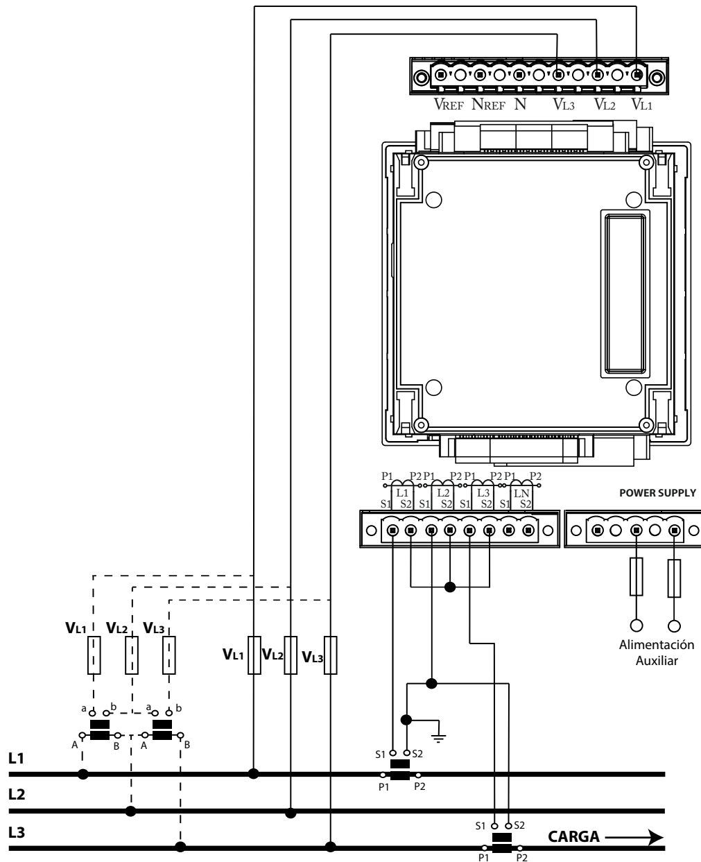
Figura 8: Medida trifásica con conexión a 3 hilos y transformadores en conexión ARON (Secundario del transformador: /1A, /5A o MC1 (/0.250)).
