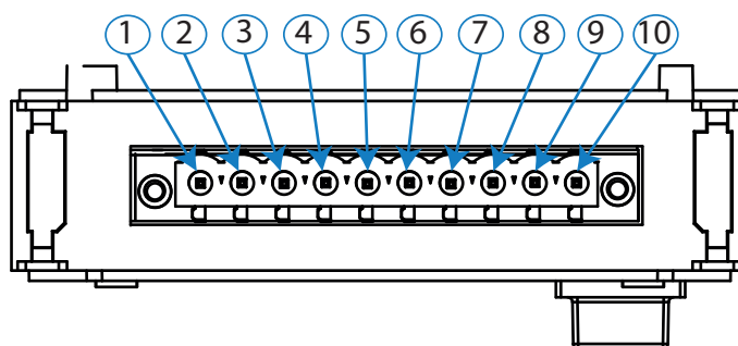
Figura 261: Bornes Entradas/Salidas digitales de Relé, cara superior.
