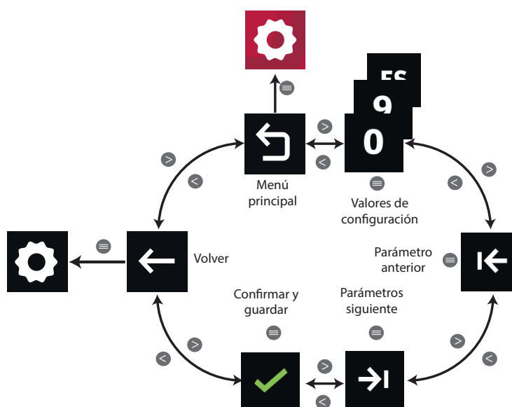
Figura 207: Menú configuración : Clave de acceso.
