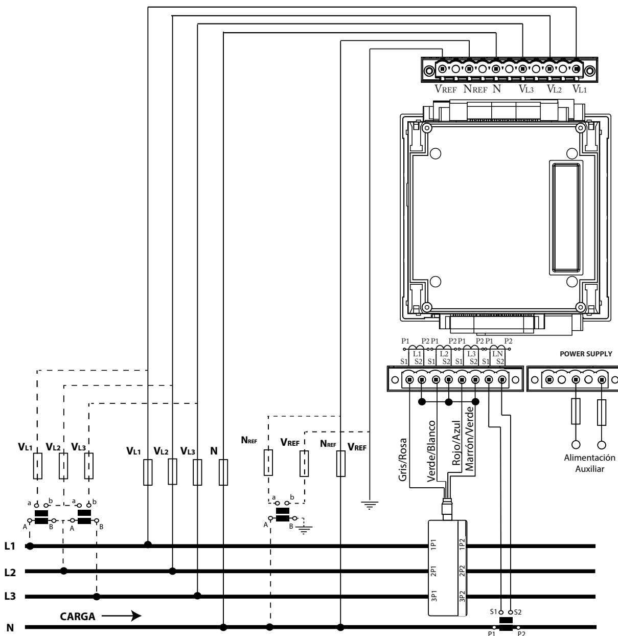
Figura 4: Medida trifásica con conexión a 4 hilos (Transformador tipo MC3 (/0.250)).
