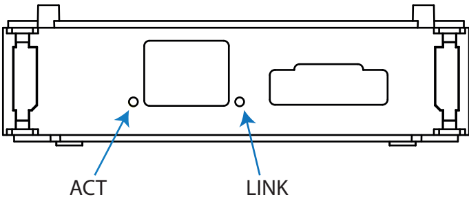
Figura 326: LEDs Modbus Datalogger.
