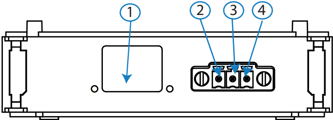
Figura 296: Bornes Módulo de comunicaciones Modbus TCP (Bridge)
