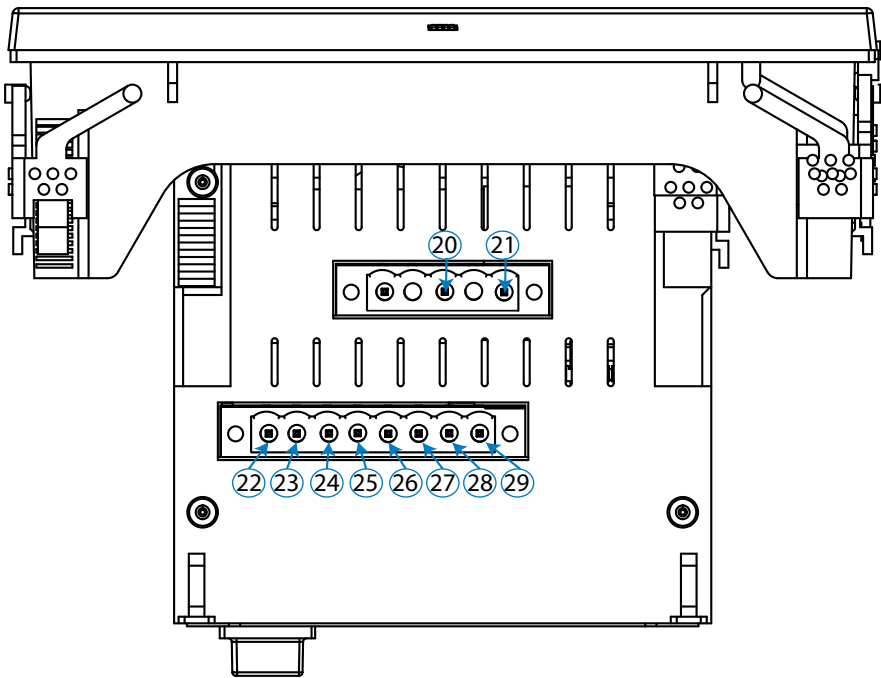
Figura 2: Bornes del CVM-B, cara inferior.
