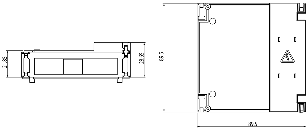
Figura 354: Dimensiones módulo de expansión (Tapa protectora versión 2).
