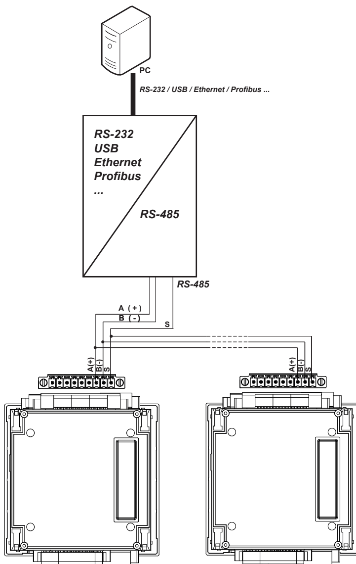
Figura 253: Esquema de conexionado RS-485.
