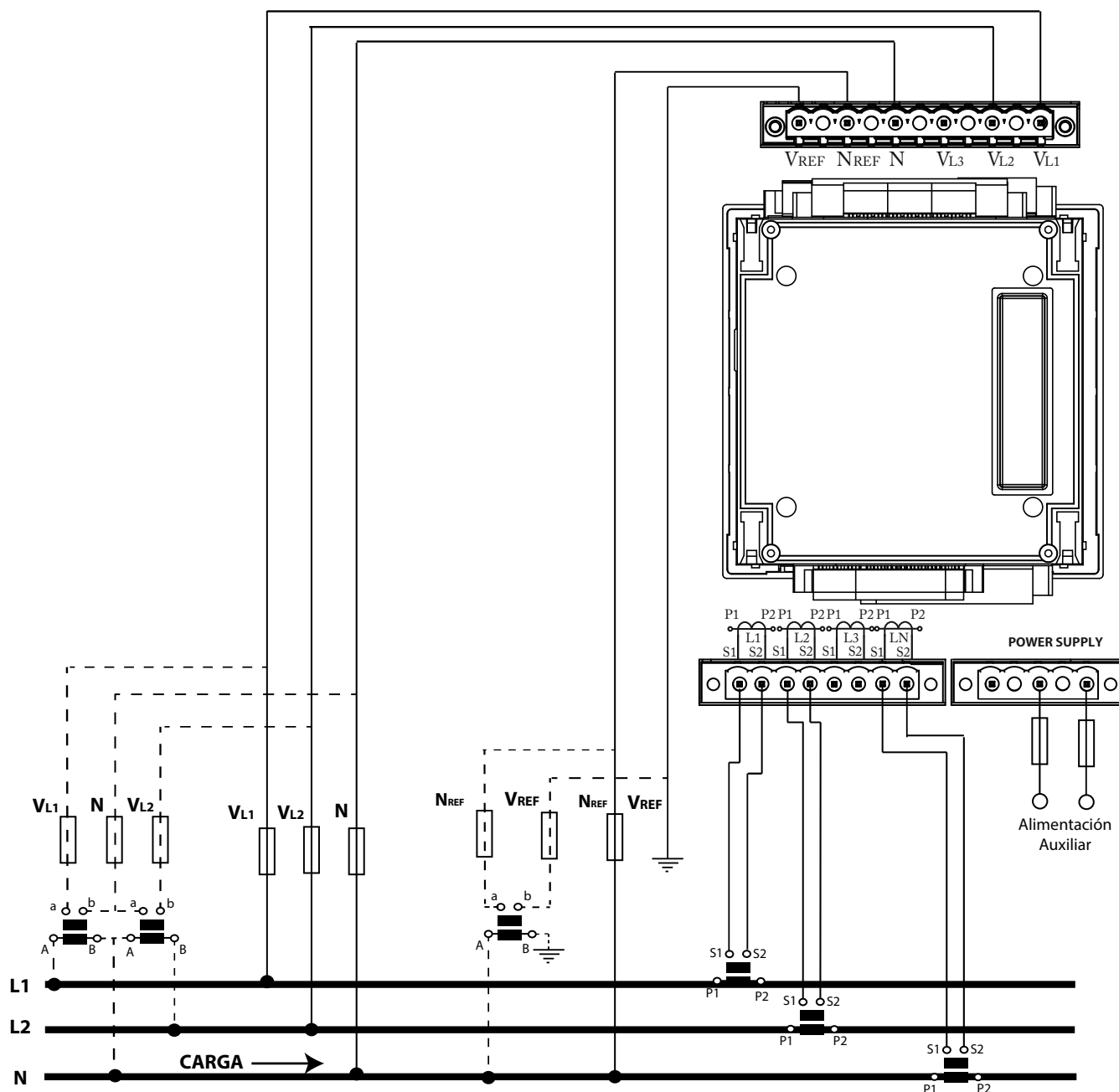
Figura 9: Medida bifásica con conexión a 3 hilos (Secundario del transformador: /1A, /5A o MC1 (/0.250)).
