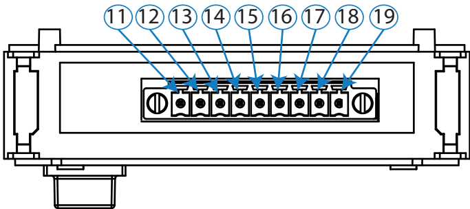
Figura 273:Bornes Entradas/Salidas digitales de Transistor, cara inferior.
