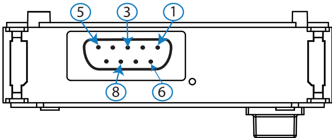
Figura 314: Bornes Módulo de comunicaciones Profibus.
