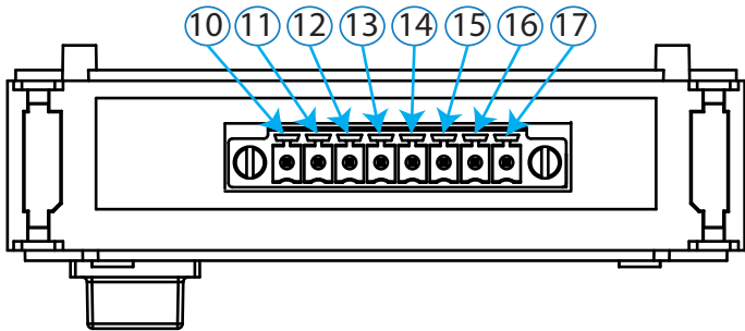
Figura 282:Bornes Entradas/Salidas analógicas, cara inferior.
