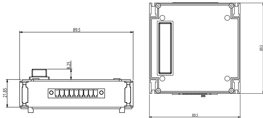
Figura 353: Dimensiones módulo de expansión (Tapa protectora versión 1).
