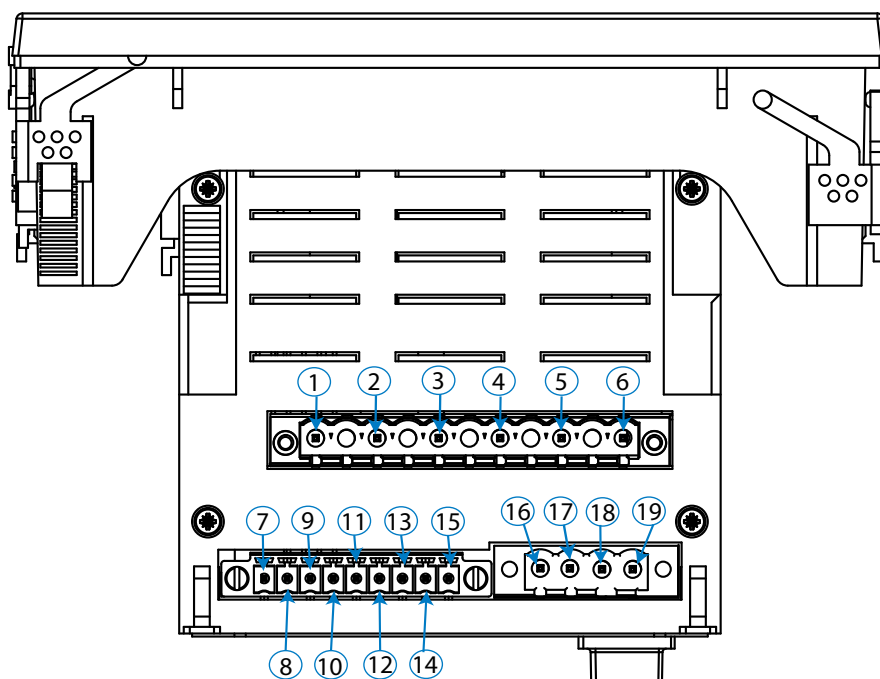
Figura 1: Bornes CVM-Bx, cara superior.
