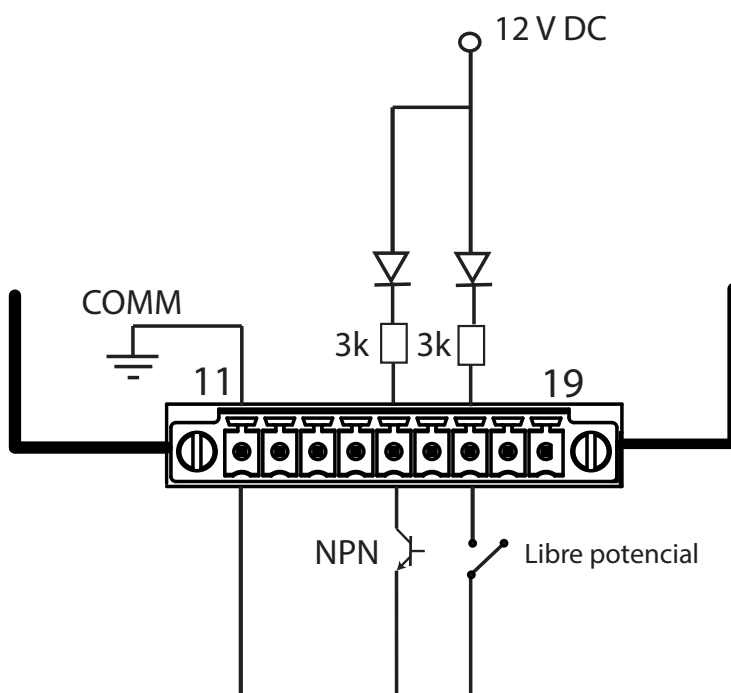
Figura 264: Esquema de conexionado, entradas digitales.
