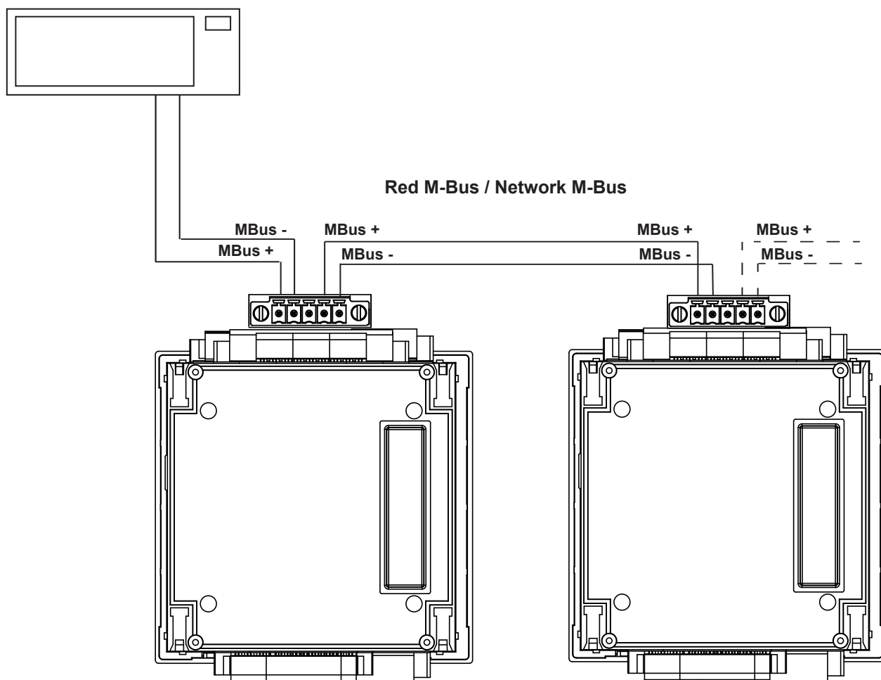
Figura 321: Esquema de conexión, MBus.
