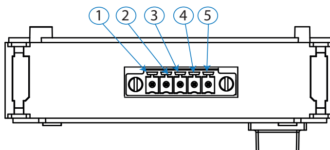
Figura 308: Bornes Módulo de comunicaciones LonWorks.
