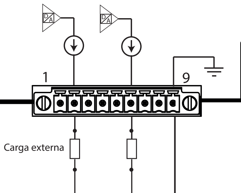
Figura 283: Esquema de conexionado, salidas analógicas.
