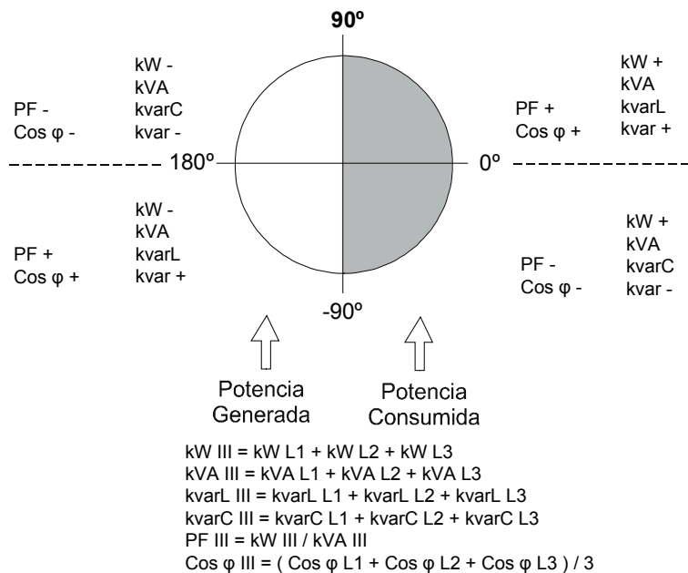
Figura 23: Cuatro cuadrantes de CVM-B.
