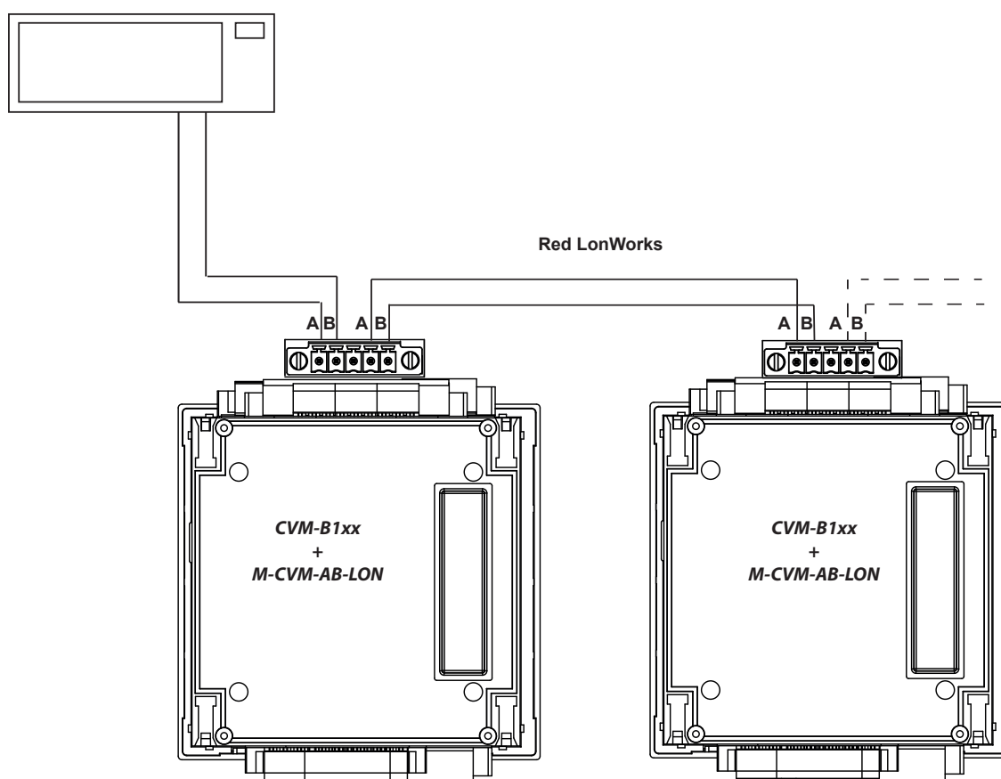
Figura 309: Esquema de conexión, LonWorks.
