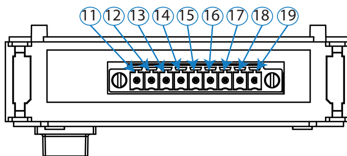
Figura 262: Bornes Entradas/Salidas digitales de Relé, cara inferior.
