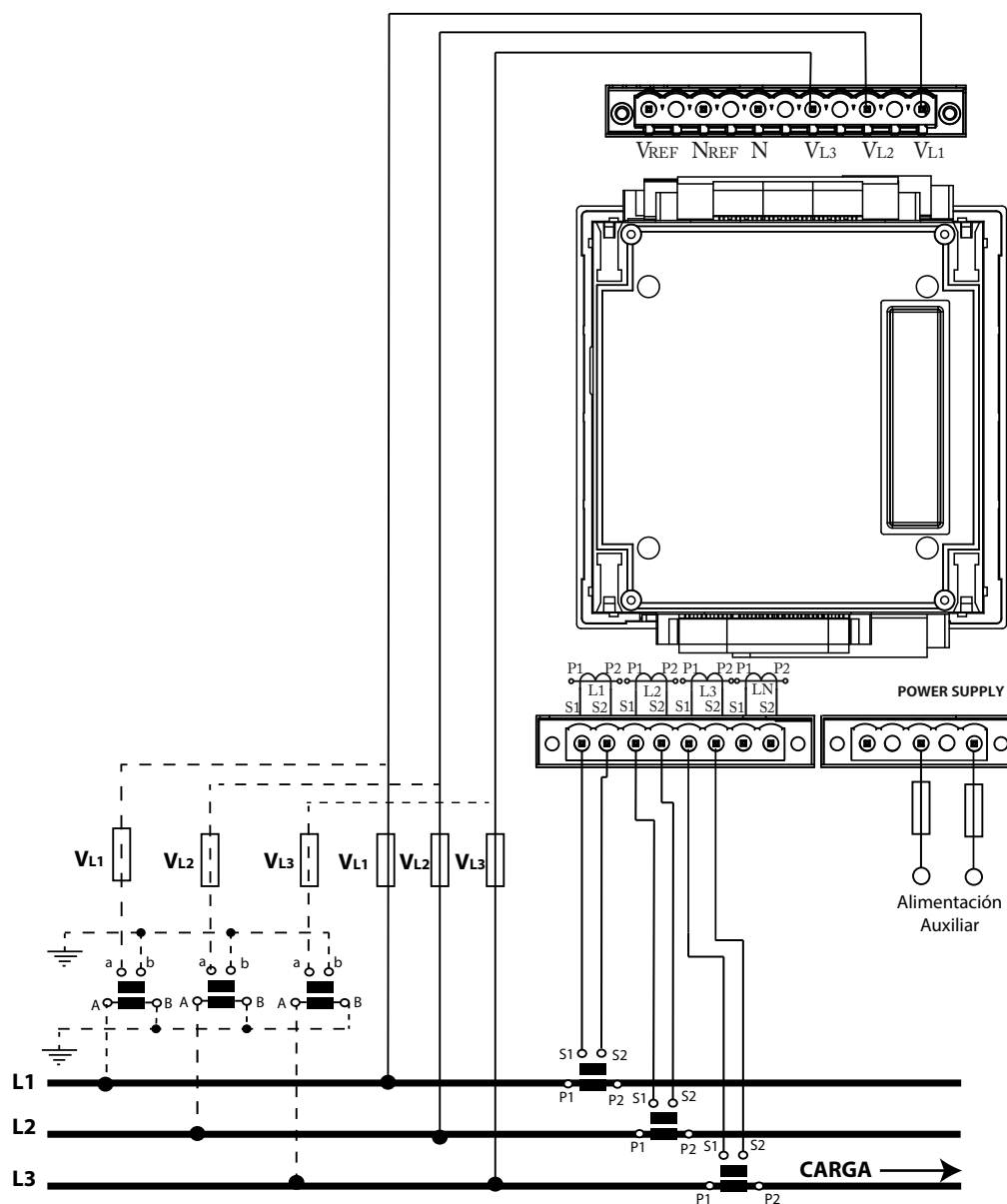
Figura 7: Medida trifásica con conexión a 3 hilos y 3 transformadores de tensión (Secundario del transformador: /1A, /5A o MC1 (/0.250)).
