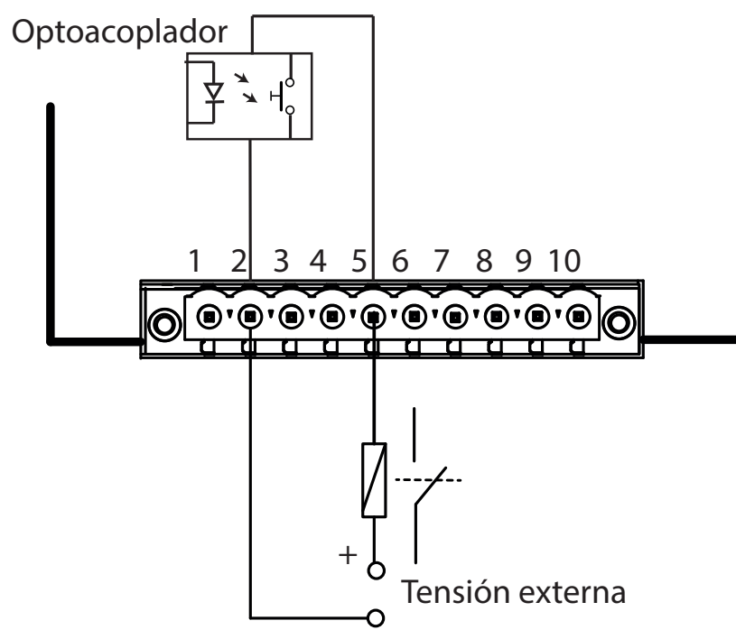
Figura 274: Esquema de conexionado, salida digitales de transistor.
