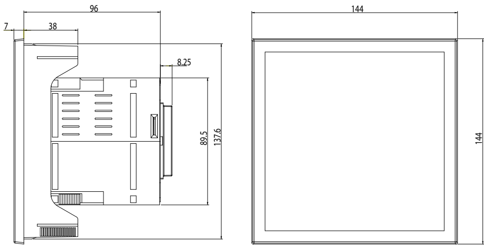
Figura 352:Dimensiones CVM-B150.
