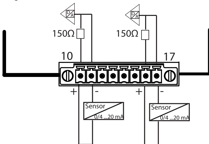
Figura 284: Esquema de conexionado, entradas analógicas.
