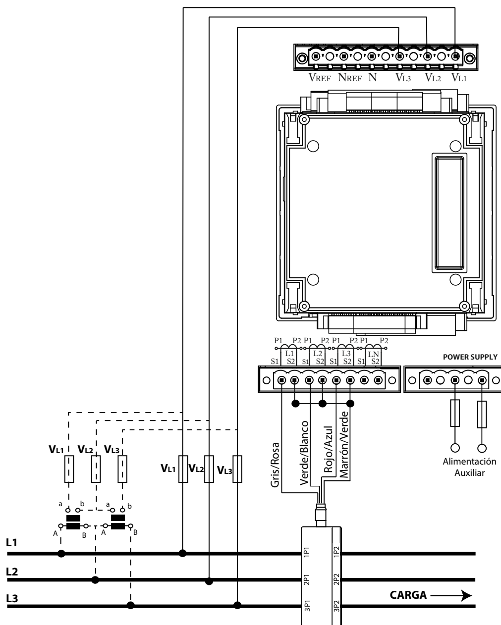
Figura 6: Medida trifásica con conexión a 3 hilos (Transformador tipo MC3 (/0.250)).
