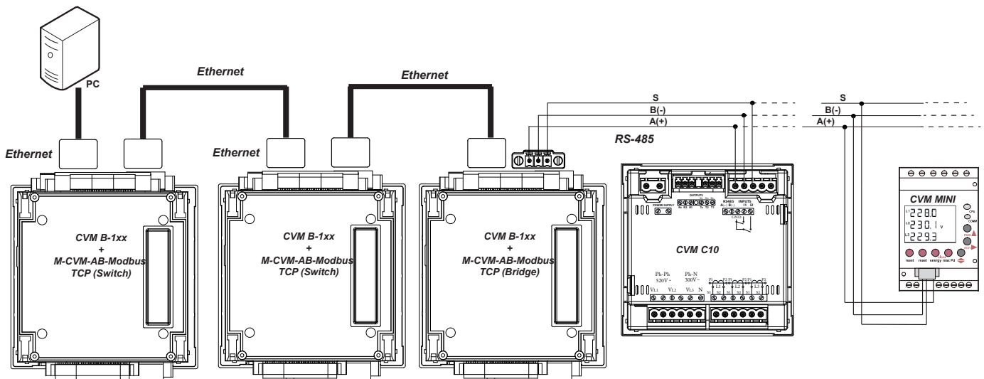
Figura 339: Esquema de conexionado, Modbus TCP (Switch).
