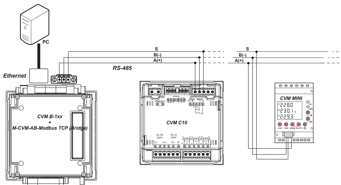
Figura 298: Esquema de conexión, Modbus TCP (Bridge).
