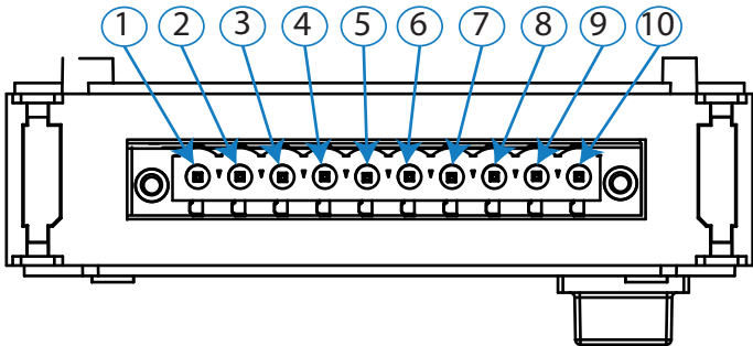
Figura 272: Bornes Entradas/Salidas digitales de Transistor, cara superior.
