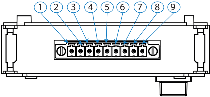
Figura 281:Bornes Entradas/Salidas analógicas, cara superior.
