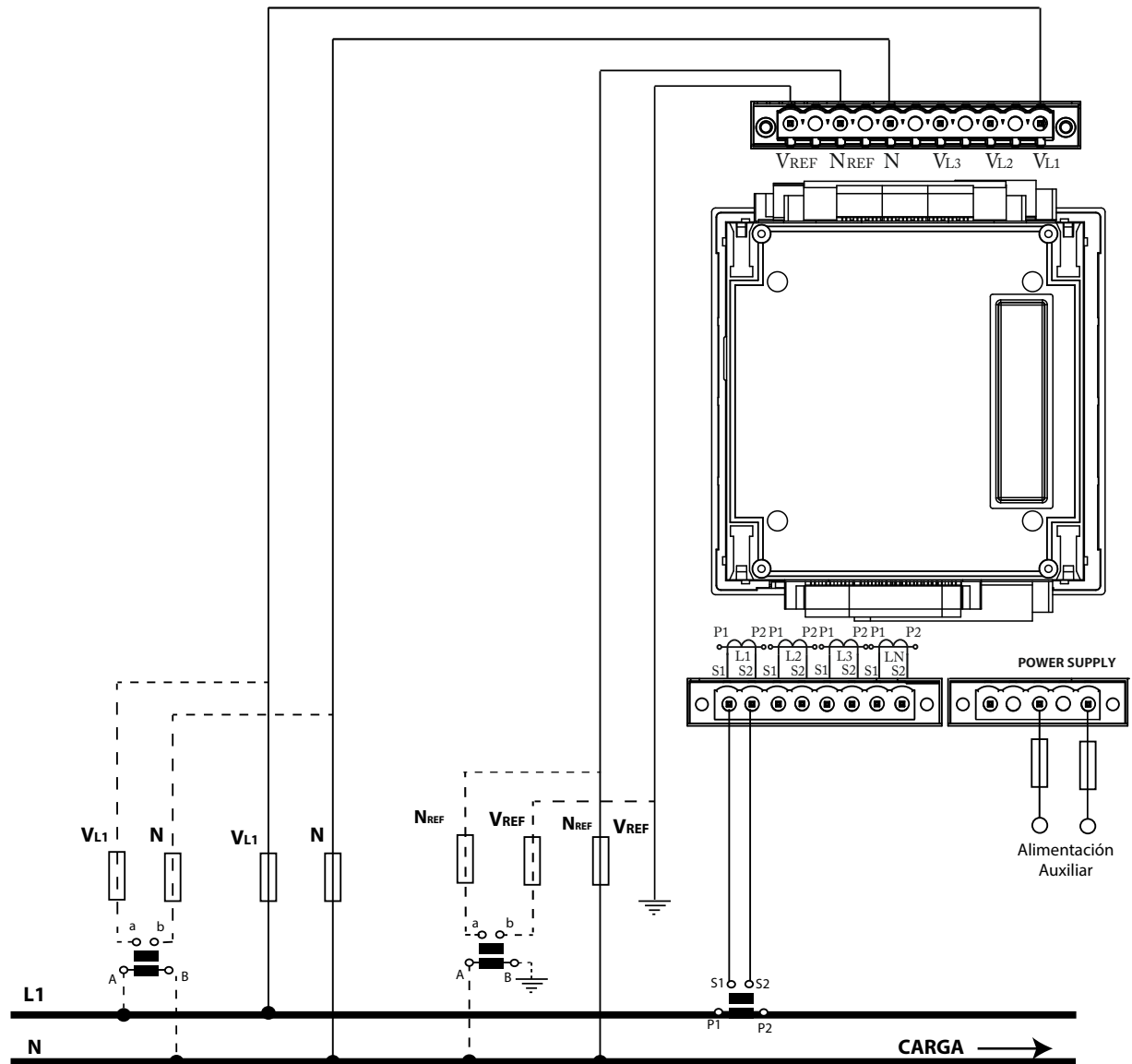
Figura 11: Medida monofásica de fase a neutro de 2 hilos (Secundario del transformador: /1A, /5A o MC1 (/0.250)).
