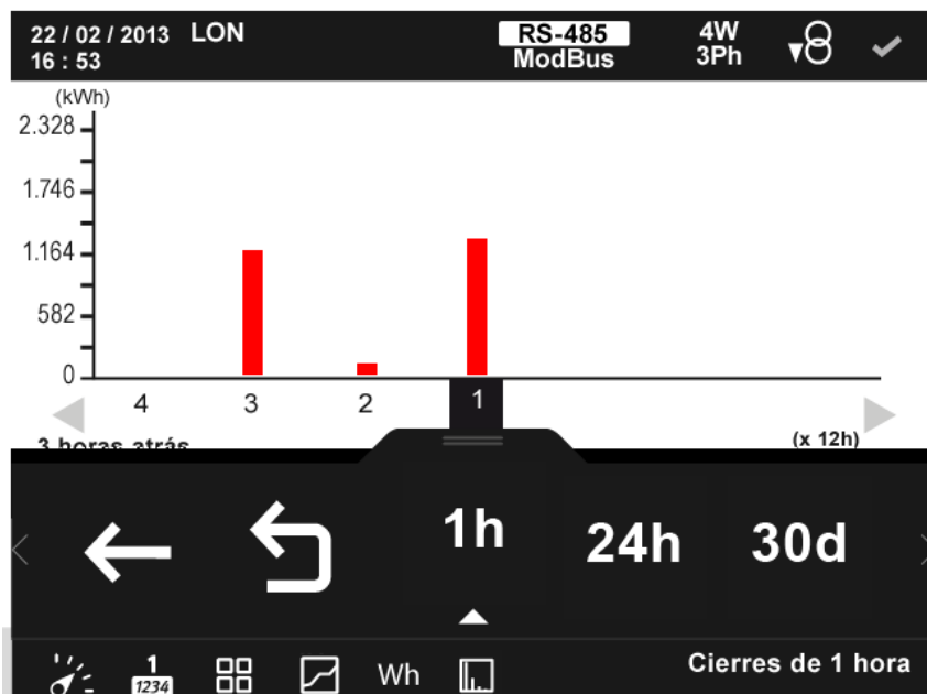
Figura 53: Parámetros incrementales, visualización gráfica (visualizar 1 parámetro).
