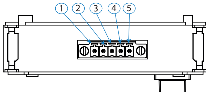
Figura 320: Bornes Módulo de comunicaciones MBus.
