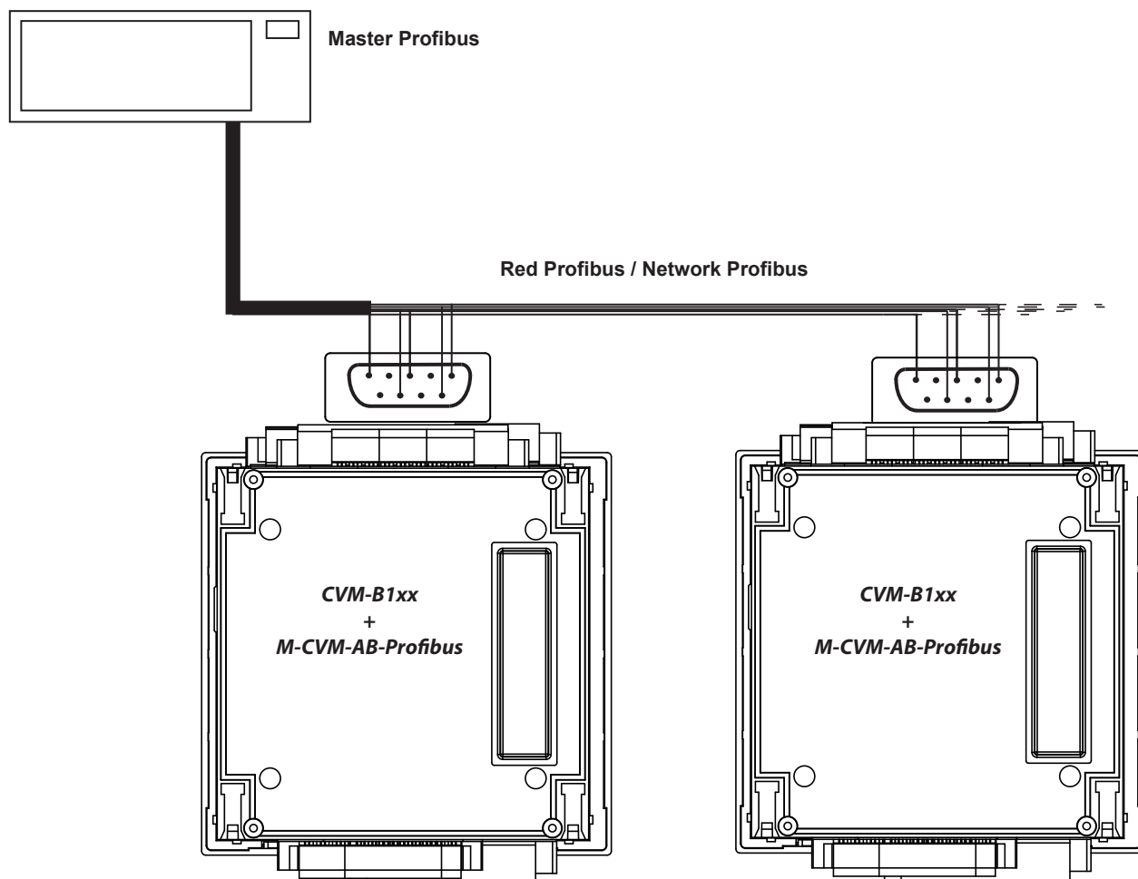
Figura 316:Esquema de conexionado, Profibus.
