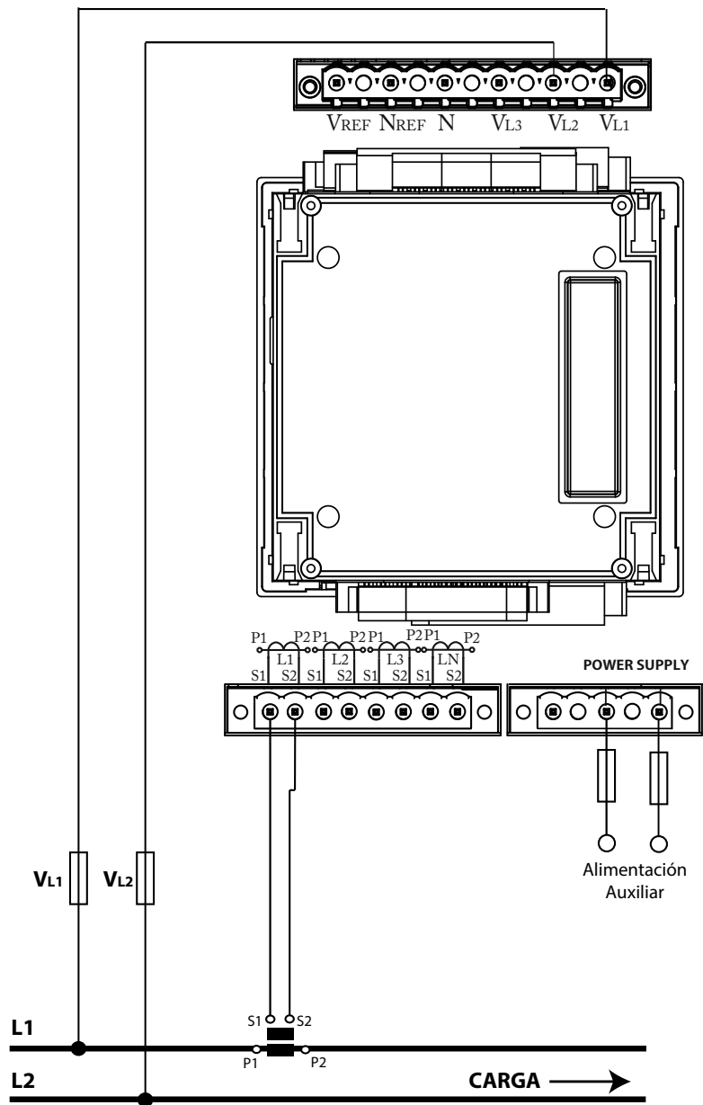
Figura 10: Medida monofásica de fase a fase de 2 hilos (Secundario del transformador: /1A, /5A o MC1 (/0.250)).
