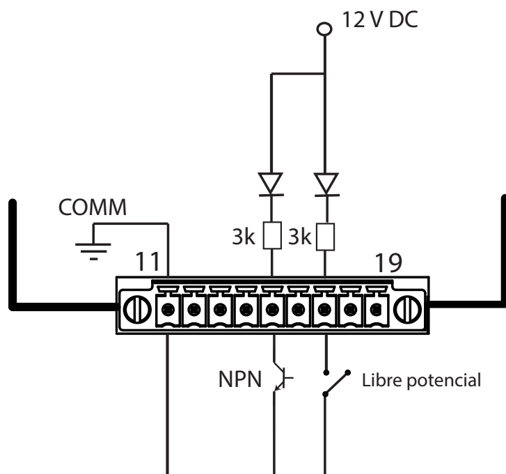
Figura 275: Esquema de conexionado, entradas digitales.
