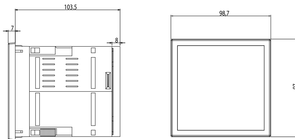
Figura 351: Dimensiones CVM-B100.
