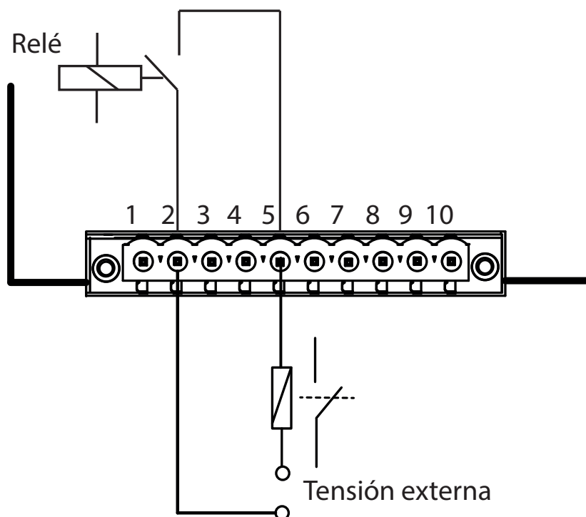
Figura 263: Esquema de conexionado, salida digitales de relé.
