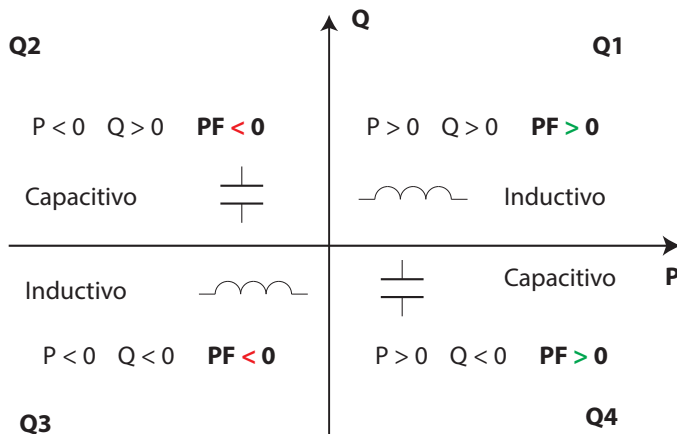
Figura 21: Convenio de medida IEC.
