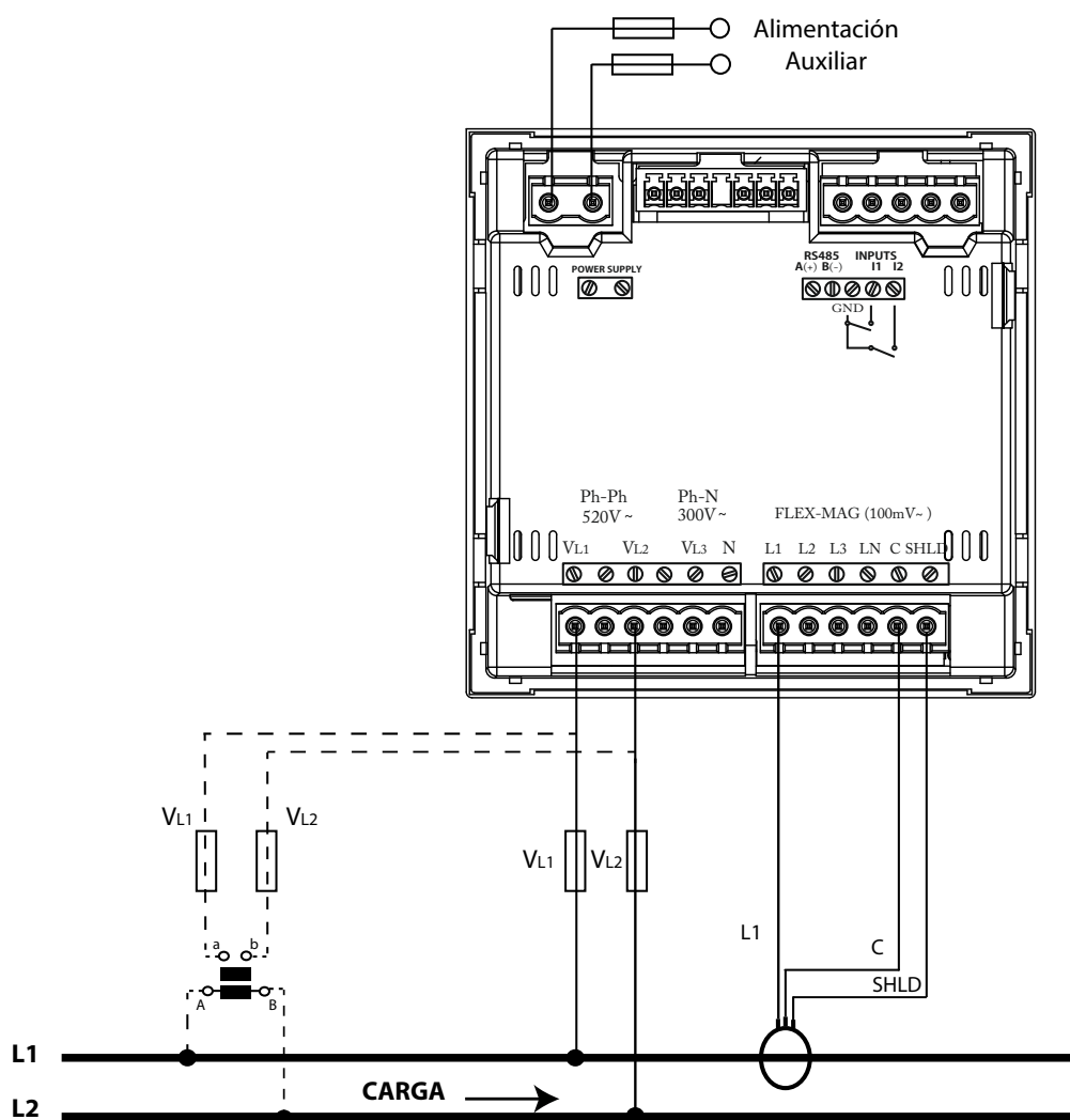
Figura 17: Medida monofásica de fase a fase de 2 hilos, modelos CVM-C10-FLEX.
