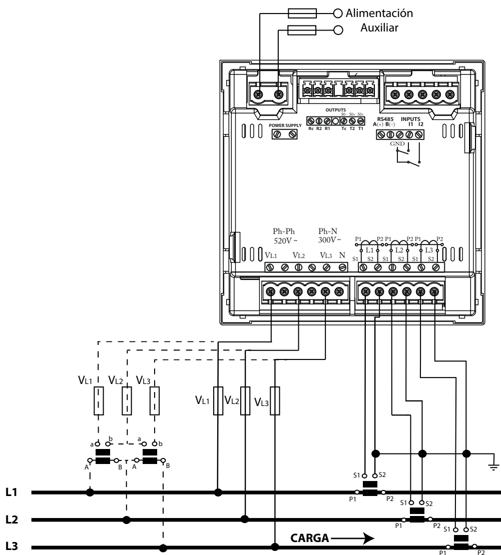
Figura 9: Medida trifásica con conexión a 3 hilos, modelos CVM-C10-ITF y CVM-C10-mV.
