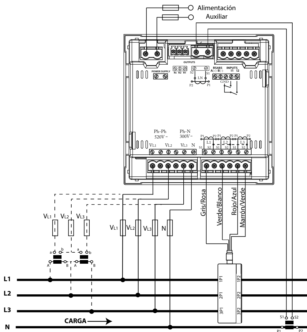
Figura 7: Medida trifásica con conexión a 4 hilos, modelo CVM-C10-MC-IN.
