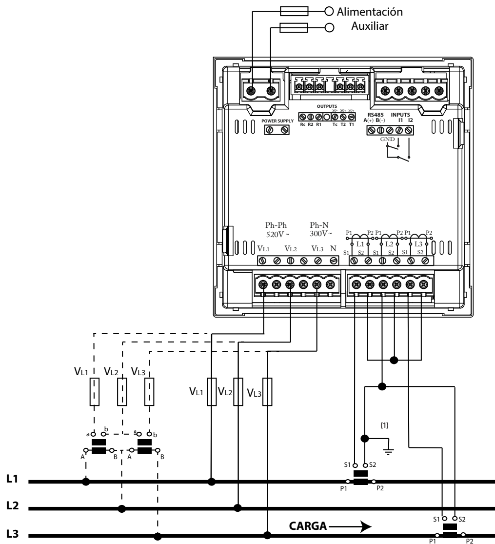
Figura 12: Medida trifásica con conexión a 3 hilos y transformadores en conexión ARON, modelos CVM-C10-ITF y CVM-C10-MC.
