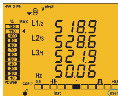
Figura 32: Pantalla del CVM-C10 con el perfil de funcionamiento user.
