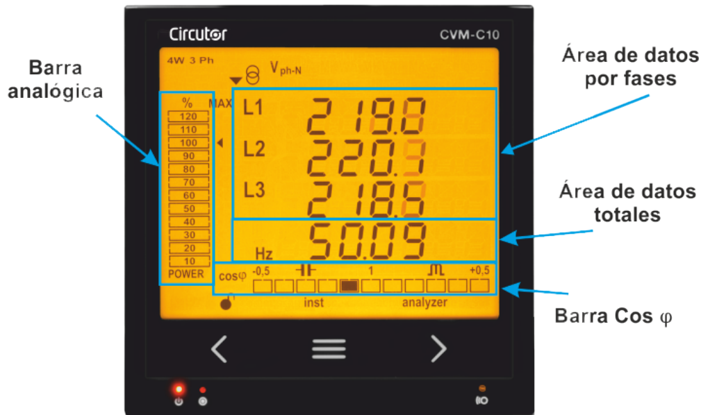
Figura 23: Áreas del display del CVM-C10
