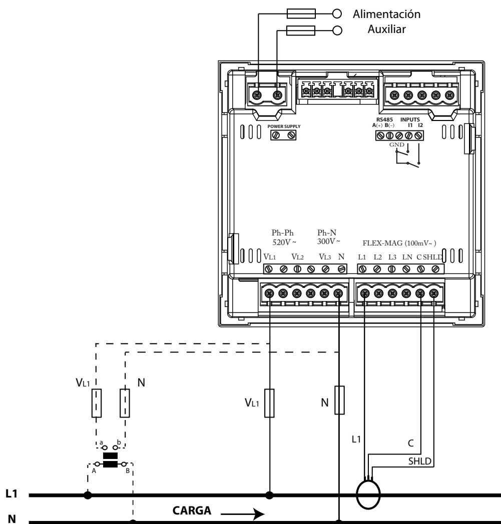
Figura 19: Medida monofásica de fase a neutro de 2 hilos, modelos CVM-C10-FLEX.
