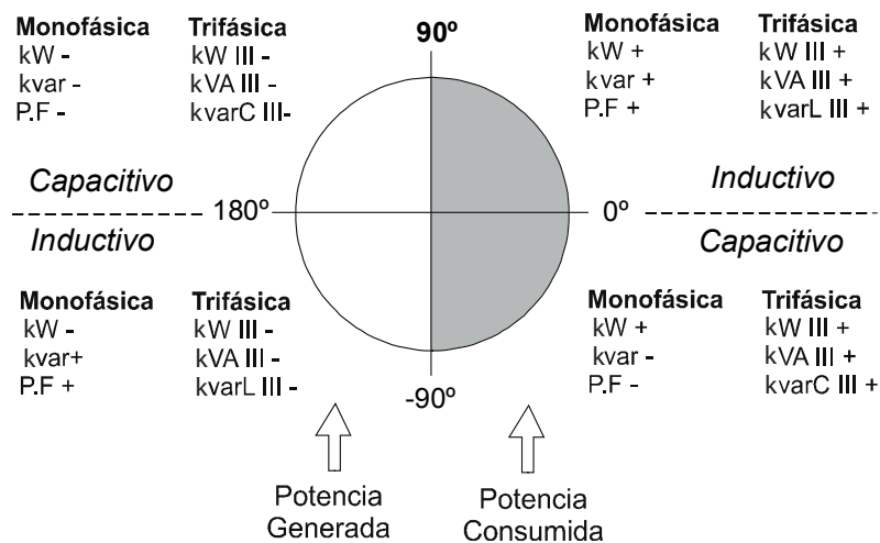
Figura 20: Convenio de medida CIRCUTOR
