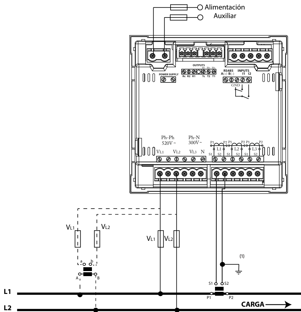
Figura 16: Medida monofásica de fase a fase de 2 hilos, modelos CVM-C10-ITF, CVM-C10-MC y CVM-C10-mV.
