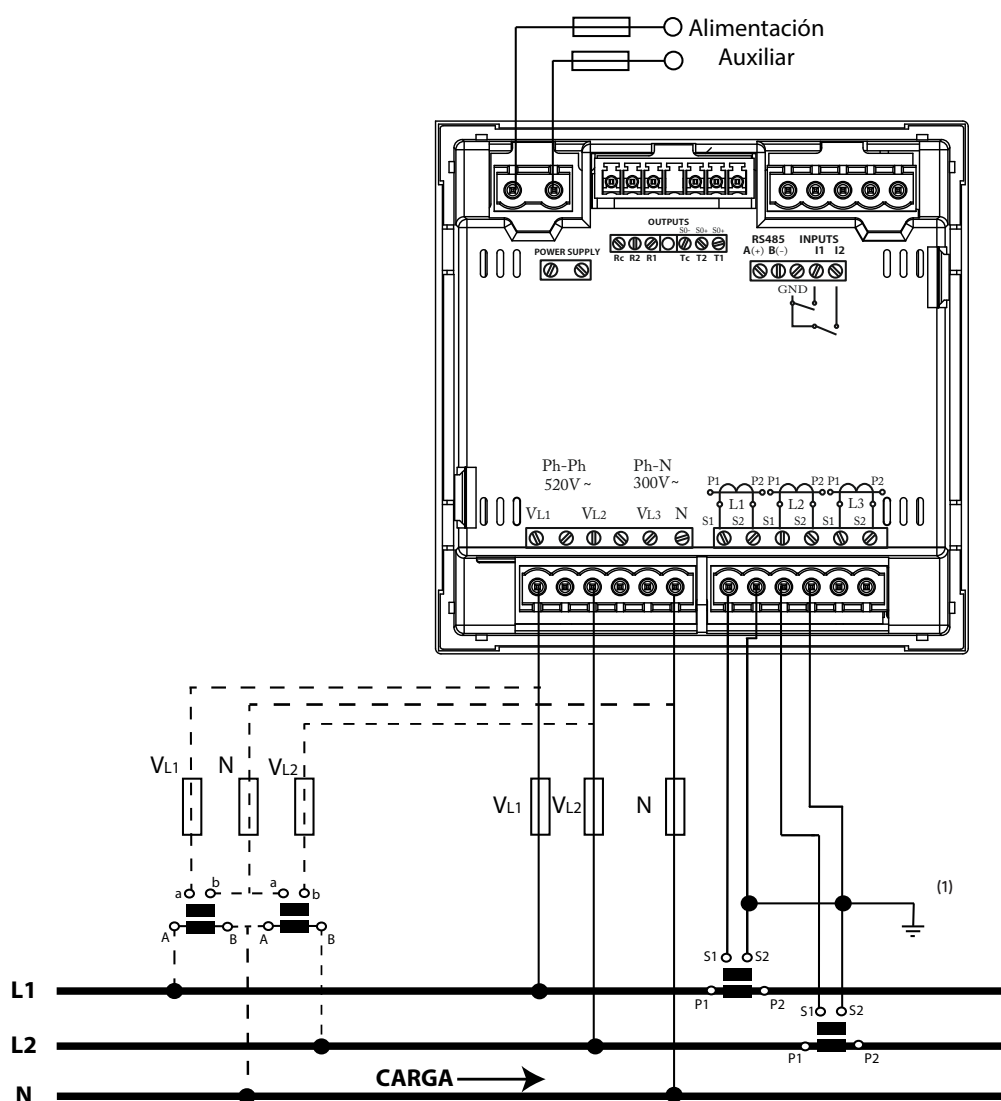
Figura 13: Medida bifásica con conexión a 3 hilos, modelos CVM-C10-ITF, CVM-C10-MC y CVM-C10-mV.
