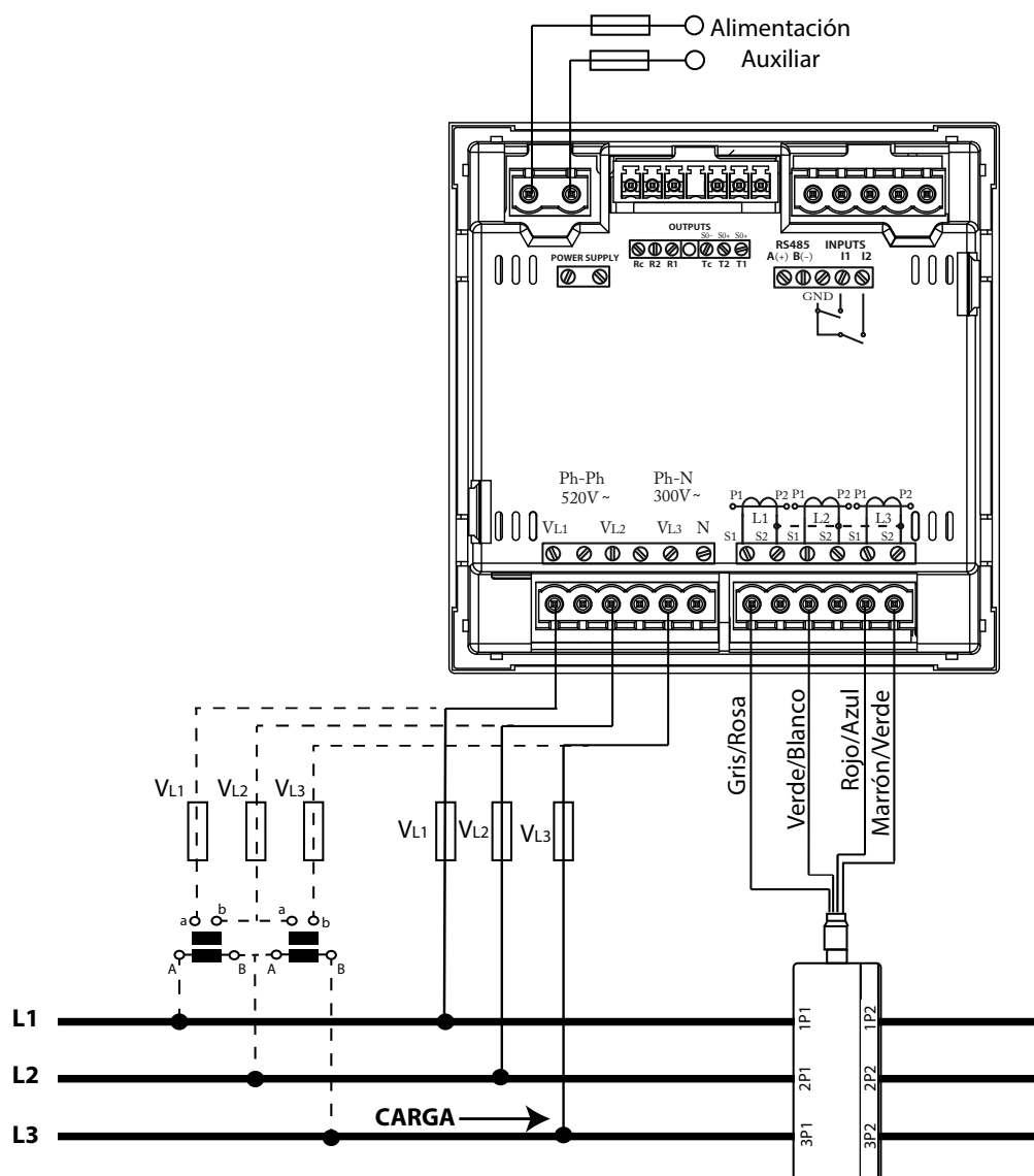
Figura 10: Medida trifásica con conexión a 3 hilos, modelo CVM-C10-MC.
