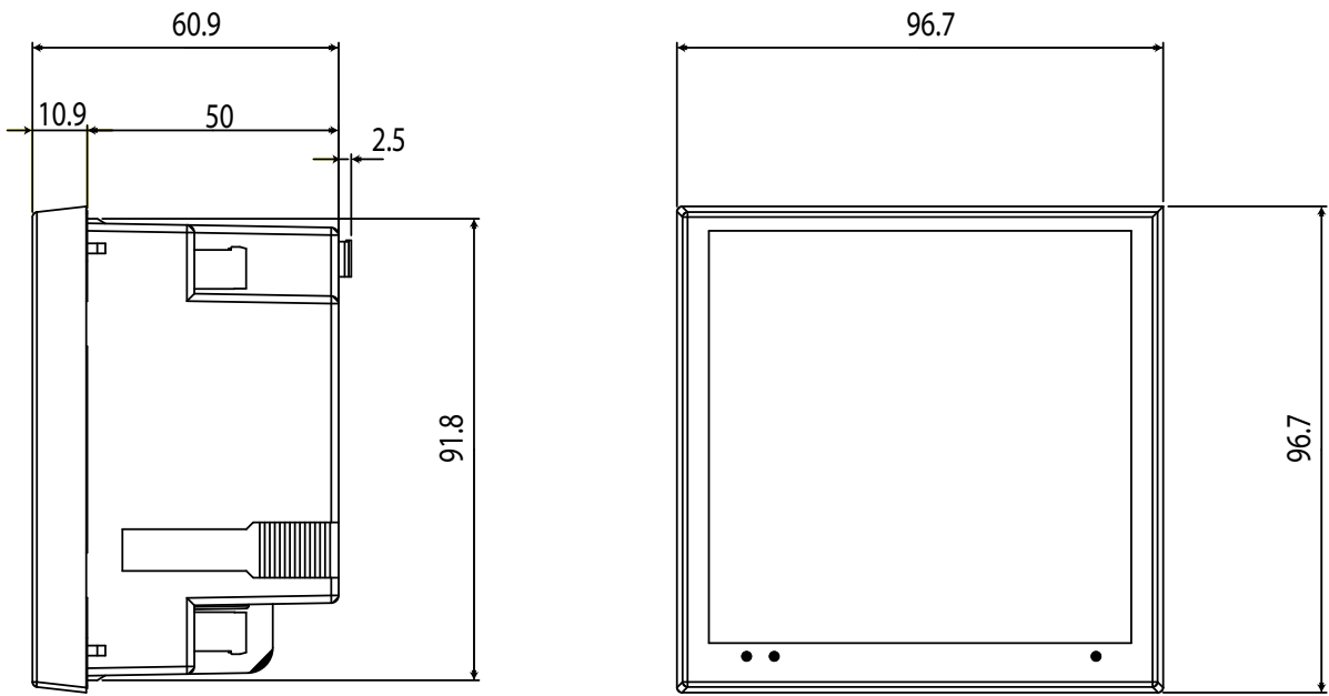
Figura 35: Dimensiones del CVM-C10.
