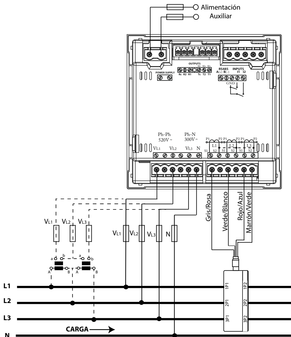
Figura 6: Medida trifásica con conexión a 4 hilos, modelo CVM-C10-MC.
