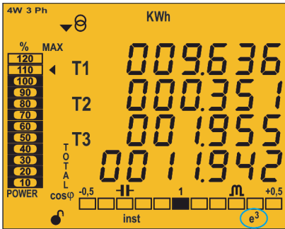
Figura 31: Pantalla del CVM-C10 con el perfil de funcionamiento e 3 .
