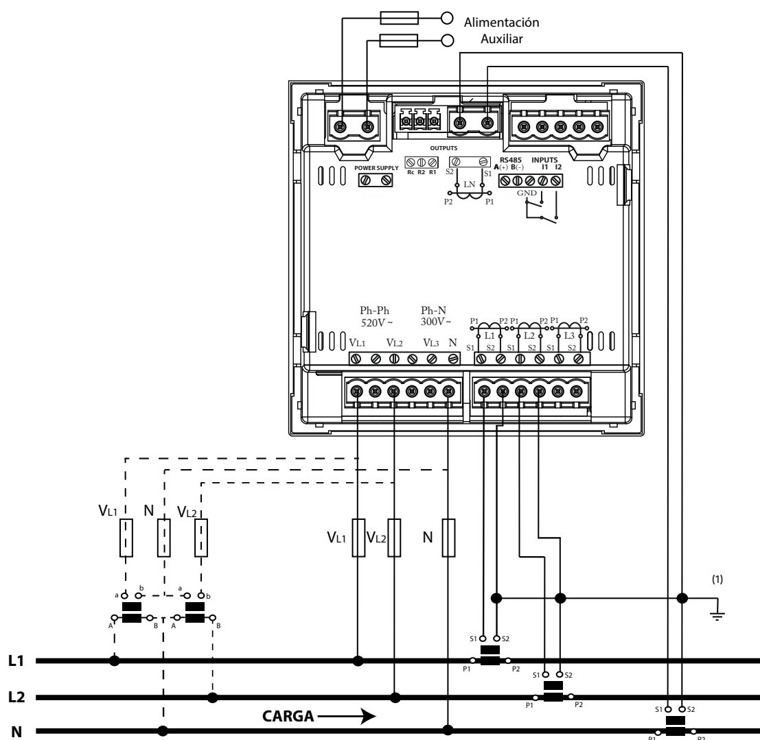
Figura 14: Medida bifásica con conexión a 3 hilos, modelos CVM-C10-ITF-IN y CVM-C10-MC-IN.
