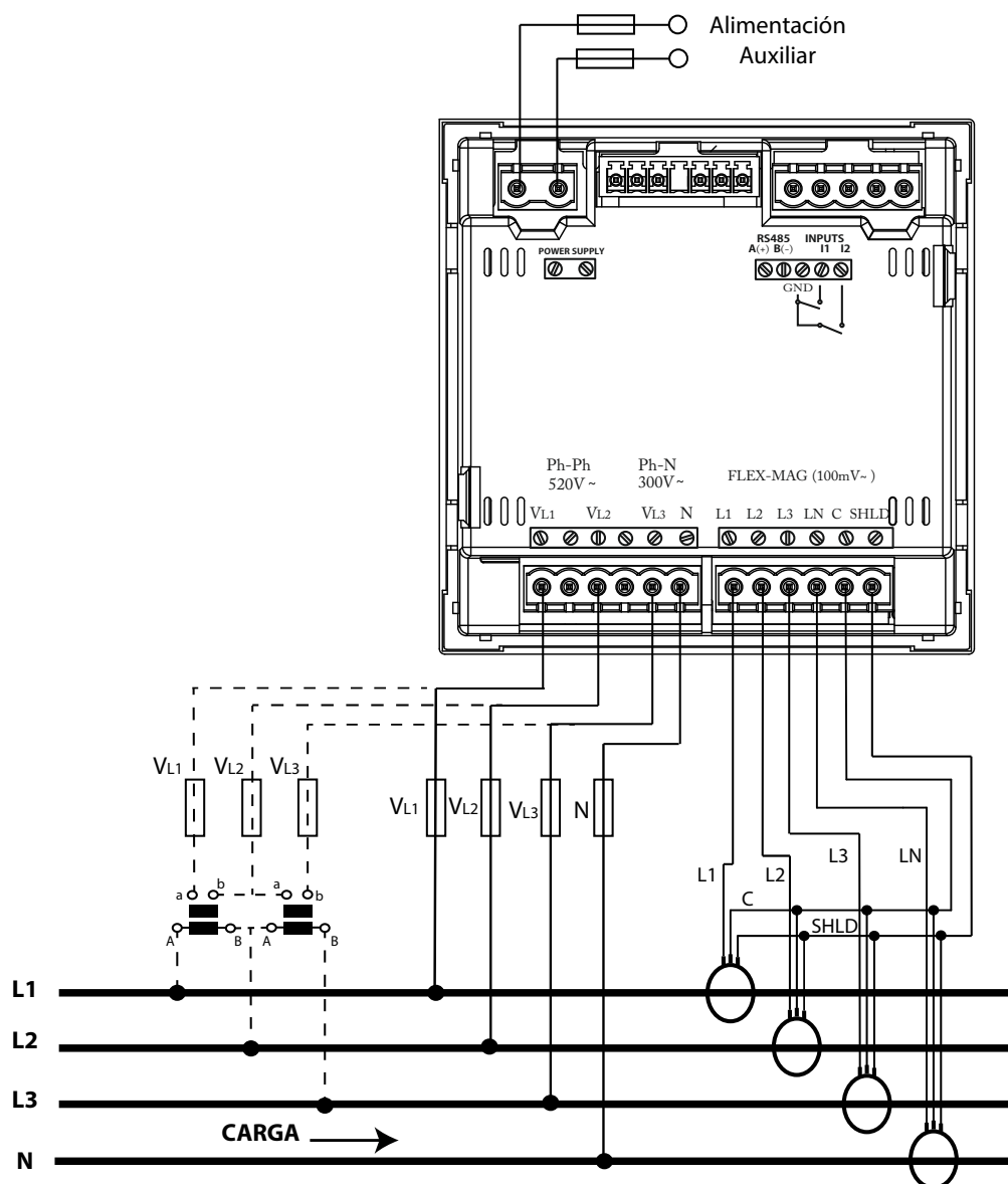
Figura 8: Medida trifásica con conexión a 4 hilos, modelo CVM-C10-FLEX.
