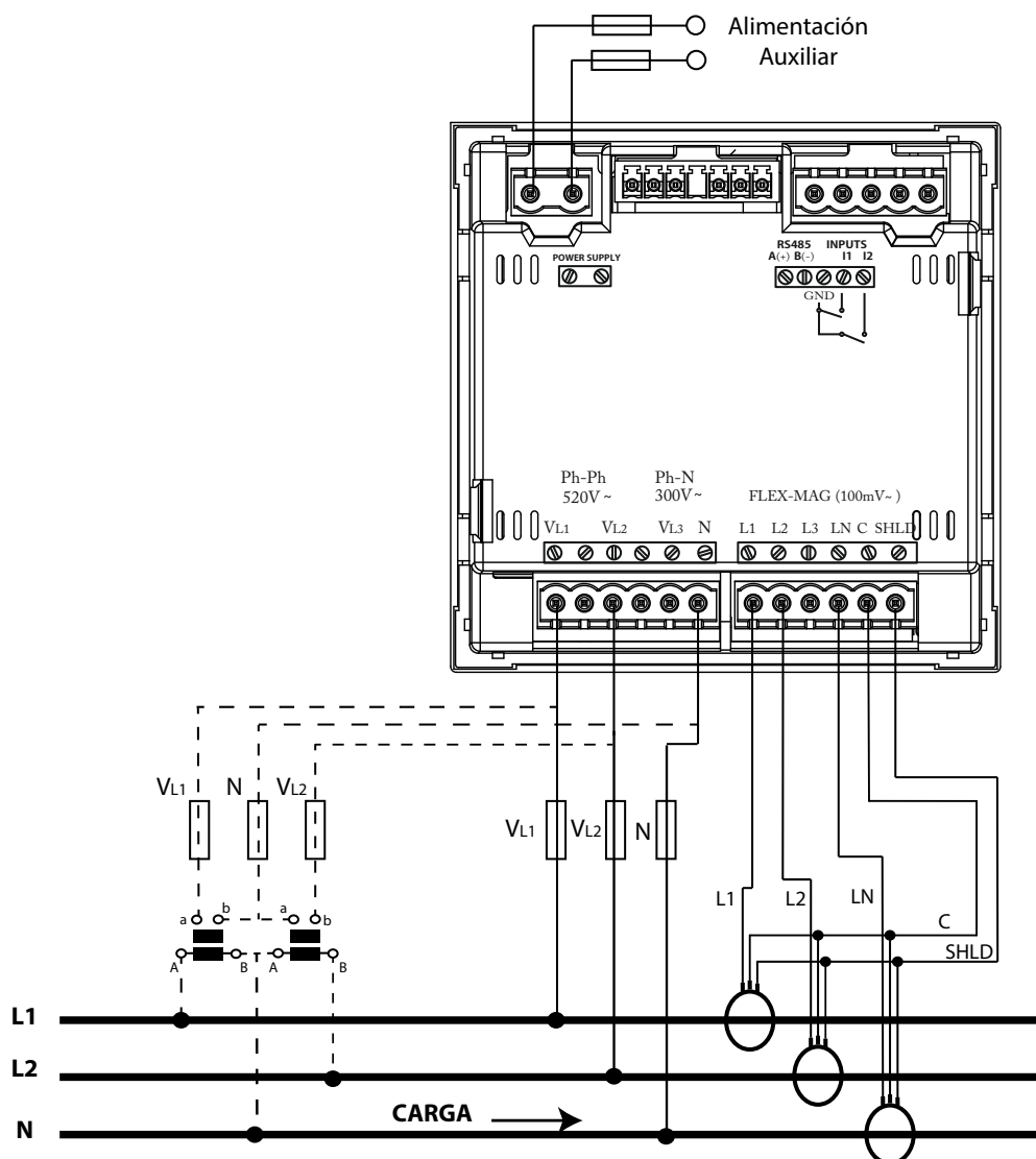
Figura 15: Medida bifásica con conexión a 3 hilos, modelo CVM-C10-FLEX.
