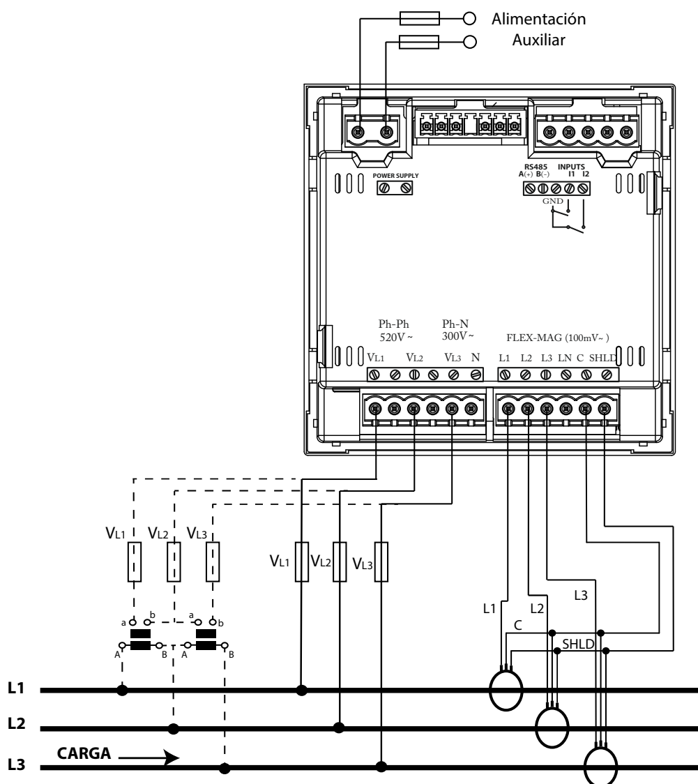
Figura 11: Medida trifásica con conexión a 3 hilos, modelo CVM-C10-FLEX.
