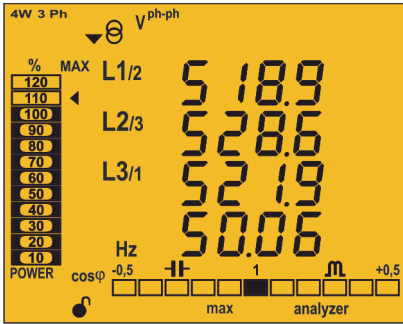
Figura 28: Pantalla del perfil analyzer visualizando los valores máximos.
