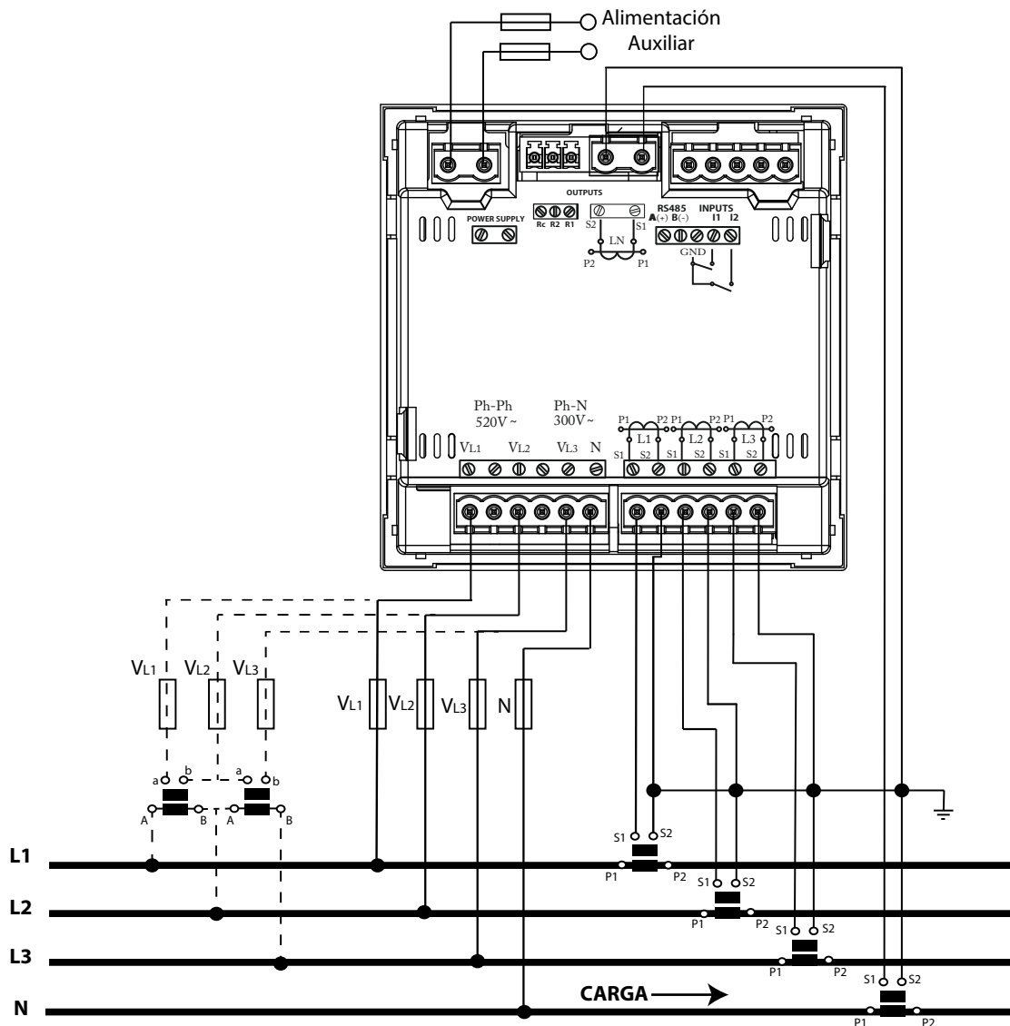
Figura 5: Medida trifásica con conexión a 4 hilos, modelo CVM-C10-ITF-IN.
