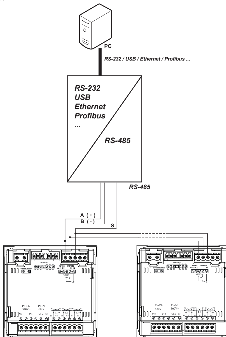
Figura 34: Esquema de conexionado RS-485.
