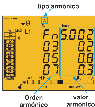
Figura 33: Pantalla de los armónicos de corriente del CVM-C10.
