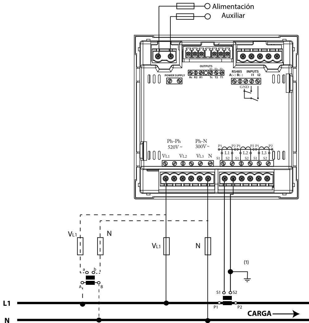
Figura 18: Medida monofásica de fase a neutro de 2 hilos, modelos CVM-C10-ITF, CVM-C10-MC y CVM-C10-mV.
