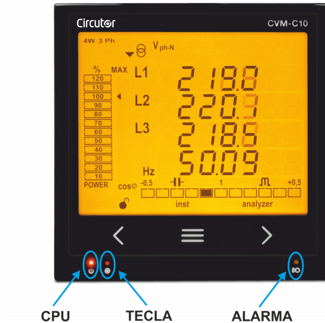
Figura 26: Indicadores LED del CVM-C10.
