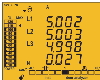
Figura 30: Pantalla del perfil analyzer visualizando los valores de máxima demanda.
