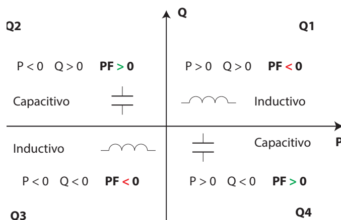
Figura 22: Convenio de medida IEEE.
