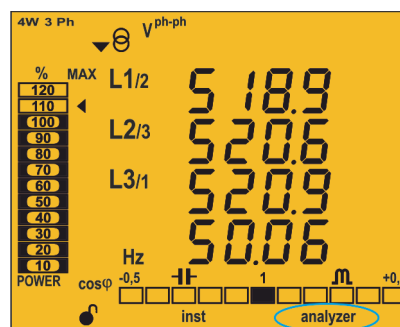
Figura 27: Pantalla del CVM-C10 con el perfil de funcionamiento analyzer.
