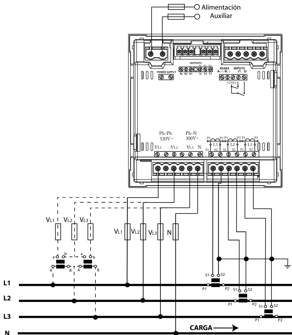
Figura 4: Medida trifásica con conexión a 4 hilos, modelos CVM-C10-ITF y CVM-C10-mV.
