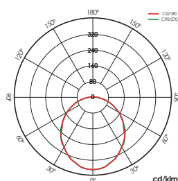
Lynx/Lynx difusor Lynx/Lynx diffuser Lynx/Lynx diffuseur Lynx/Lynx difusor
